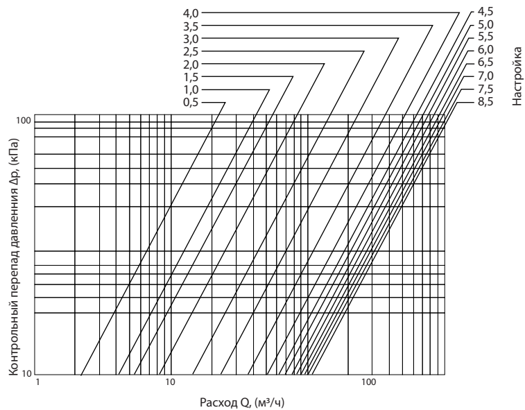
Пропускная способность, Kv («Гранбаланс» КБЧ серии 10, DN150)
