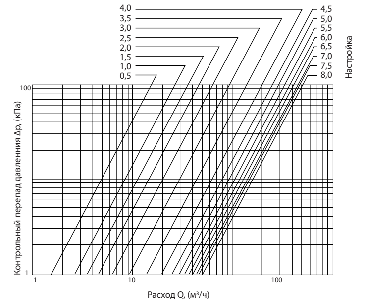
Пропускная способность, Kv («Гранбаланс» КБЧ серии 10, DN100)
