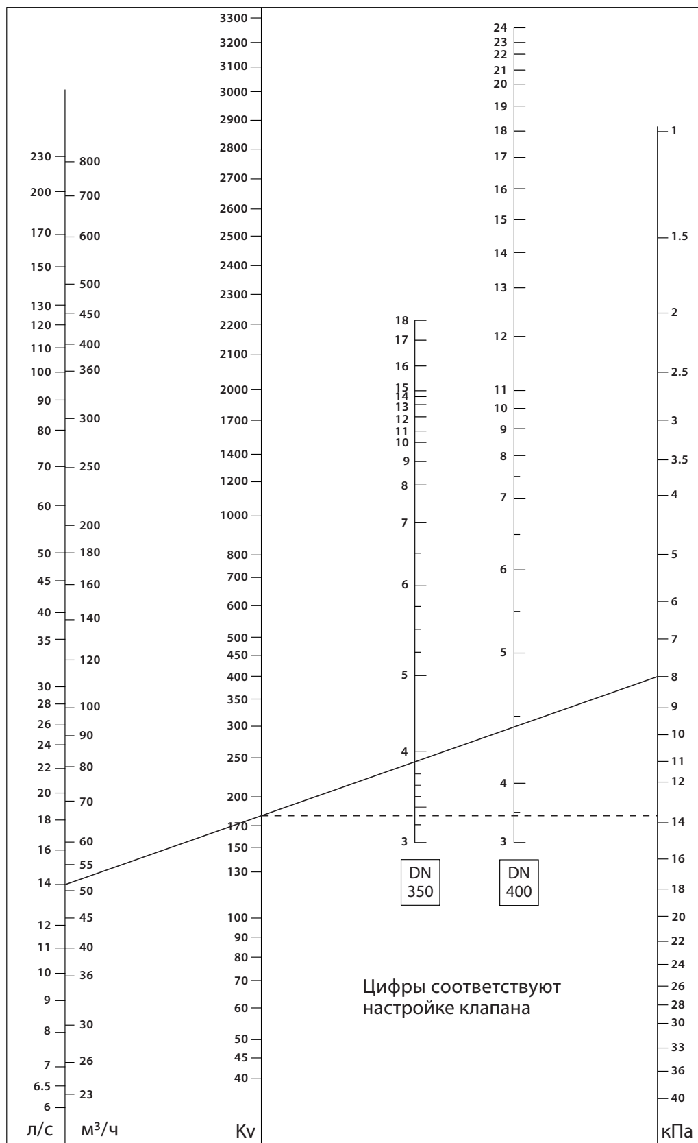
Диаграмма 3. Подбор типоразмера и предварительной настройки клапана (DN350–400)
