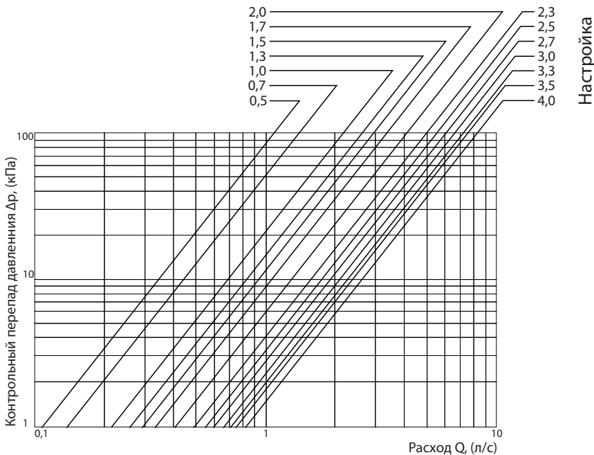
Пропускная способность, Kv (VIR 9505K, DN50)
