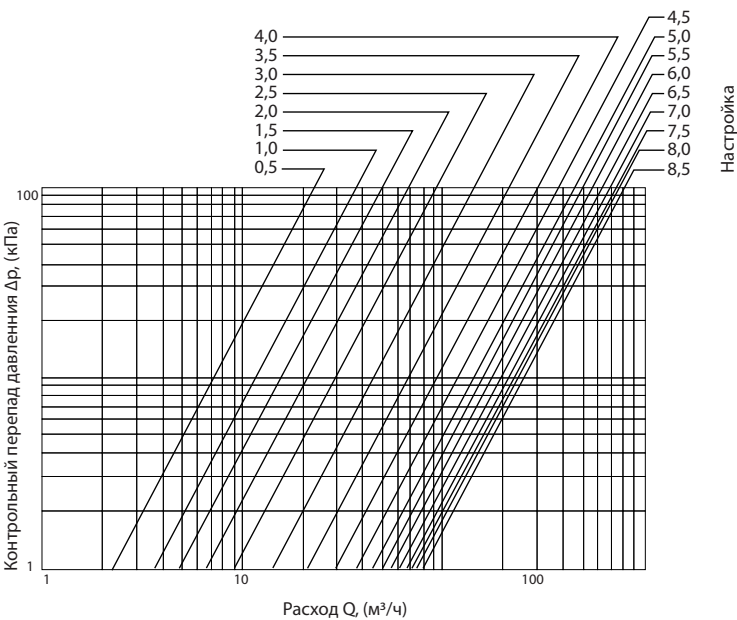
Пропускная способность, Kv («Гранбаланс» КБЧ серии 10, DN125)
