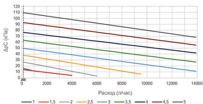
Диаграмма подбора настроечной позиции картриджа регулятора давления DN40–50 мм
