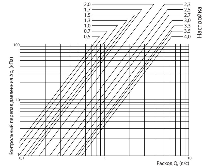
Пропускная способность, Kv (VIR 9505K, DN40)
