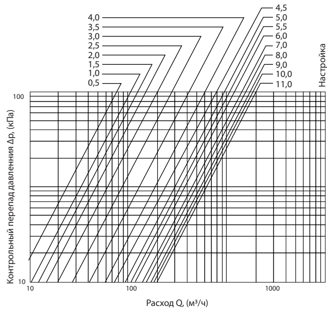
Пропускная способность, Kv («Гранбаланс» КБЧ серии 10, DN200)
