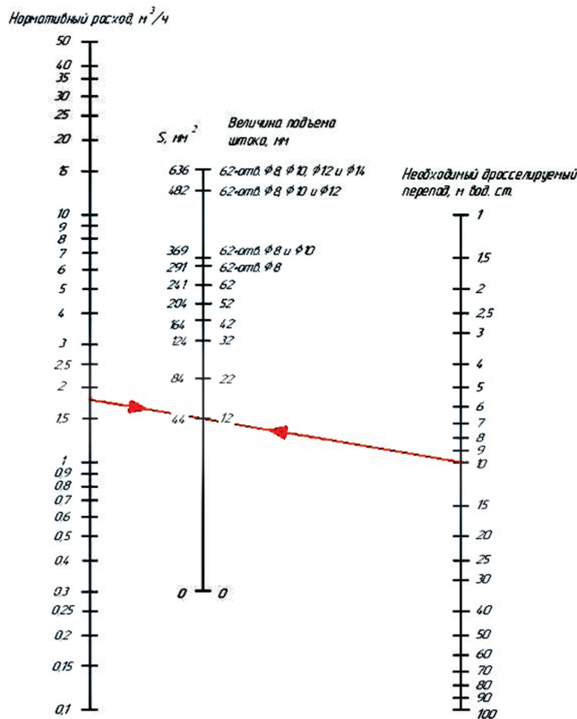
Номограмма настройки регулируемой дроссельной шайбы Ду 100 мм
