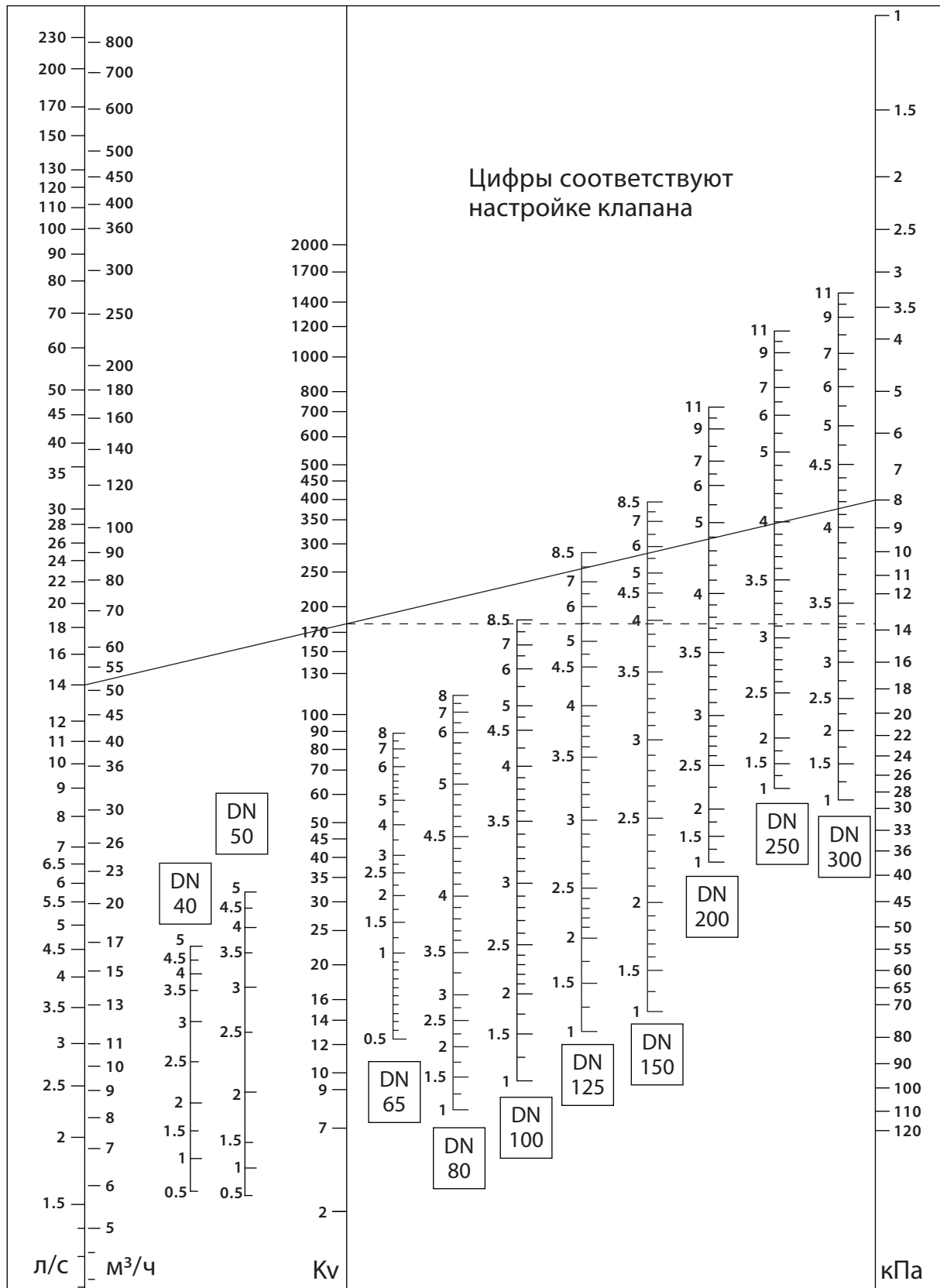
Диаграмма 3. Подбор типоразмера и предварительной настройки клапана (DN40–300)
