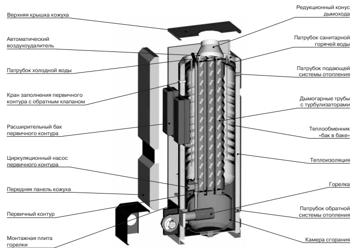
Устройство котла Heat Master 70 N / 100 N
