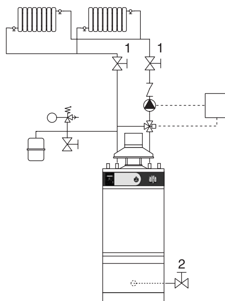
Рис. 12a: Слив контура отопления
