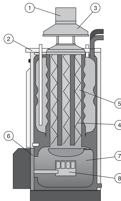
Рис. 11: Устройство котла
