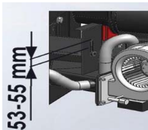
Положение направляющей воздушной заслонки системы безопасности
