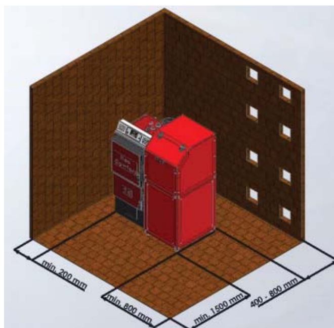
Расположение котла ECO COMFORT
