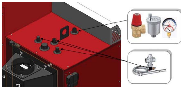
Расположение предохранительных устройств
