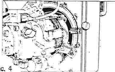
Рис. 4 Первичный воздух (см. таблицу)
