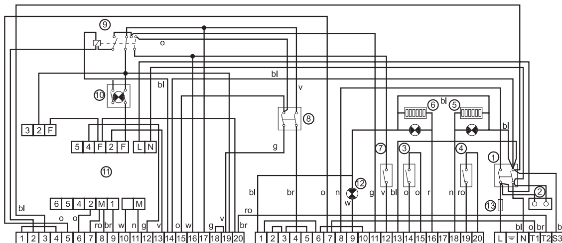
Рис. 2: Электрическая схема
