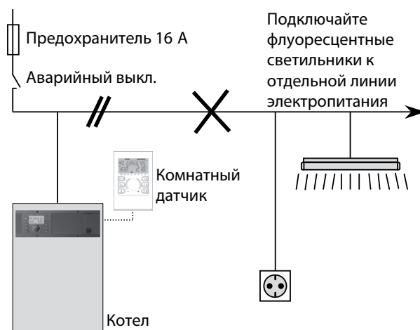
Рис. 3: Линии электропитания в котельной
