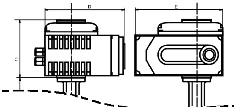
Чертеж габаритный полнопроходного шарового крана ABRA-BV с электроприводом Сатурн, DN 15-DN150
