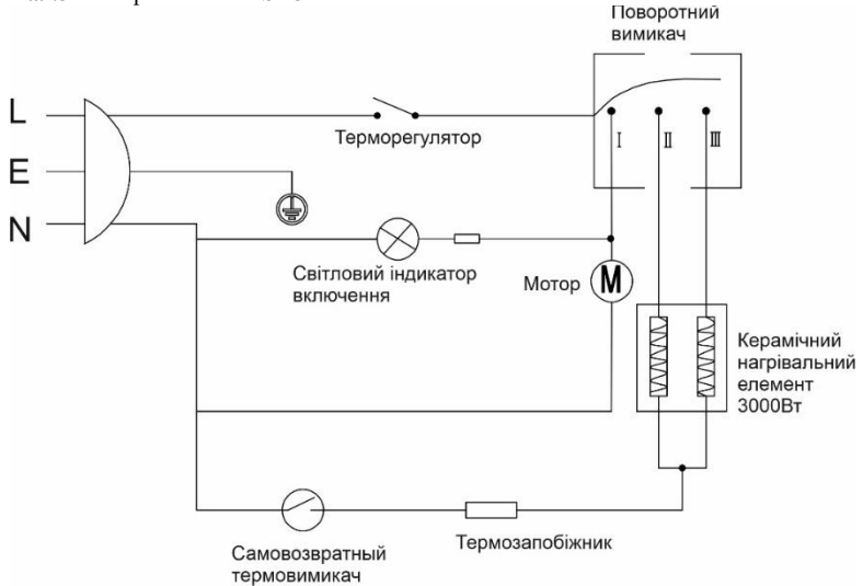
Мал.4 Електрична схема STORM 3
