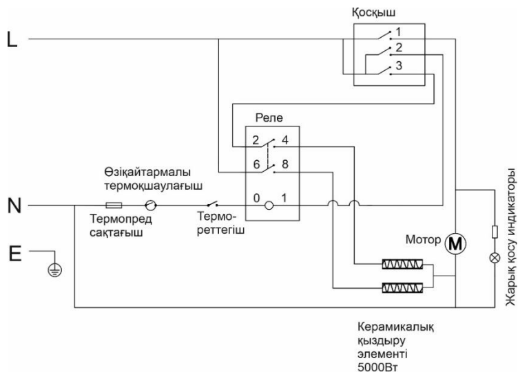
5-сұр. Электр схемасы STORM 5
