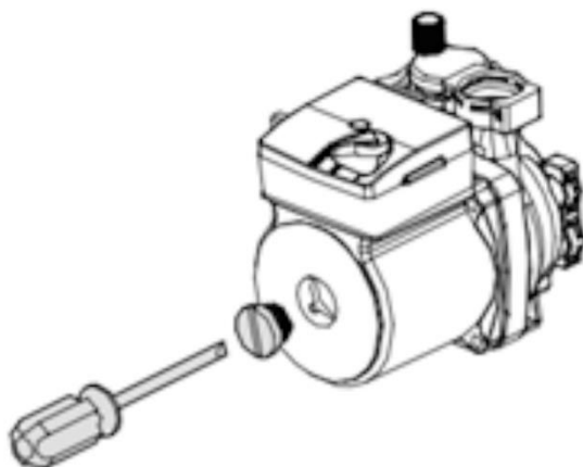
Рис.15. Проверка насоса
