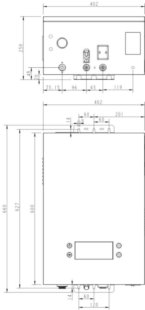
Рис.2. Габаритные размеры
