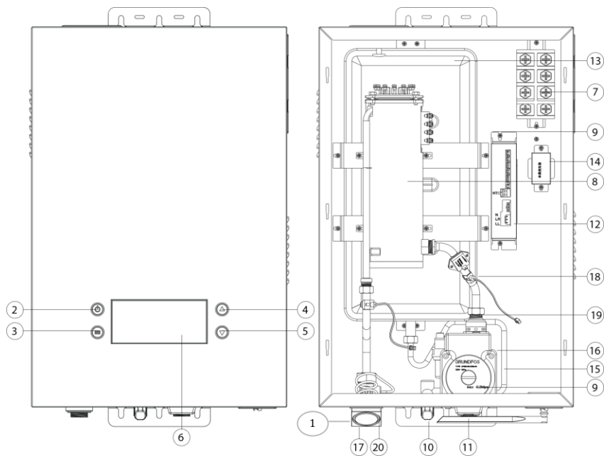
Рис. 1. Конструкция изделия
