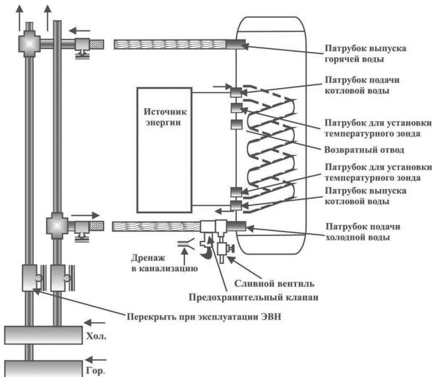
Рисунок 1. Схема подключения.
