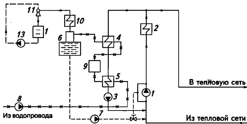
Рис. 6.6. Принципиальная тепловая схема районной-квартирной тепловой станции (РТС или КТС) с водогрейными котлами
