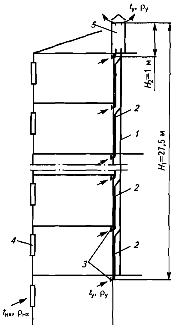
Рис. 2.4. Схема естественной канальной вытяжной вентиляции из кухонь квартир многоэтажного жилого дома
