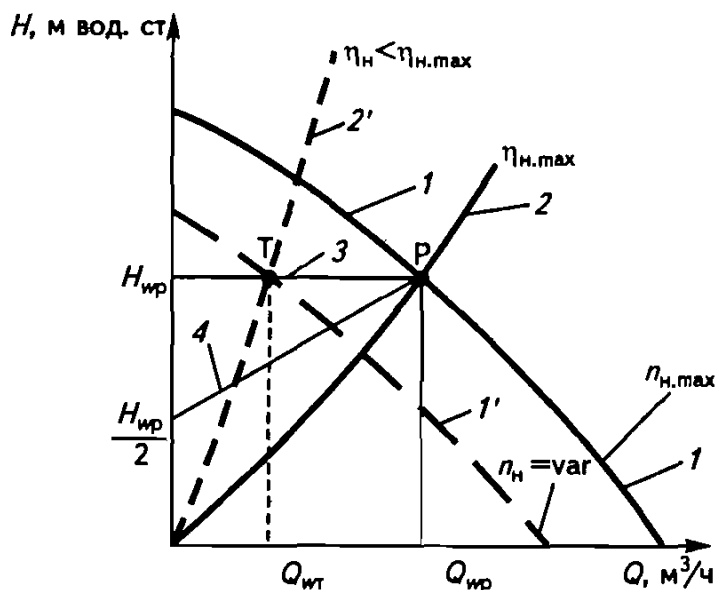
Рис. 3.14. Рабочие характеристики насоса при переменной частоте вращения рабочего колеса \eta_n = \text{var} по команде датчика, контролирующего постоянство развиваемого насосом напора H_{\text{вр}} или пропорциональное изменение напора H_{\text{вр.пр}} . 1 и 1' – характеристики насоса при различном числе оборотов рабочего колеса; 2 и 2' – характеристики гидравлической сети при количественном регулировании расхода горячей воды от Q_{\text{вр}} до Q_{\text{нт}} ; 3 – настройка работы насоса на поддержание постоянного напора в сети H_{\text{вр}} ; 4 – настройка работы насоса на пропорциональное изменение напора в сети от H_{\text{вр}} до H_{\text{вр}} / 2
