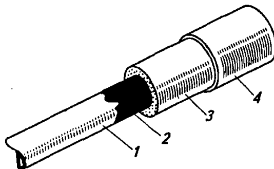
Рис. 6.29. Теплоизоляционная конструкция с битумоперлитной изоляцией 1 – труба; 2 – антикоррозионное покрытие; 3 – битумоперлит; 4 – гидрозащитное покрытие из стеклоткани по лаку
