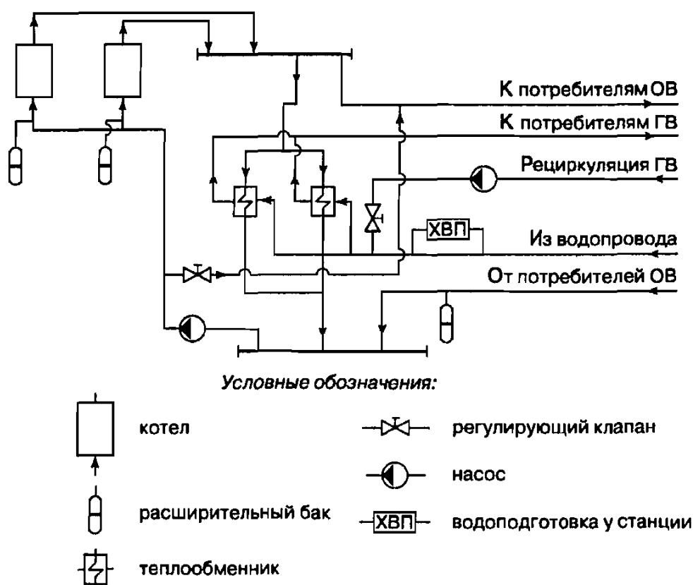
Рис. 6.8. Принципиальная тепловая схема крышной газифицированной котельной
