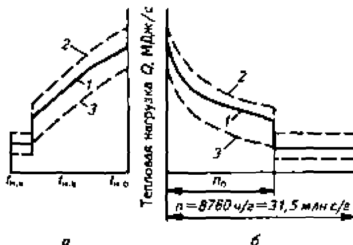
Рис. 10.5. Построение графика продолжительности сезонной тепловой нагрузки
