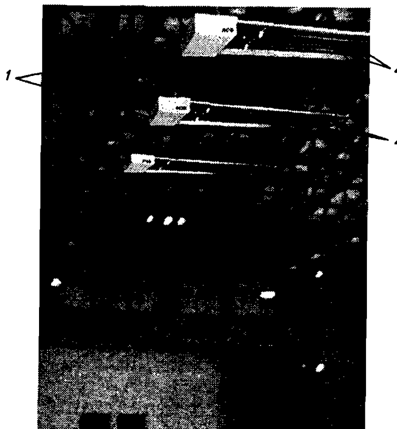
Рис. 5.5. Внешний вид нагревателя лучистого типа НЛТ фирмы «Промгаз» (а) и монтажная подвеска трех агрегатов НЛТ к металлическим конструкциям перекрытия цеха (б)
