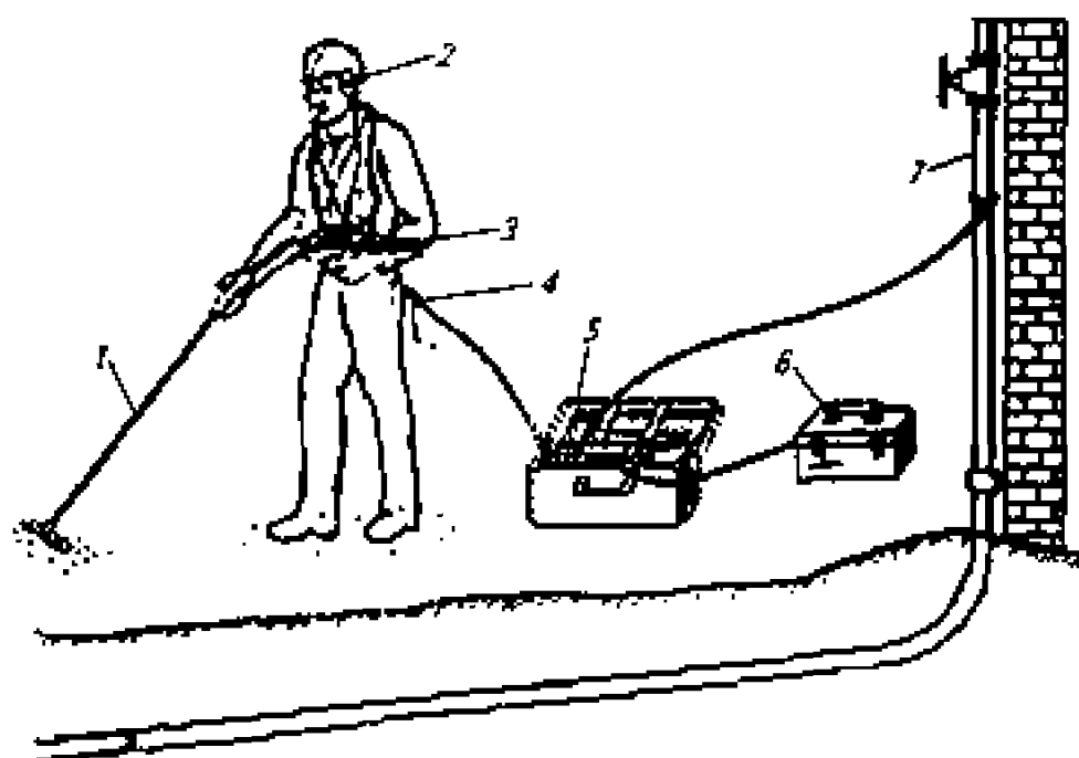
Рис. 10.13. Определение места утечки воды с помощью трассоискателя 1 – трассоискатель; 2 – наушники; 3 – измерительный прибор; 4 – заземлитель; 5 – генератор; 6 – аккумулятор; 7 – подзаемный трубопровод
