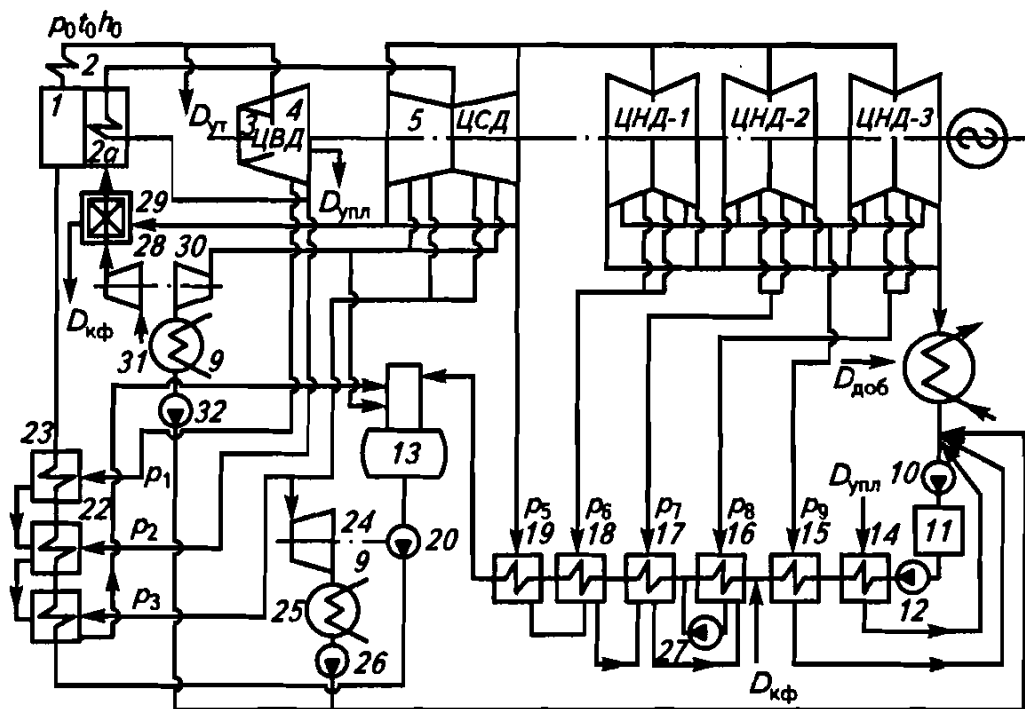
Рис. 6.5. Тепловая схема конденсационной электрической станции (КЭС)
