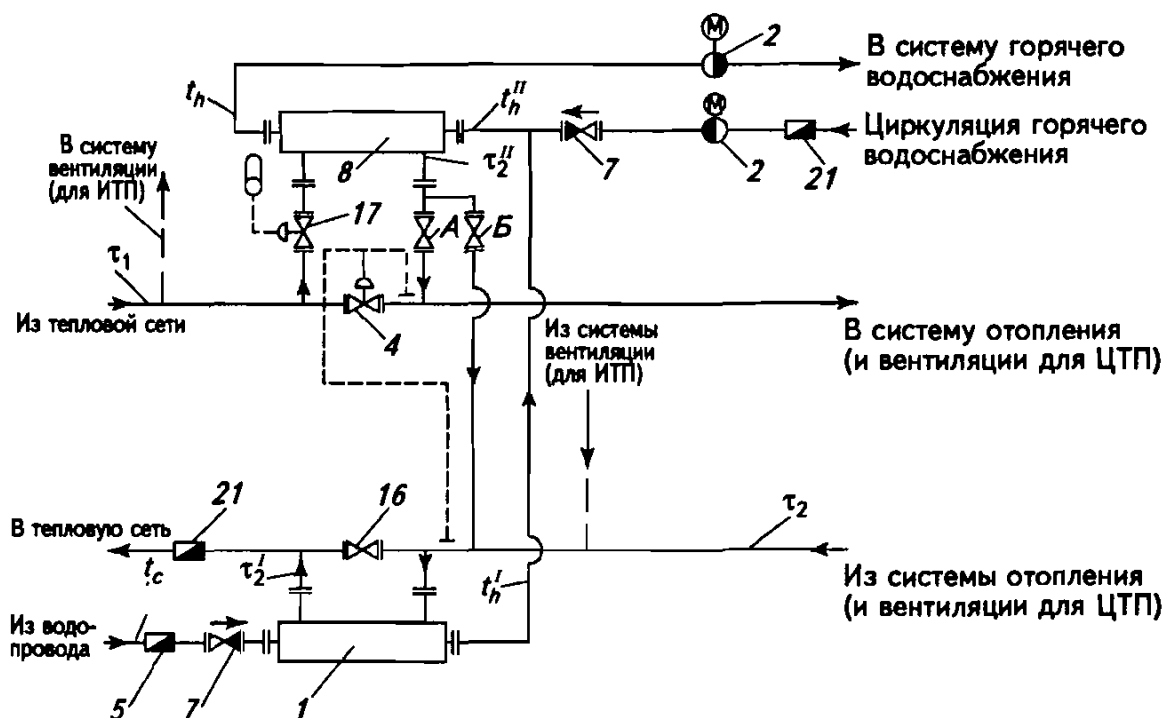
Рис. 6.36. Двухступенчатая последовательная схема присоединения ВВП ГВС с зависимым присоединением систем отопления при отсутствии регуляторов расхода теплоты на отопление в ЦТП и ИТП в закрытых СЦТ 1–21 – см. рис. 6.35
