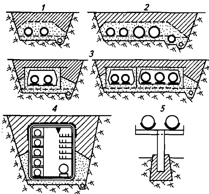
Рис. 6.15. Современные способы прокладки тепловых сетей
