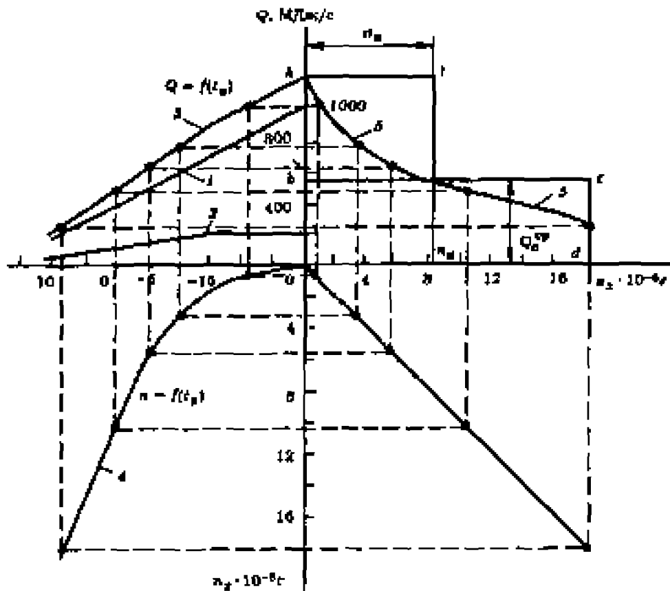
Рис. 10.5. Построение графика продолжительности сезонной тепловой нагрузки
