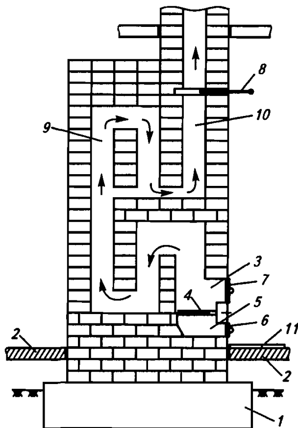
Рис. 3.1. Конструкция комнатной отопительной печи
