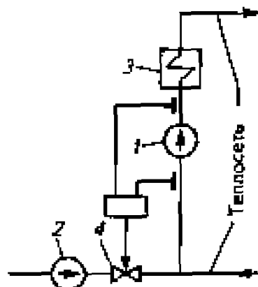
Рис. 10.11. Принципиальная схема автоматизации подпитки тепловой сети на теплоисточнике
