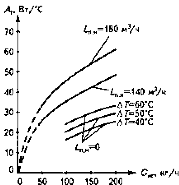
Рис. 7.19. Опытная зависимость удельной тепловой производительности теплообменника в доводчике ДЭ 2.6.140/180
