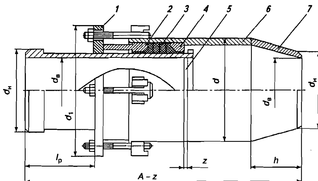
Рис. 6.24. Односторонний сварной сальниковый компенсатор 1 – нажимной фланец; 2 – грундбукса; 3 – сальниковая набивка; 4 – контрбукса; 5 – стакан; 6 – корпус; 7 – переход диаметров. Компенсирующая способность его составляет 250–400 мм
