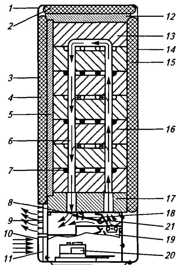
Рис. 1.3. Принципиальная схема местного электроотопительного агрегата с теплоаккумулирующей насадкой
