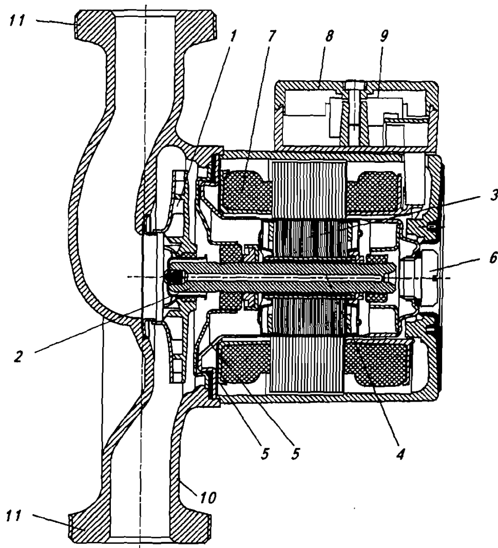
Рис. 4.2. Конструктивная схема бессальниковых насосов UPS для систем отопления
