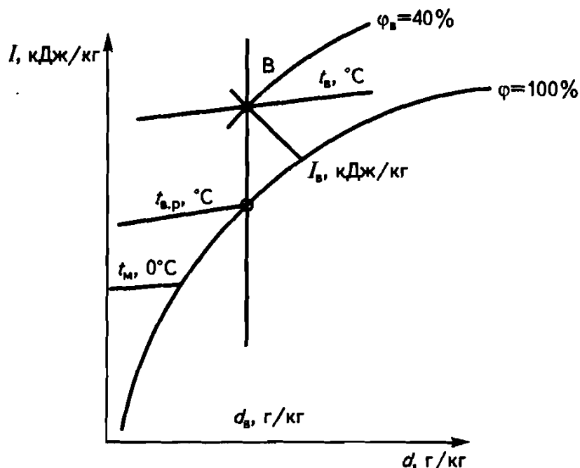
Рис. 2.7. Нахождение на I - d -диаграмме параметров влажного воздуха t_b – температура, °C; d_b – влагосодержание, г/кг; \varphi_b – степень насыщения воздуха водяными парами, %; \varphi = 100\% – полностью насыщенный водяными парами воздух; I_b – энтальпия воздуха, кДж/кг; t_{a.p.} – температура точки росы влажного воздуха, °C; t_m = 0^\circ\text{C} – температура строительного материала при 0^\circ\text{C} , когда замерзает вода
