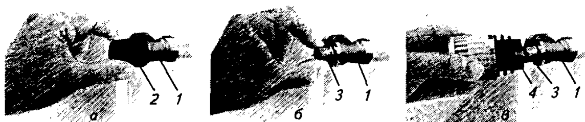
Рис. 4.18. Наладочное регулирование гидравлического сопротивления циркуляционных колец системы отопления с помощью терморегуляторов типа RTD а – монтаж при наличии защитного колпачка; б – подъем и поворот настроечного кольца; в – установка термостатической головки; 1 – корпус клапана; 2 – защитный пластмассовый колпачек; 3 – настроечное кольцо клапана; 4 – термостатическая головка
