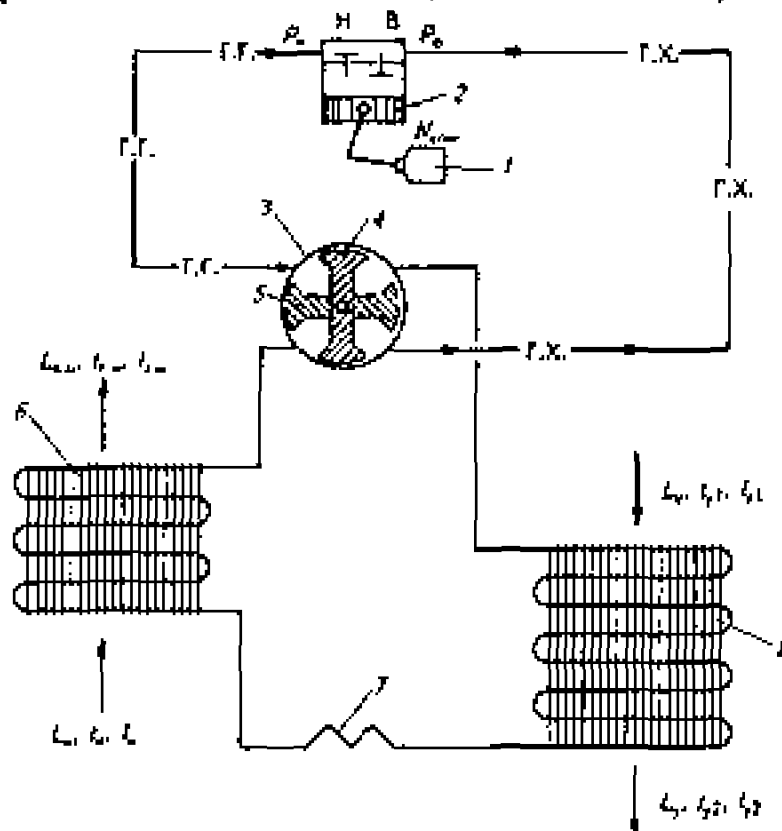
Рис. 8.3. Принципиальная схема парокомпрессионной холодильной машины с воздушным конденсатором и испарителем
