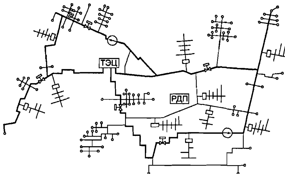
Рис. 6.14. Схема изолированной тепловой сети от одной ТЭЦ с насосно-повысительными подстанциями, гидравлическими регуляторами и перемычками РДП – районный диспетчерский пункт; ———— – магистральные тепловые сети; ———— – распределительные (квартальные) тепловые сети; □ – ЦТП; ○ – ИТП; ⊗ – насосные подстанции
