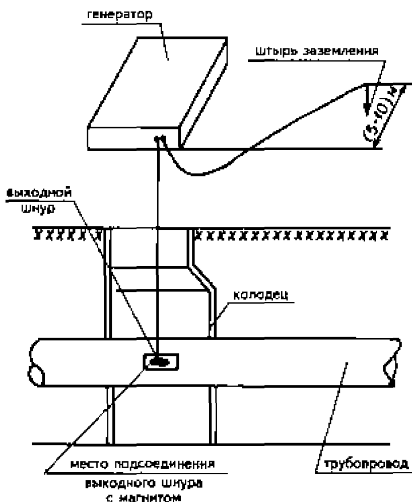
Рис. 10.17. Схема подключения генератора к коммуникации
