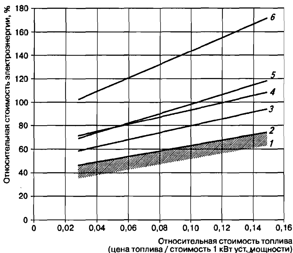
Рис. 6.11. Относительная стоимость электроэнергии для различных энергоустановок при различной стоимости топлива
