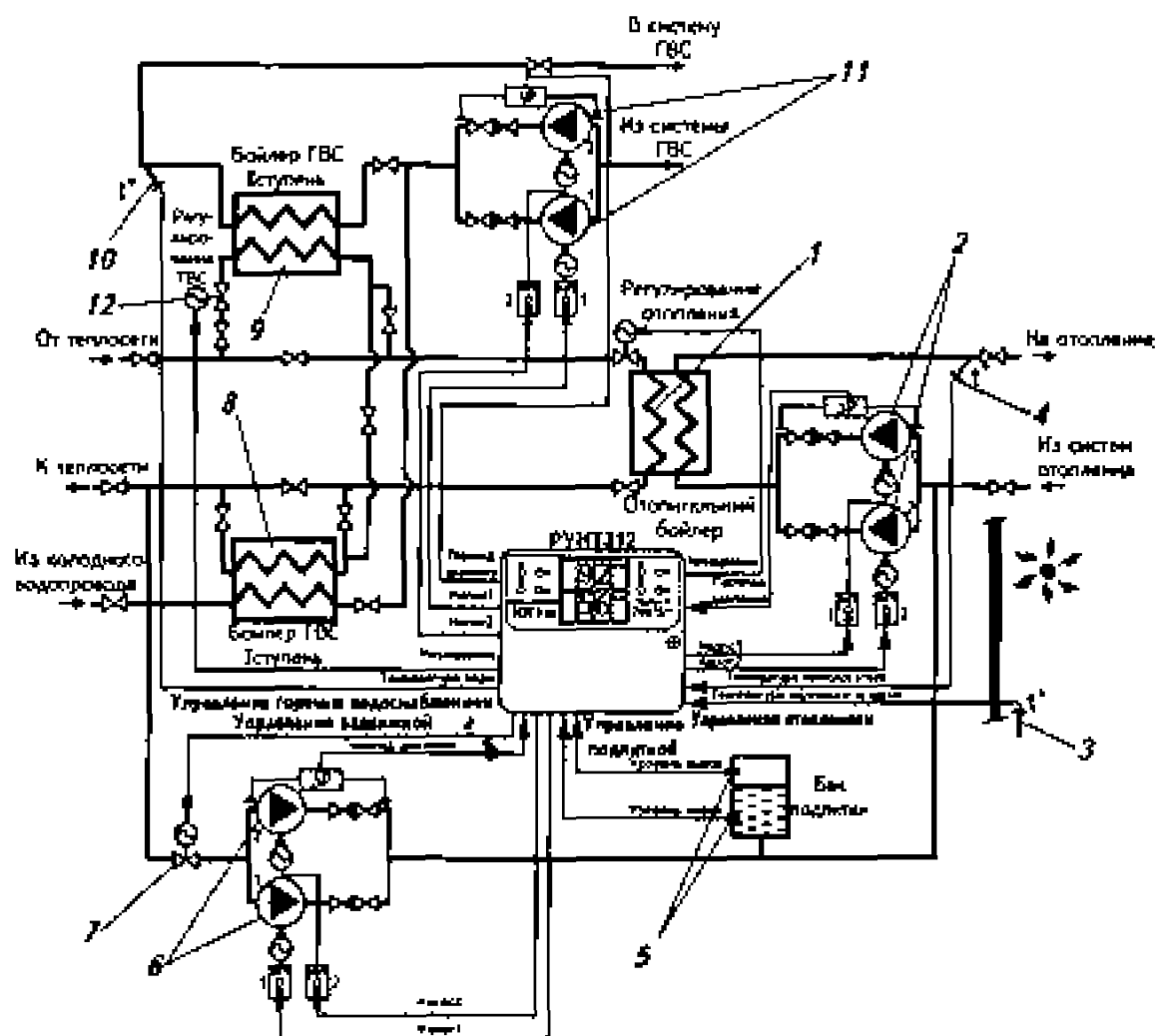
Рис. 7.1. Принципиальная схема применения автоматического регулятора РУНТ 312 в ЦТП для теплоснабжения систем отопления и горячего водоснабжения зданий
