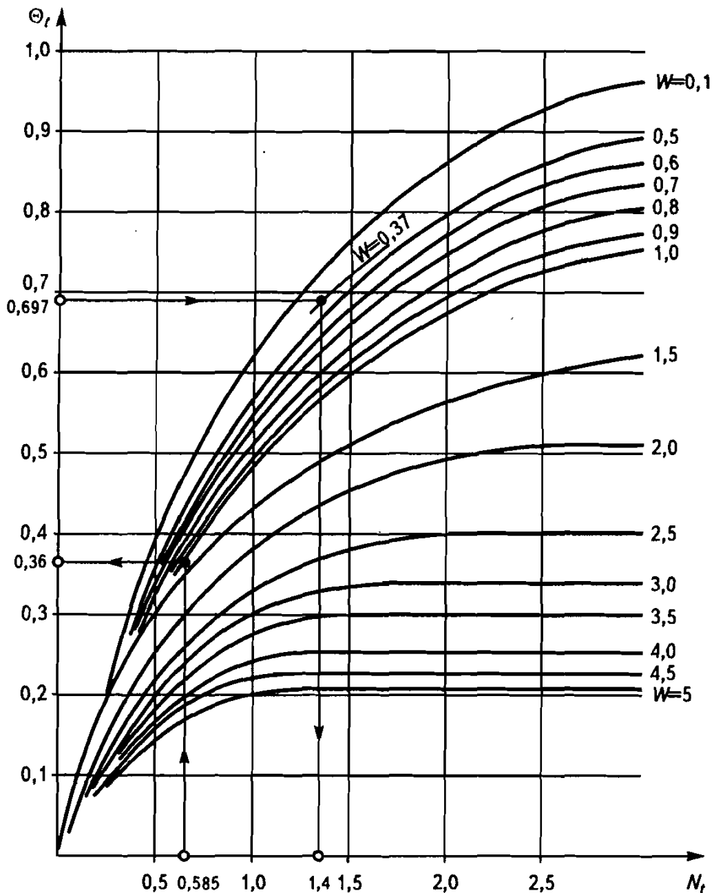
Рис. 3.7. Графическая зависимость показателя теплотехнической эффективности \Theta_r для противоточной схемы движения теплообменивающихся сред
