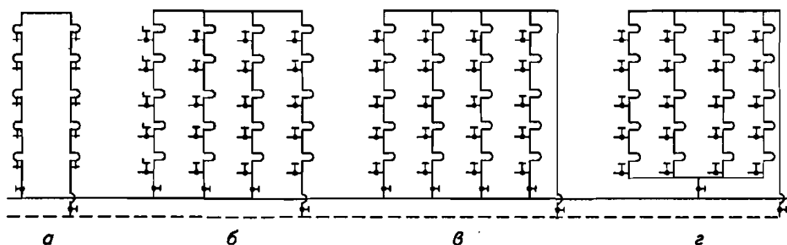
Рис. 6.39. Схемы присоединения водоразборных и циркуляционных стояков а – парнозакольцованный стояк; б – секционный узел с циркуляционно-водоразборным стояком; в, г – секционный узел с циркуляционным стояком
