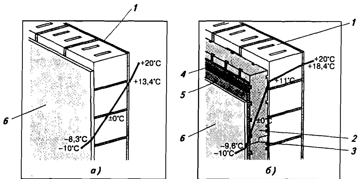
Рис. 2.2. Теплоизоляция наружных стен существующих зданий
