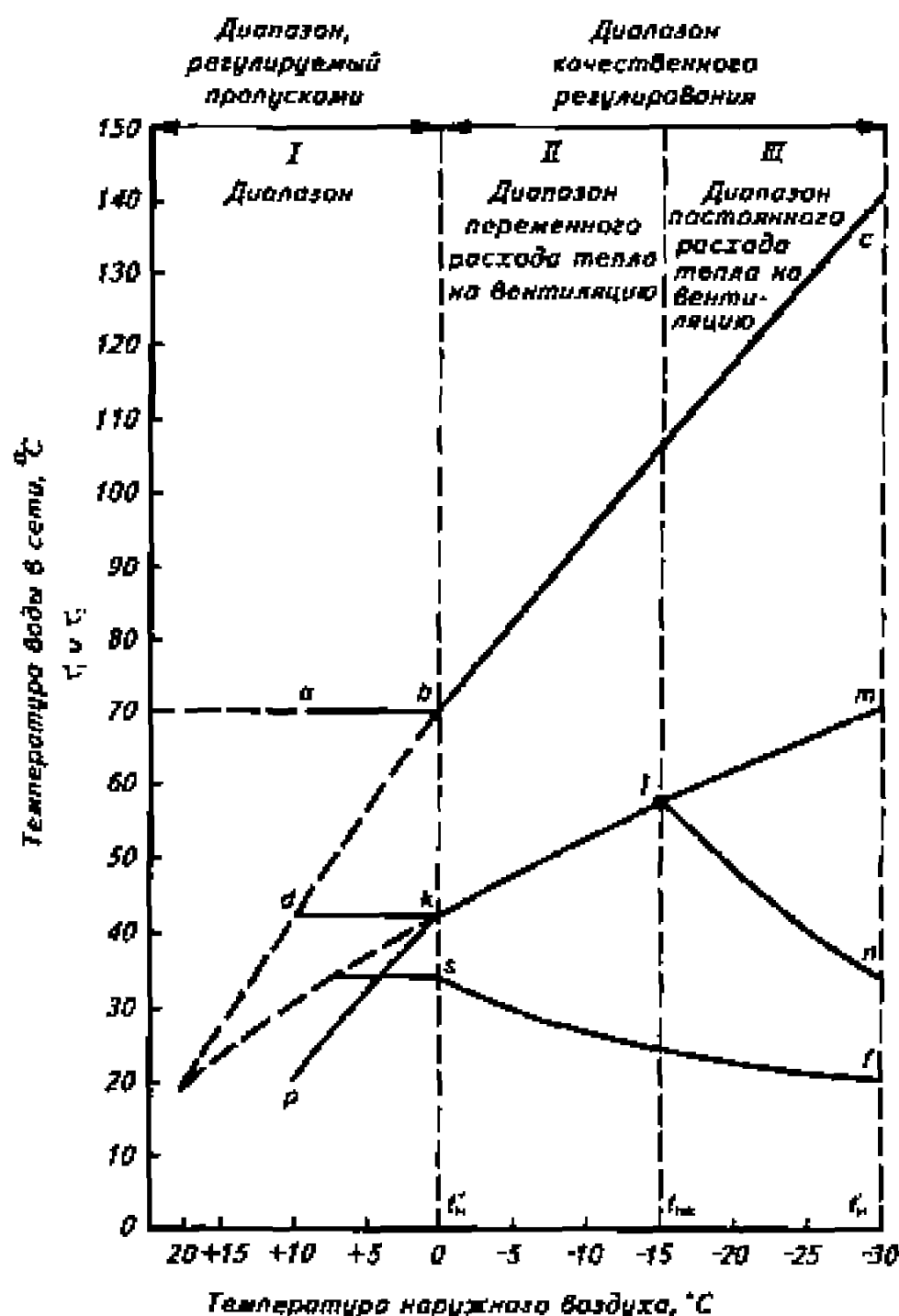
Рис. 10.8. График температуры воды в магистральных линиях теплосети при комбинированном регулировании
