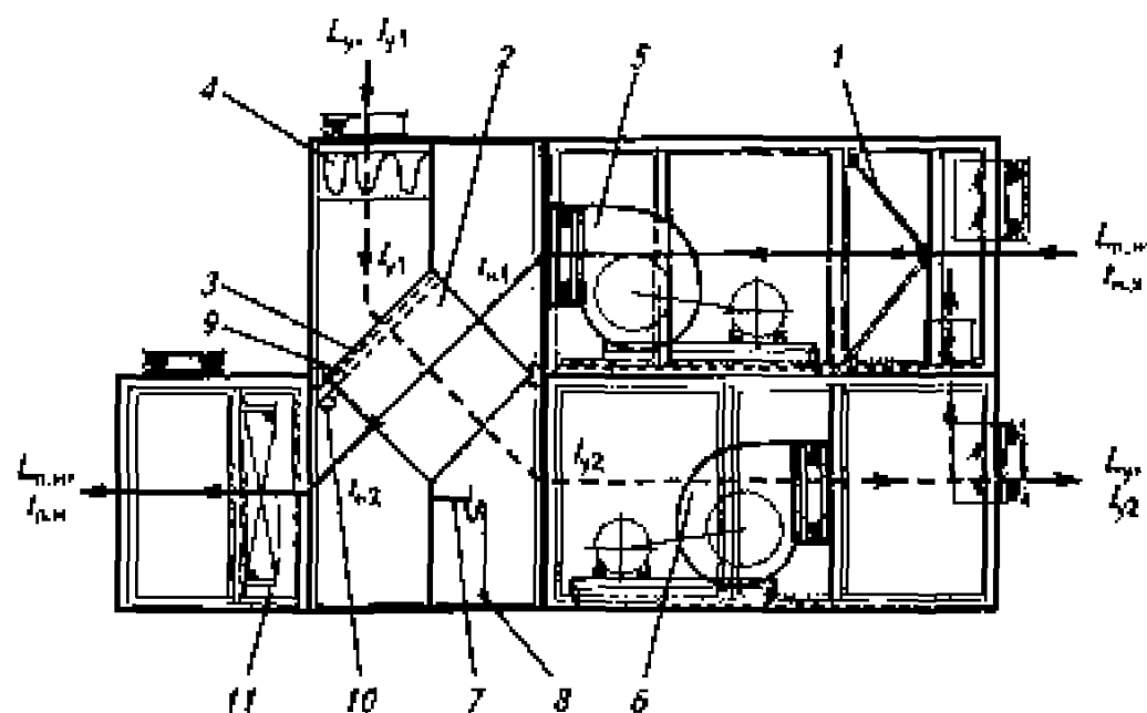
Рис. 9.8. Конструктивная схема приточного и вытяжного агрегатов с пластинчатым утилизатором, имеющим обводной воздушный канал по приточному наружному воздуху
