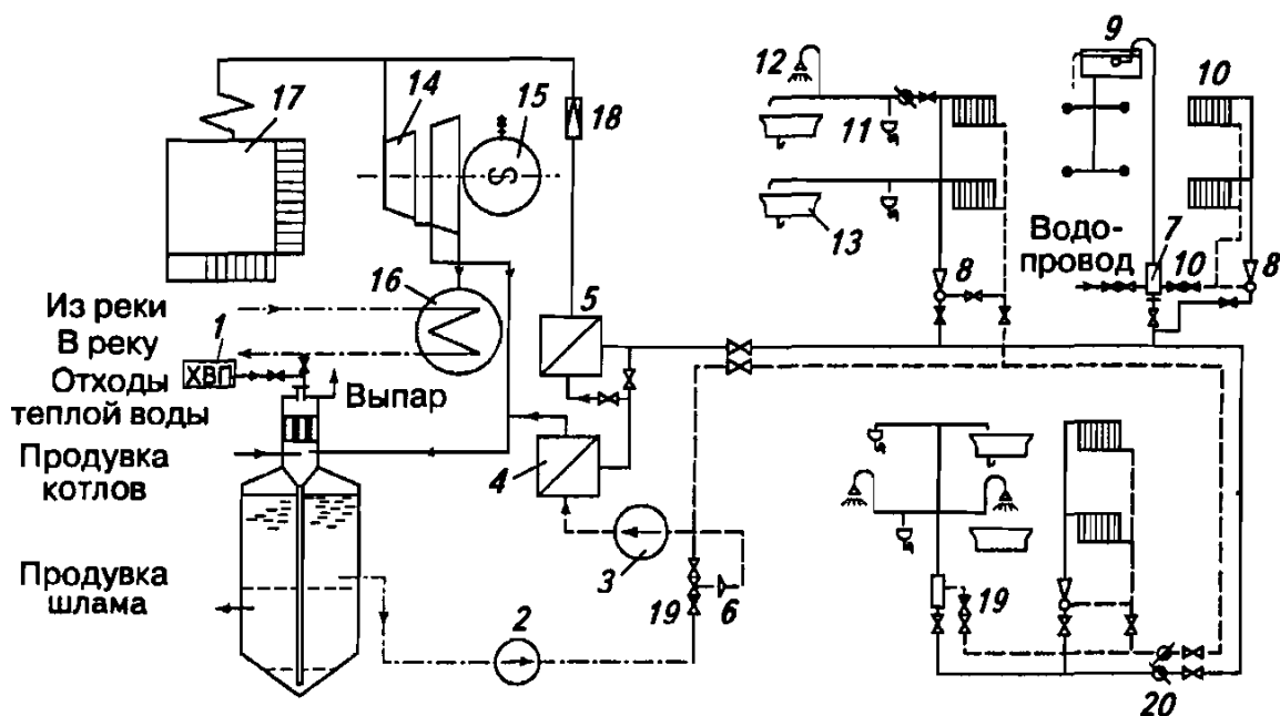
Рис. 6.9. Принципиальная схема ТЭЦ с непосредственным водоразбором из тепловых сетей с термической стабилизацией подпиточной воды для тепловых сетей [27]
