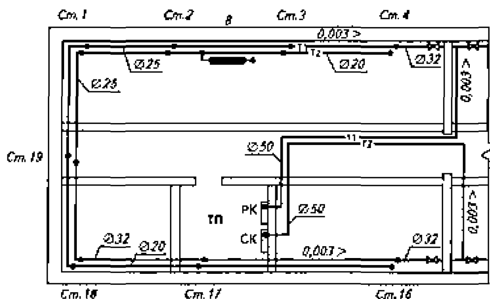
Рис. 9.5. Система с нижней разводкой с размещением распределительных и сборных магистральных трубопроводов в подвале здания
