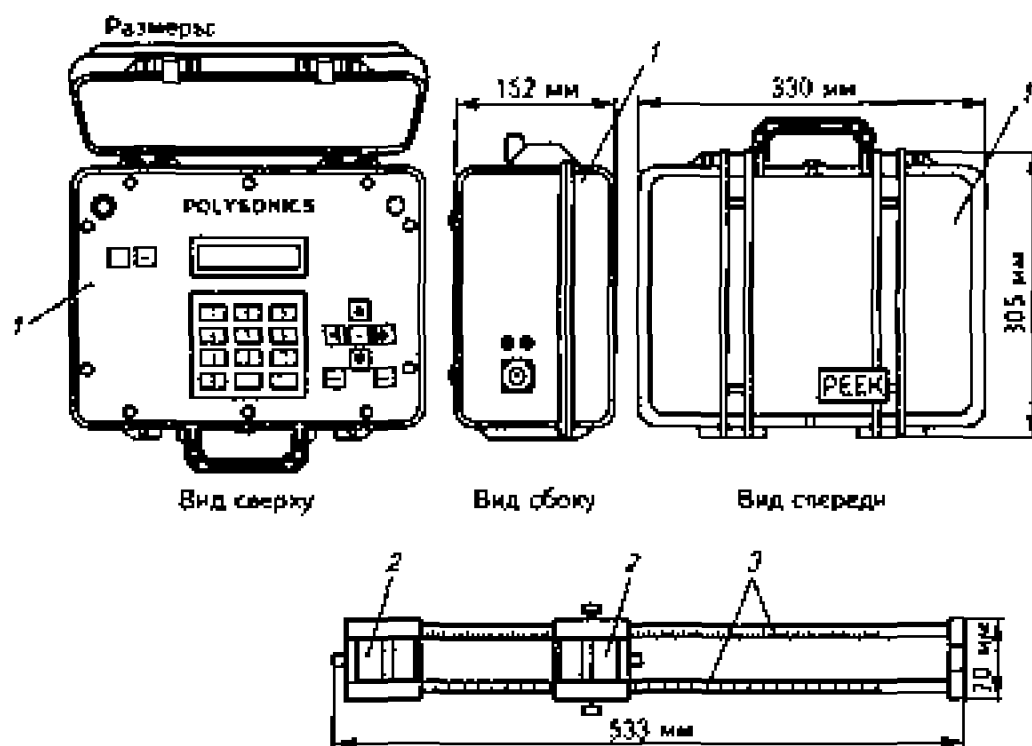
Рис. 7.10. Переносной ультразвуковой расходомер типа -Polysonics ISTT-P. 1 – кейс с измерительными и показывающими приборами, батареями электропитания; 2 – измеряющие контакты, устанавливаемые на поверхности трубопровода; 3 – рейка с направляющими для перемещения контактов 2
