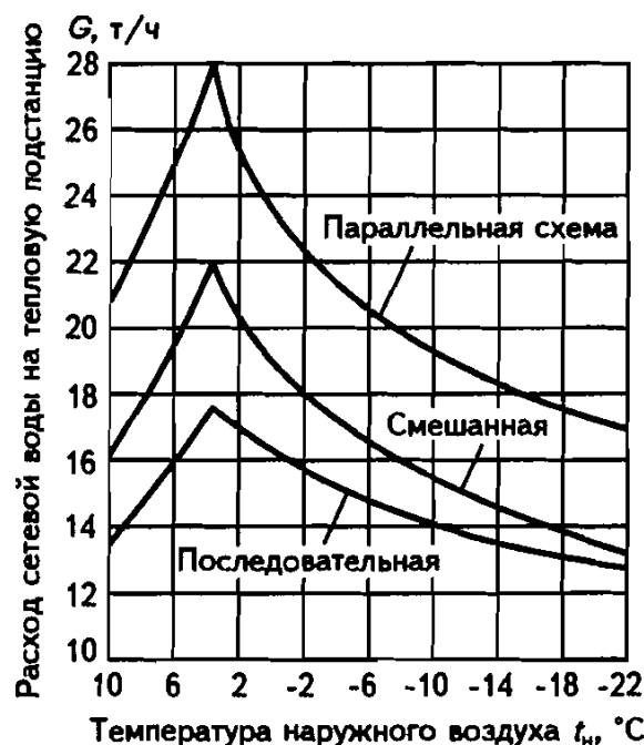
Рис. 6.37. Расходы сетевой воды на ИТП при различных схемах присоединения подогревателей горячего водоснабжения и максимальной нагрузке горячего водоснабжения. Температурный график отопительный. Расчетная нагрузка отопления Q_o = 1,16 МВт (1 Гкал/ч) при t_n = -22 °C; нагрузка ГВС: средняя Q_{\text{ГВС}}^{\text{ср}} = 0,364 МВт (0,314 Гкал/ч); максимальная Q_{\text{ГВС}}^{\text{макс}} = 0,728 МВт (0,628 Гкал/ч).
