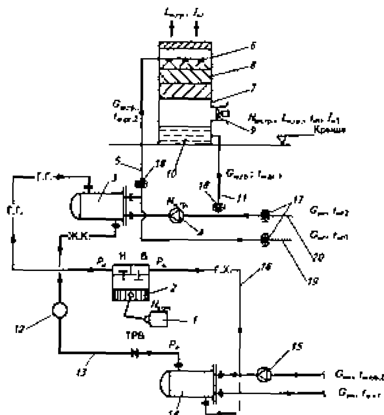
Рис. 8.1. Принципиальная схема парокомпрессионной холодильной машины с водяным конденсатором и испарителем
