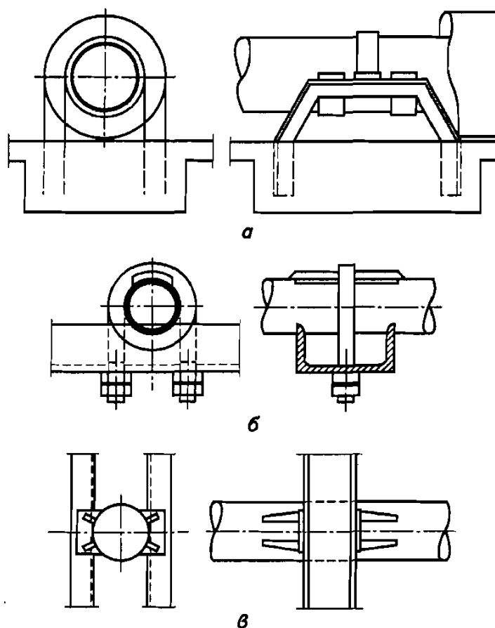
Рис. 6.22. Неподвижные опоры а — на фундаментах; б — на балке; в — на стойках
