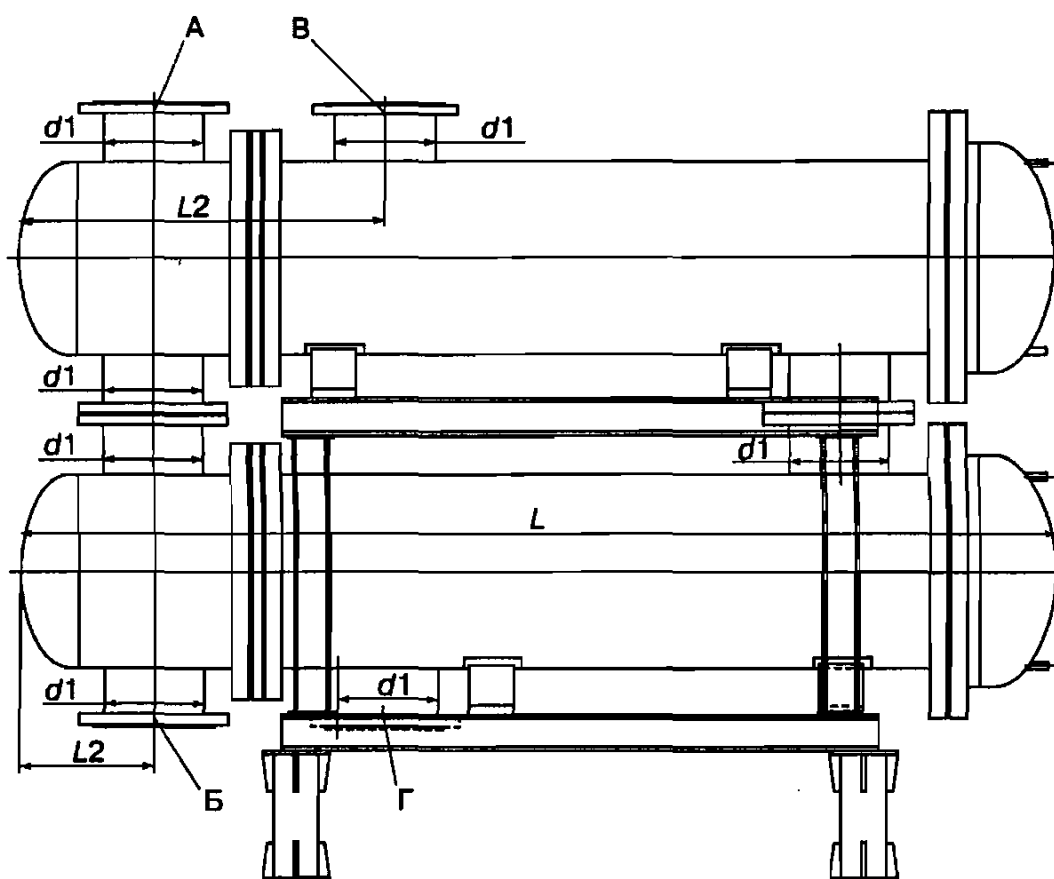
Рис. 6.42. Блок из двух подогревателей ПБМР
