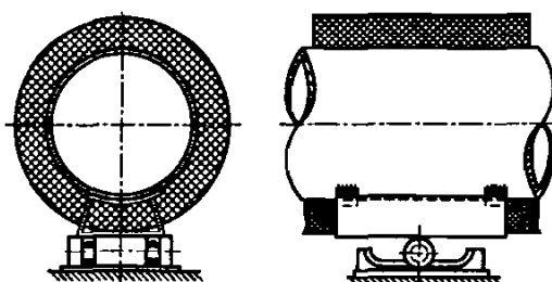
Катковая опора
