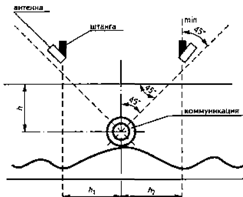
Рис. 10.16. Схема определения глубины заложения коммуникации
