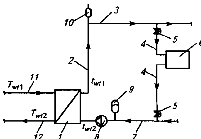
Рис. 1.4. Принципиальная схема центрального отопления здания от крупного источника теплоснабжения
