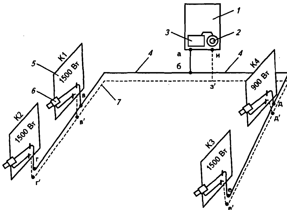
Рис. 4.28. Аксонометрическая схема квартирной системы отопления с автономным источником теплоснабжения
