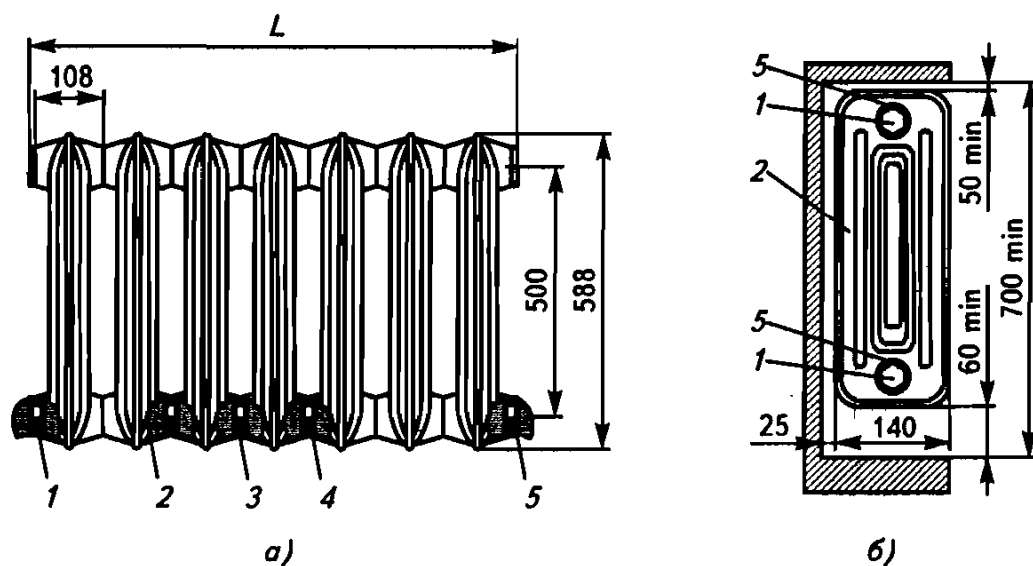
Рис. 3.2. Конструкция отопительных приборов из секций чугунных радиаторов типа МС-140
