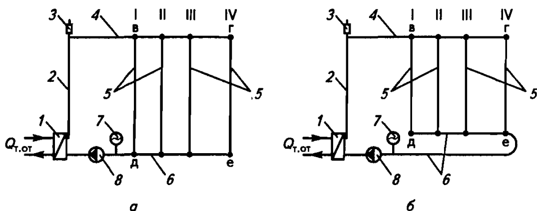
Рис. 4.25. Схемы гидравлической увязки параллельных циркуляционных колец системы отопления
