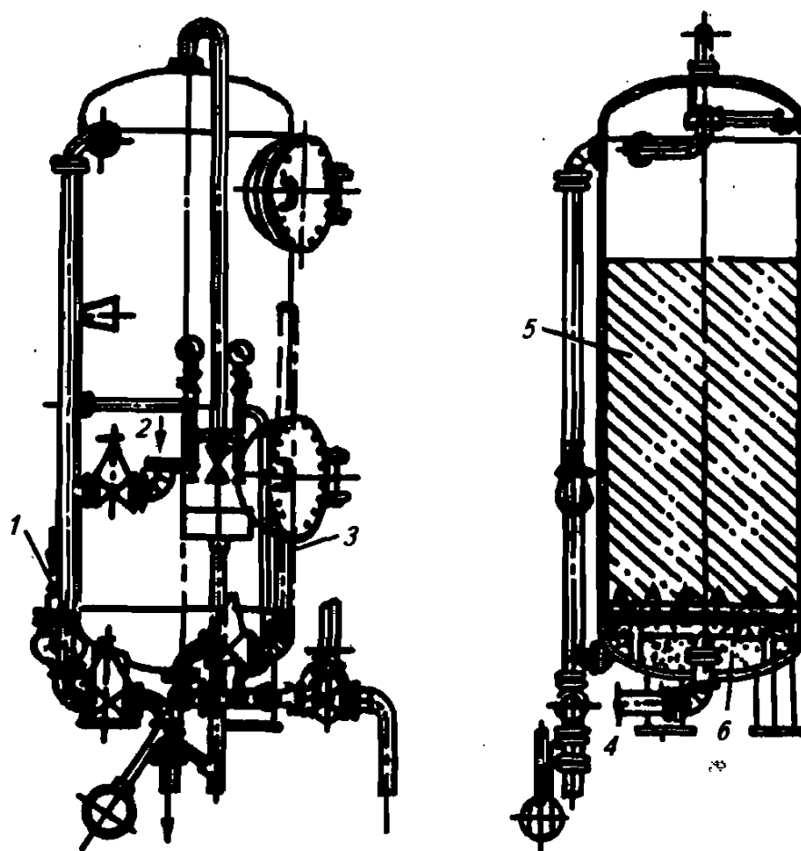
Рис. 6.51. Вертикальный катионитовый фильтр первой ступени
