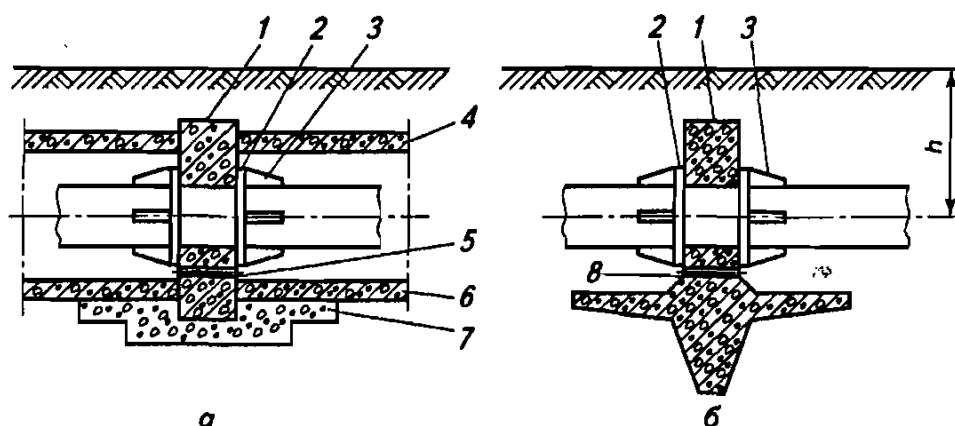
Рис. 6.21. Щитовая неподвижная опора при установке а – в непроходном канале; б – в бесканальной теплотрассе; 1 – железобетонная щитовая стенка; 2 – асбестовая прокладка; 3 – лобовая опора; 4 – перекрытие; 5 – дренажное отверстие; 6 – дно канала; 7 – опорная бетонная подушка; 8 – отверстие для дренажной трубы
