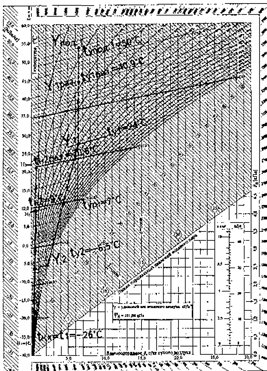
Рис. 9.10. Построение на t - d -диаграмме режима работы в климате Москвы установки утилизации с пластинчатым теплообменником и размораживанием его по новому методу (по схеме на рис. 9.9).
