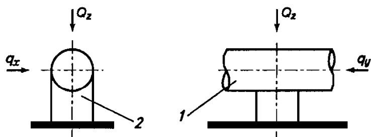
Рис. 6.18. Схема нагрузок на опору 1 – труба; 2 – подвижная опора; Q_z – вертикальное давление трубопровода на подвижную опору; q_y – продольная составляющая силы трения (вдоль оси трубы); q_x – боковая составляющая силы трения (поперек оси трубы)
