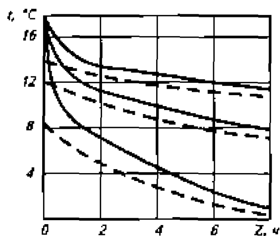
Рис. 10.1. Линии падения температуры внутреннего воздуха (—) и внутренней поверхности наружной стены (---) здания после отключения отопления
