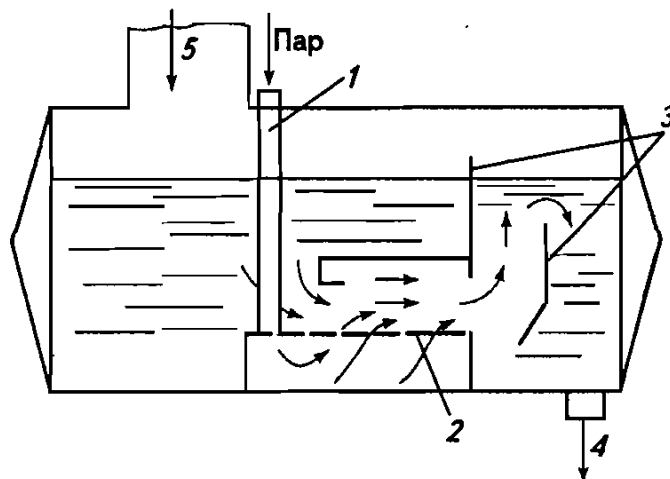
Рис. 6.46. Схема барботажного устройства ЦКТИ
