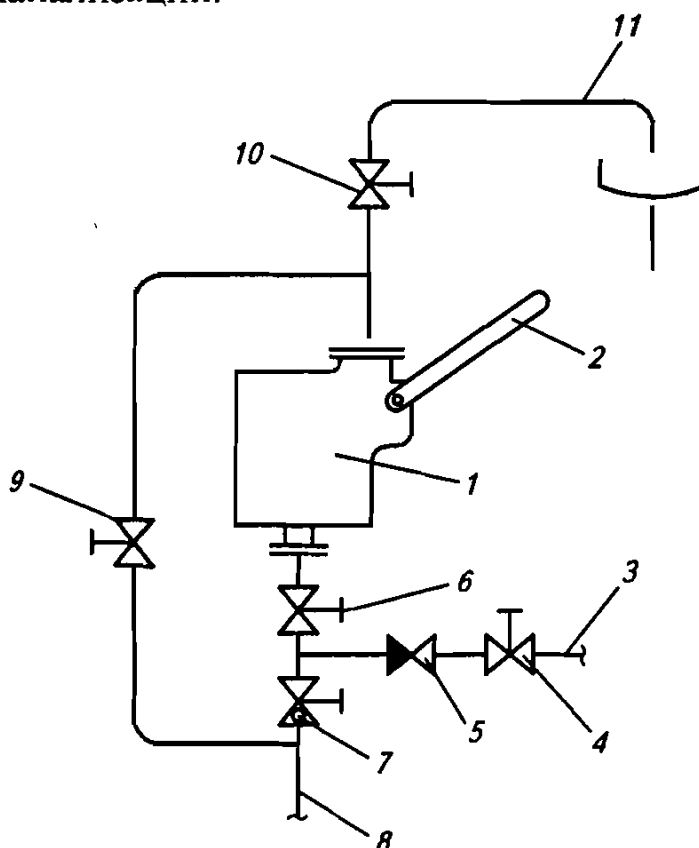
Рис. 4.11. Принципиальная схема подключения ручного насоса к системе отопления, водопроводу и канализации
