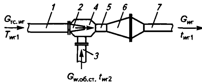
Рис. 4.20. Принципиальная схема включения водоструйного элеватора 1 – соединительный трубопровод подачи сетевой воды из системы теплоснабжения; 2 – коническое сопло; 3 – трубопровод обратной воды системы отопления; 4 – камера смешения; 5 – горловина; 6 – диффузор элеватора; 7 – подающий трубопровод в систему отопления
