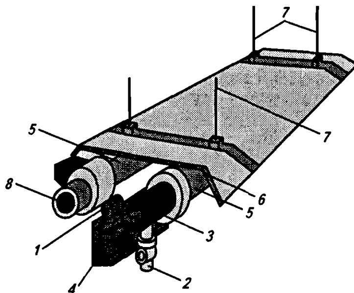
Рис. 5.4. Схема нагревателя лучистого типа НЛТ на газовом топливе 1 – подводка природного газа; 2 – забор воздуха для сжигания газа; 3 – газовая горелка с вентилятором; 4 – автоматика горения газа; 5 – трубы лучистого нагрева от сгорания газа; 6 – отражательный щиток с теплоизоляцией с верхней стороны; 7 – подвески агрегата НЛТ к конструкциям перекрытия; 8 – выход в верхнюю зону помещения продуктов сгорания газа
