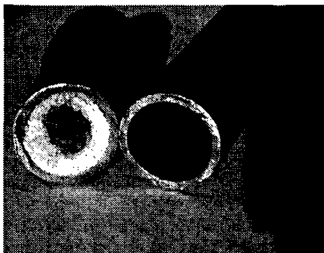
Рис. 6.53. Конвективные трубы ( d = 28 мм) водогрейного котла до и после очистки по технологии ООО «ЭкоМИРТ»
