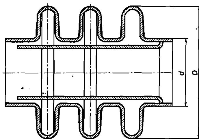
Рис. 6.25. Схема трехволнового сильфонного компенсатора (Компенсирующая способность его составляет 50–150 мм)
