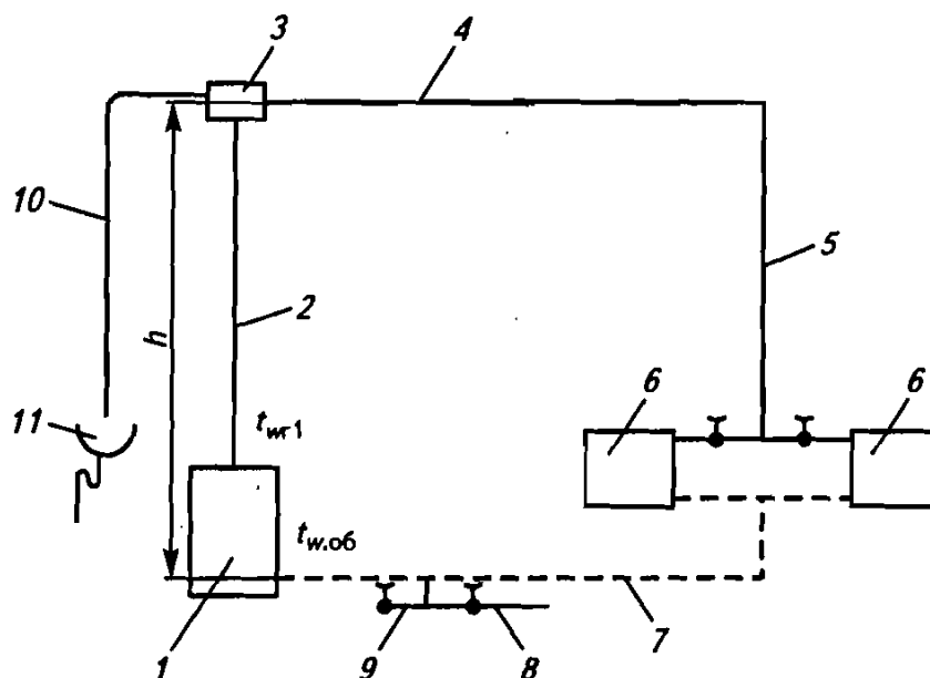
Рис. 4.1. Квартирная система отопления с естественной циркуляцией горячей воды
