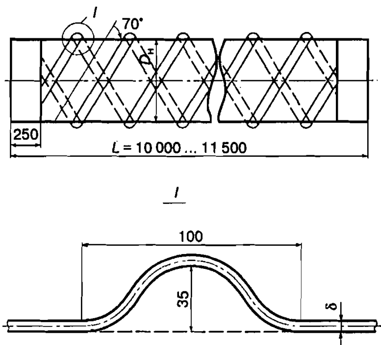
Рис. 6.26. Самокомпенсирующаяся стальная труба и гофра (узел 1)
