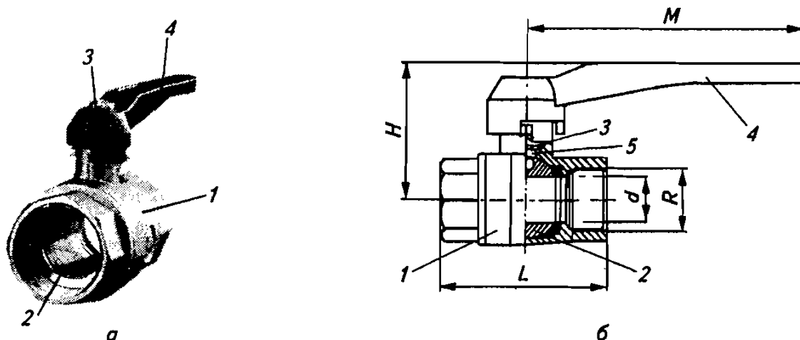
Рис. 4.17. Шаровой полнопроходной кран с внутренней соединительной резьбой а – внешний вид; б – конструктивная схема; 1 – корпус латунный или стальной; 2 – запорный шар с отверстием; 3 – шток шарового крана; 4 – рукоятка поворота штока; 5 – сальниковое уплотнение
