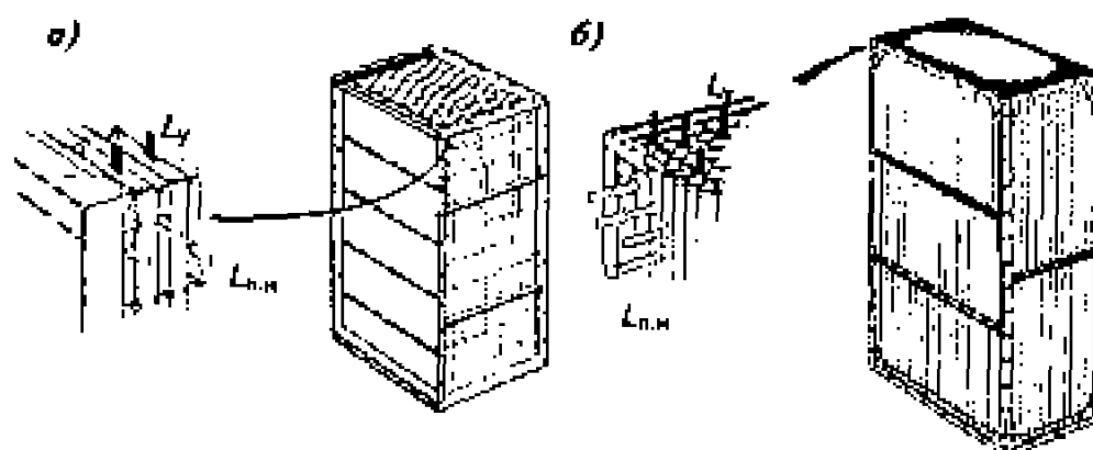
Рис. 9.7. Конструктивная схема рекуперативного теплообменника из пластинчатых и трубчатых каналов прохождения приточного и вытяжного воздуха
