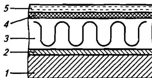
Рис. 2.1. Устройство кровельного покрытия со слоем теплоизоляции из плит «Rockwool» по железобетонному основанию.
