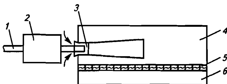
Рис. 5.7. Принципиальная схема газового инфракрасного нагревателя 1 – подвод газа; 2 – автоматика горелочного устройства; 3 – смешивающая камера сгорания; 4 – распределительная камера продуктов сгорания газа; 5 – нагреваемые керамические перфорированные плитки; 6 – направляющий диффузор потока излучения
