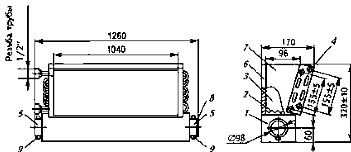
Рис.7.18 Конструктивная схема доводчика эжекционного типа ДЭ 2.6.140/180 1 – камера первичного воздуха; 2 – блок эжектирующих сопел; 3 – смешительная камера; 4 – теплообменники; 5 – патрубок; 6 – стенка задняя; 7 – стенка боковая; 8 – заглушка; 9 – хомут
