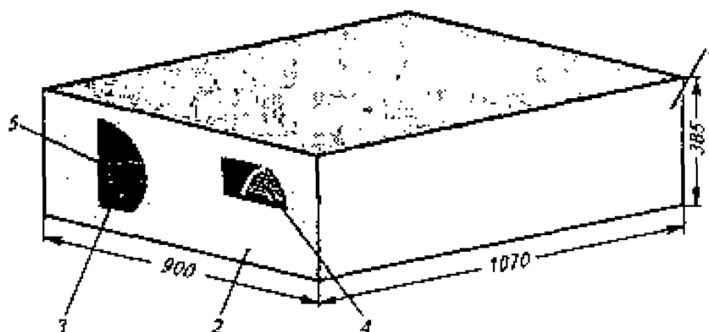
Рис. 8.4. Внешний вид приточно-вытяжного агрегата «Сибирь», работающего в режимах нагрева зимой (тепловой насос) и летом – охлаждения приточного наружного воздуха
