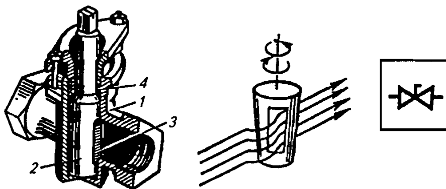
Рис. 4.16. Пробочный запорный кран 1 – корпус; 2 – пробка; 3 – отверстие в пробке; 4 – сальник
