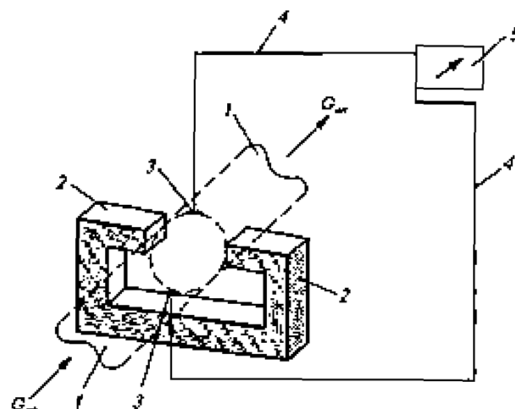
Рис. 7.7. Принципиальная схема электромагнитного метода измерения расхода воды
