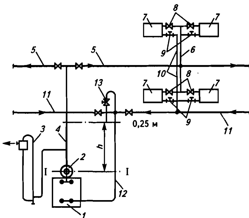
Рис. 5.1. Схема паровой системы отопления низкого давления со средним расположением подающего магистрального вертикального паропровода 1 – паровой котел; 2 – паросборник; 3 – предохранительное устройство; 4 – вертикальный магистральный паропровод; 5 – горизонтальные магистральные распределительные паропроводы; 6 – вертикальные парораспределительные стояки; 7 – отопительный прибор; 8 – паровой вентиль; 9 – тройник с пробкой; 10 – вертикальные стояки для сбора конденсата; 11 – горизонтальный сборный трубопровод конденсата; 12 – трубопровод возврата конденсата в котел; 13 – выпуск воздуха из системы отопления
