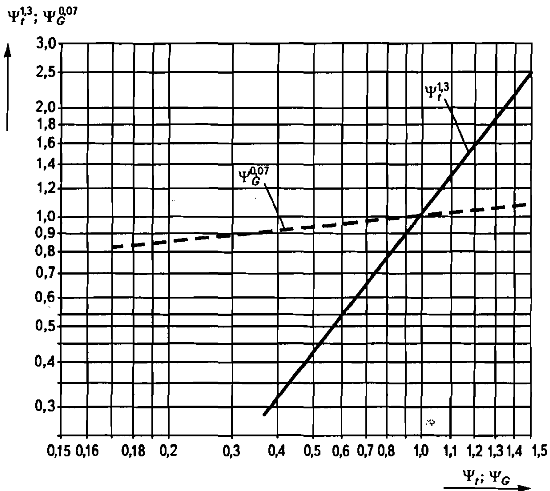
Рис. 4.27. Построение в логарифмических координатах степенной зависимости отношения действительных средних температур в отопительном приборе \Delta t_{w, \text{ср.п}} к расчетному перепаду в 70^\circ\text{C} , что отвечает степенному показателю \psi_t^{1,3} , и отношение действительных расходов горячей воды через отопительный прибор G_{\text{вт}} , кг/ч, по отношению к паспортному расходу 360 кг/ч, что отвечает степенному показателю \psi_G^{0,07}
