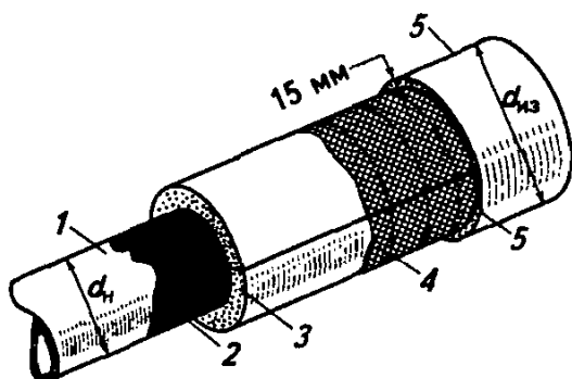
Рис. 6.28. Подвесная теплоизоляционная конструкция 1 – труба; 2 – антикоррозионное покрытие; 3 – мат из минеральной ваты; 4 – стальная сетка; 5 – асбестоцементная штукатурка
