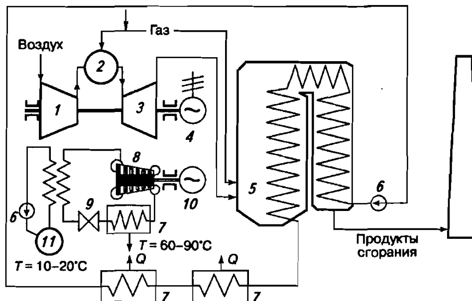
Рис. 6.10. Принципиальная тепловая схема когенерационной энергетической установки с газотурбинной надстройкой (ГТУ) к водогрейному котлу совместно с тепловым насосом
