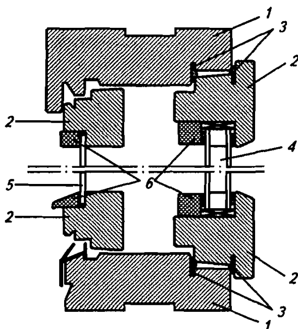
Рис. 2.3. Теплозащитная конструкция окон
