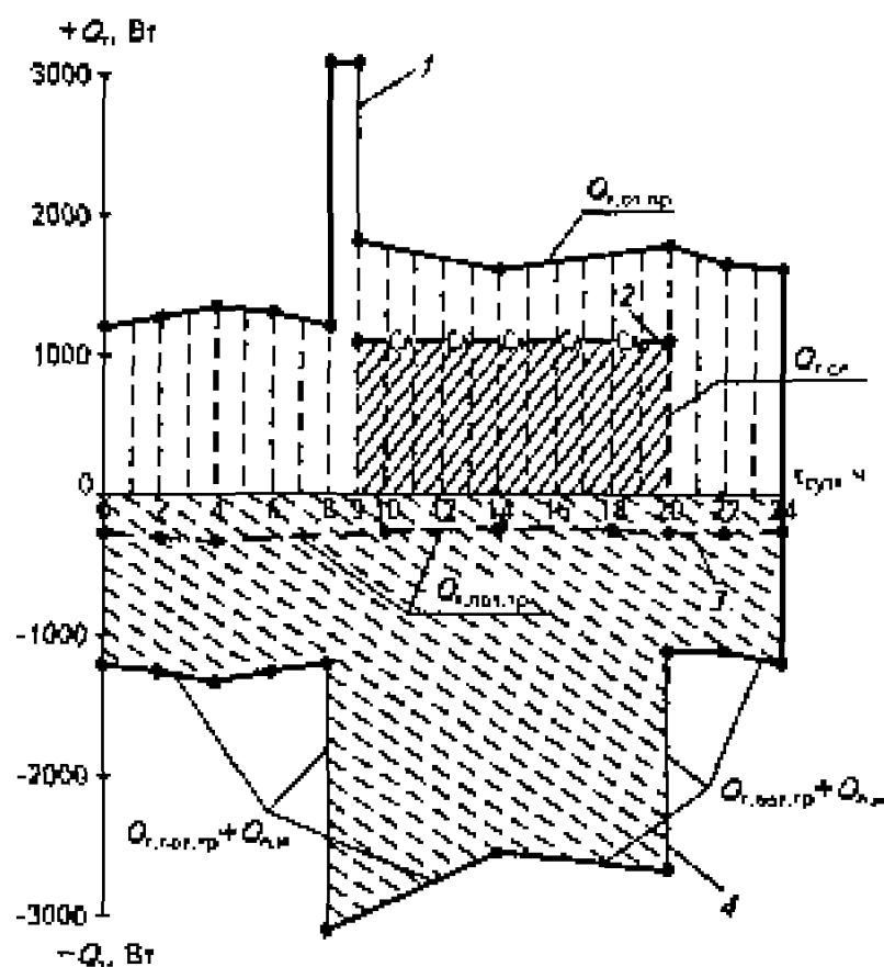
Рис. 7.17. График изменения суточной потребности мощности отопительного прибора в служебном помещении
