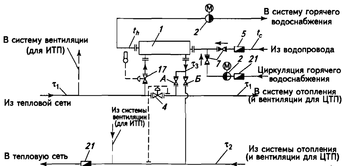
Рис. 6.35. Одноступенчатая предвключенная (А – открыта, Б – закрыта) или параллельно включенная (А – закрыта, Б – открыта) схема присоединения водоподогревателей ГВС с зависимым присоединением систем отопления при отсутствии регуляторов расхода теплоты на отопление и теплосчетчика в ЦТП и ИТП в закрытых СЦТ
