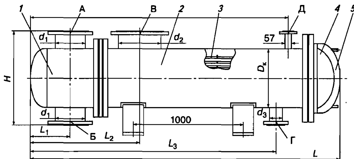
Рис. 6.43. Схема подогревателя ППМР
