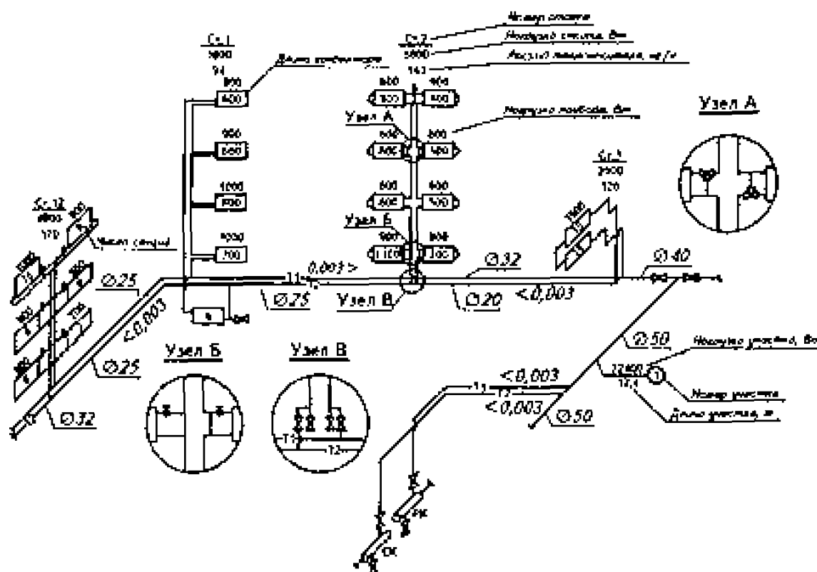
Рис. 9.6. Оформление аксонометрической схемы системы отопления с нижней разводкой и различными способами присоединения отопительных приборов
