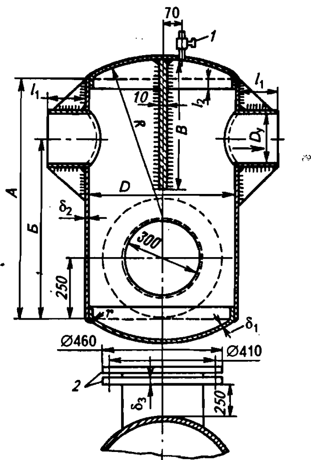
Рис. 6.52. Грязевик для тепловых сетей D_y = 250-800 мм
