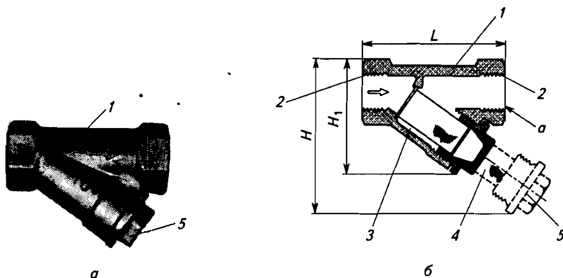
Рис. 4.15. Конструктивные особенности водяного фильтра для установки на трубопроводах систем отопления и водоснабжения
