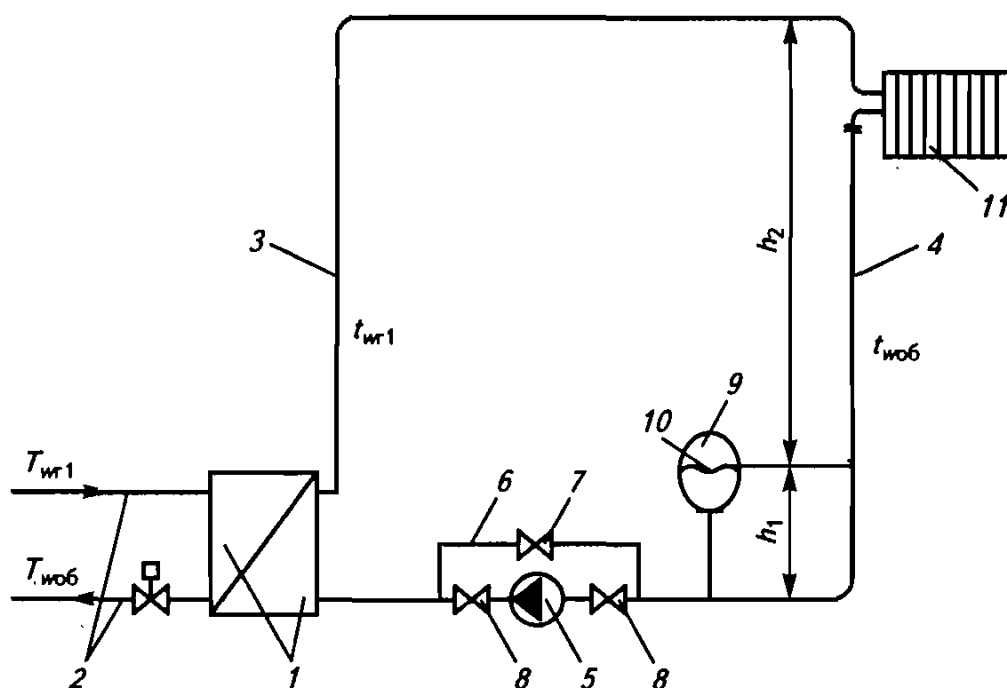
Рис. 4.13. Принципиальная схема присоединения герметичного расширительного бака в системе отопления
