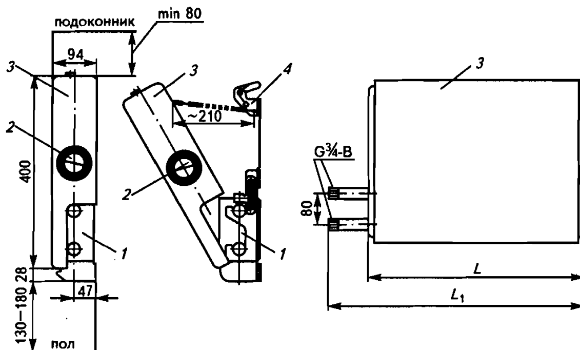
Рис. 3.5. Конструкция отечественного отопительного прибора-конвектора ОАО «Сантехпром» малой глубины с ручным регулированием теплоотдачи 1 – нагревательный теплообменник; 2 – поворотные ручки регулировочного воздушного клапана; 3 – съемный кожух; 4 – скобы для навешивания конвектора на кронштейны, заделанные в стену под подоконником
