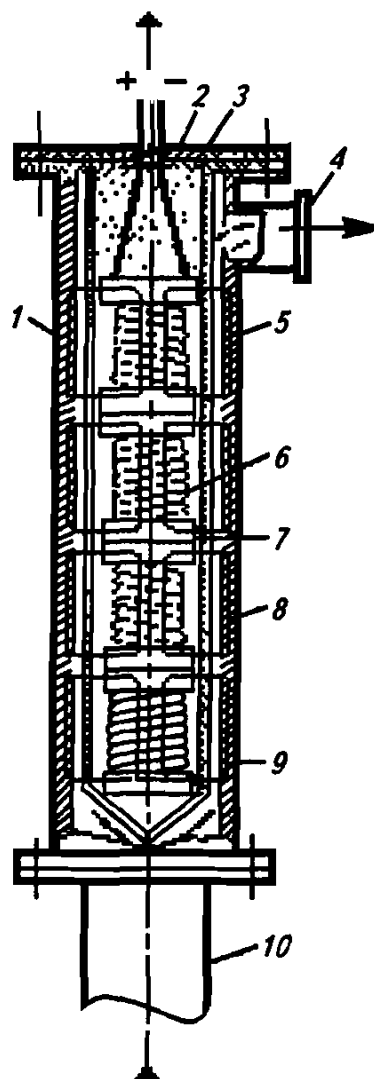
Рис. 6.50. Схема электромагнитного аппарата производительностью до 50 м³/ч
