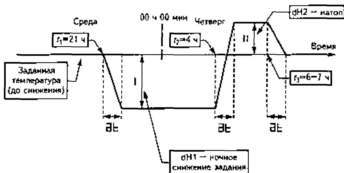
Рис. 7.15. График суточного изменения тепловой мощности системы отопления, программа которого автоматически контролируется в зависимости от температуры наружного воздуха и времени суток
