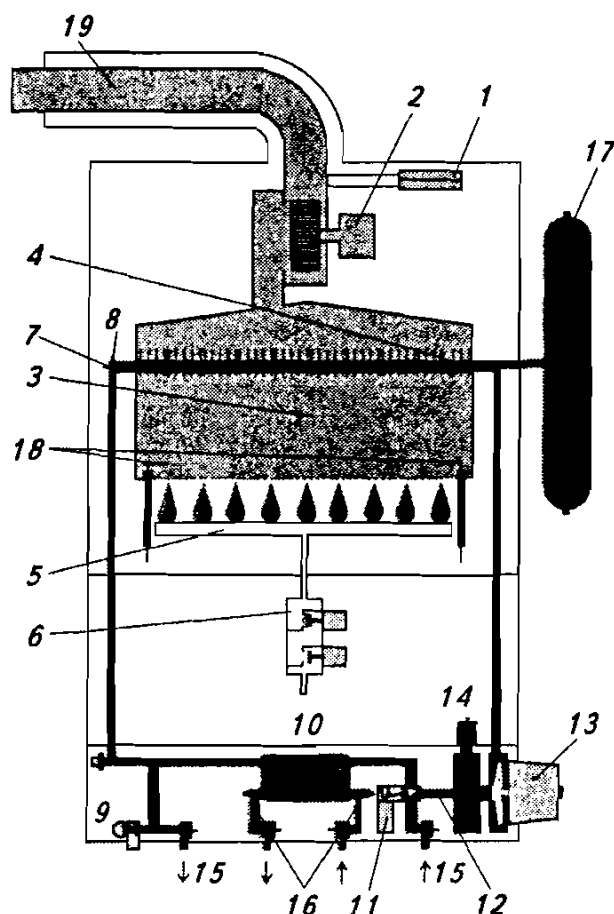
Рис. 4.9. Функциональная схема газового котла с закрытой камерой горения и двумя контурами нагрева воды для систем квартирного отопления и горячего водоснабжения
