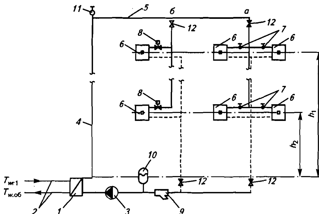
Рис. 4.5. Двухтрубная система отопления с верхней разводкой
