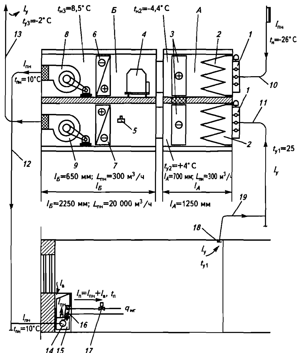
Рис. 4.7. Принципиальная схема водяной системы отопления, совмещенной с приточно-вытяжной вентиляцией
