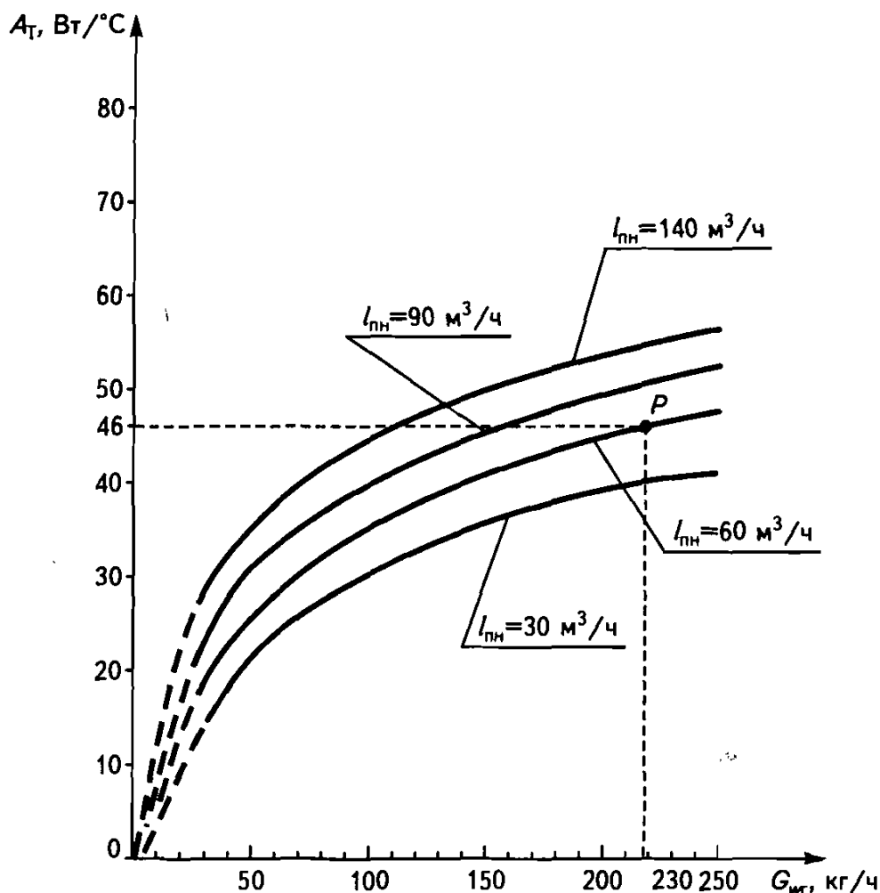
Рис. 4.8. Графическая зависимость удельного теплового показателя теплообменника (поз. 16 рис. 4.7) в доводчике эжекционном типа ДЭ 1.6 30/90
