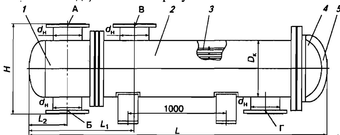
Рис. 6.41. Схема подогревателя ПВМР
