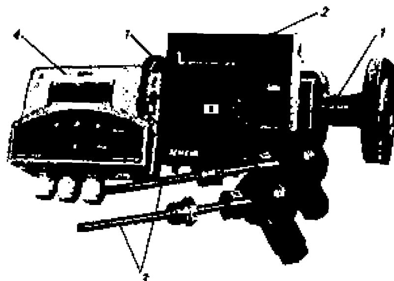
Рис. 7.9. Части теплосчетчика ТСК7 с ультразвуковым водосчетчиком 2WR 1 – корпус ультразвукового водосчетчика 2WR с фланцами для присоединения к трубопроводам сети теплоснабжения; 2 – устройство генерации ультразвука и регистрации расхода жидкости; 3 – термометры сопротивления; 4 – вычислитель ВКТ-7 с автономным электропитанием от батарей
