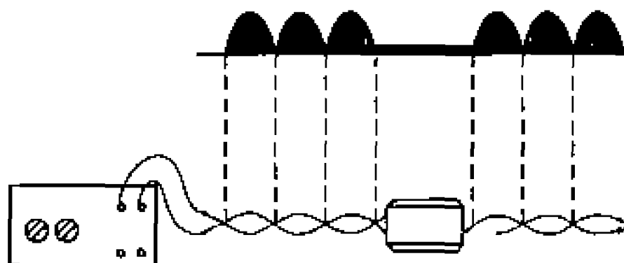
Рис. 10.19. Характер изменения сигналов датчика при поиске кабельных муфт
