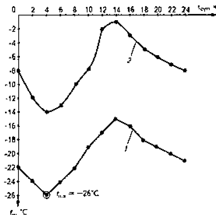
Рис. 7.14. График изменения за сутки температуры наружного воздуха в два месяца отопительного периода 1 – в январе; 2 – в марте
