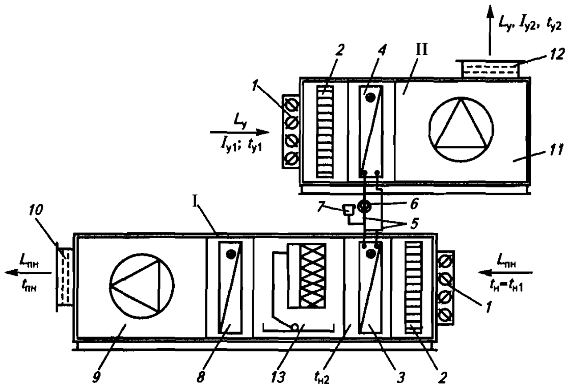
Рис. 2.5. Схемы приточного I и вытяжного II агрегатов по энергосберегающей технологии приготовления приточного наружного воздуха
