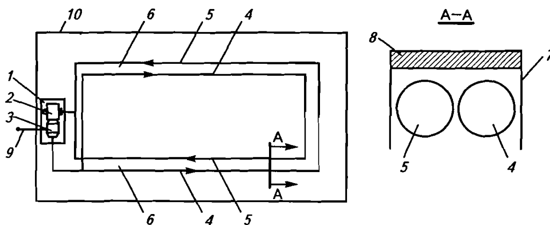
Рис. 1.2. Принципиальная схема местного лучистого газозвоздушного отопления помещения
