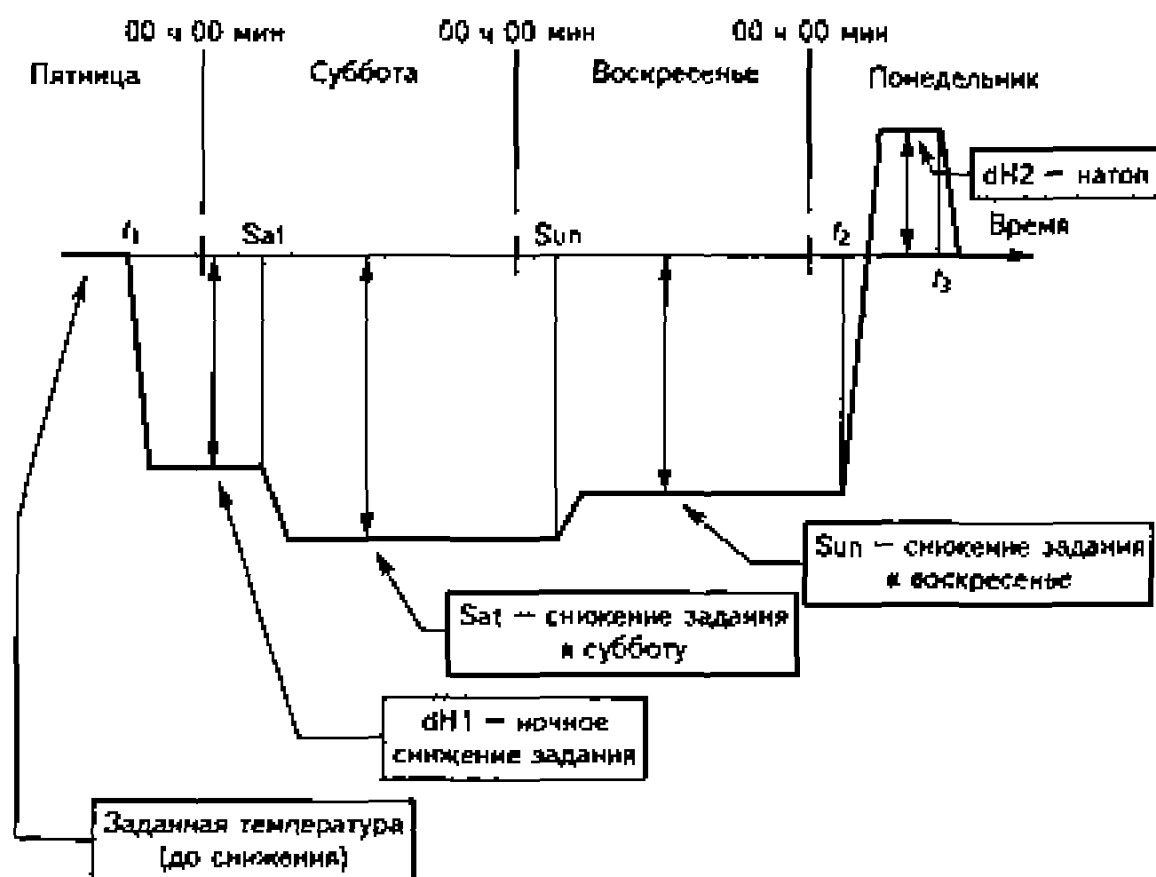
Рис. 7.16. График изменения тепловой мощности системы отопления в субботу и воскресенье (выходные и праздничные дни)
