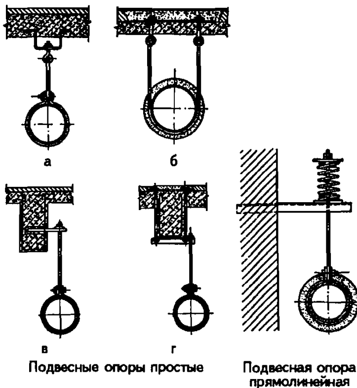
Рис. 6.20. Варианты подвесных опор трубопроводов а – для продольных и поперечных перемещений; б – для продольных перемещений; в – с непосредственной заделкой в балку; г – с обвязкой балки
