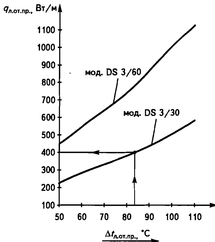
Рис. 5.3. Графики зависимости удельного теплового потока q_{\text{л.от.пр.}} от перепада температур \Delta t_{\text{л.от.пр.}} подвесных панелей лучистого отопления моделей DS 3/30 и DS 3/60 итальянской фирмы «Sabiana»
