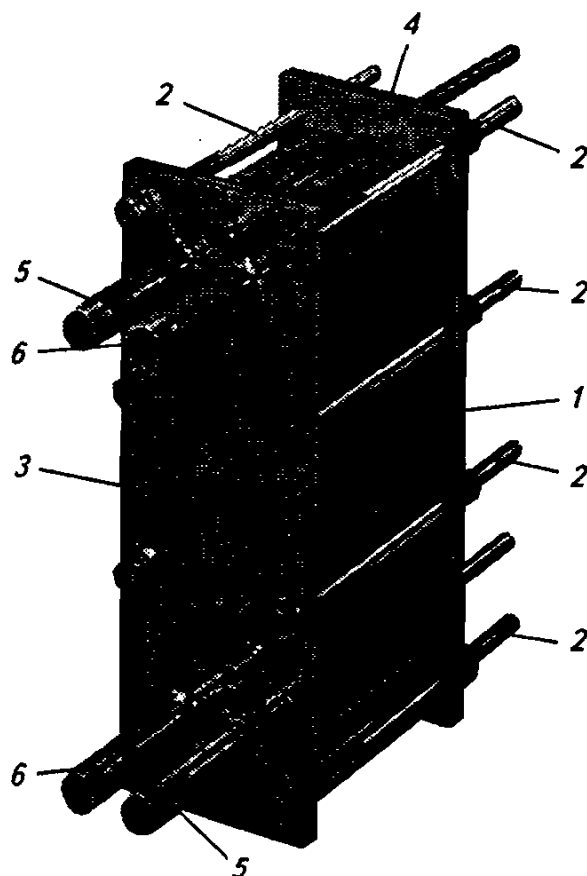
Рис. 4.23. Собранный пластинчатый теплообменник «жидкость–жидкость» 1 – тонкие штампованные пластины; 2 – стяжные болты; 3, 4 – передняя и задняя массивная плита; 5 – патрубки для присоединения трубопроводов к сети теплоснабжения; 6 – патрубки для присоединения циркуляционных трубопроводов системы отопления
