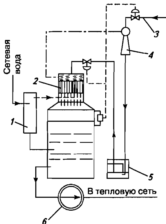
Рис. 6.47. Принципиальная схема вакуум-деаэрационной установки 1 – вакуум-испаритель; 2 – деаэрационная головка; 3 – вход сырой воды; 4 – водоструйный эжектор; 5 – бак-газоотделитель; 6 – подпиточный насос тепло-сети
