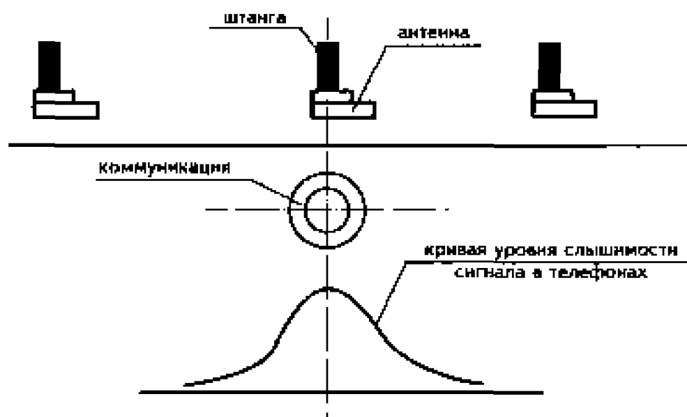
Рис. 10.14. Схема поиска коммуникации по максимуму звукового сигнала
