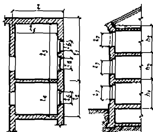
Рис. 9.1. Схема обмеров ограждающих конструкций в отапливаемом помещении
