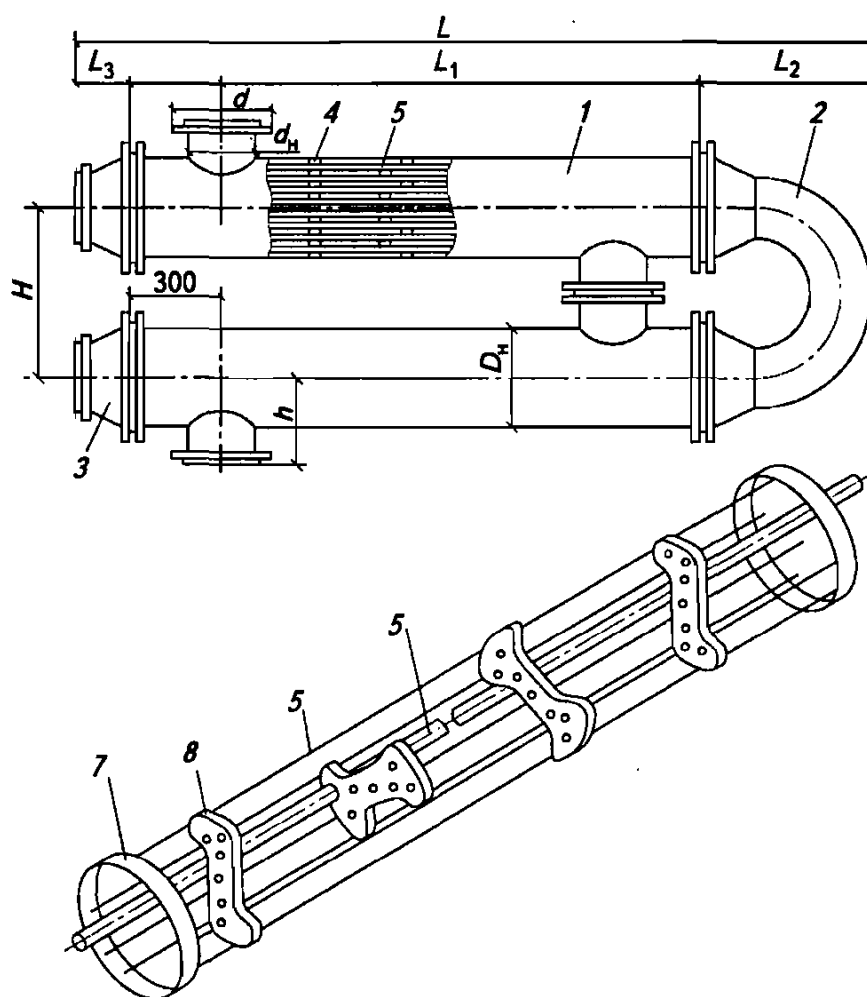
Рис. 6.34. Общий вид горизонтального секционного кожухотрубного водоподогревателя (ВВП) с опорами-турбулизаторами по ГОСТ 27590
