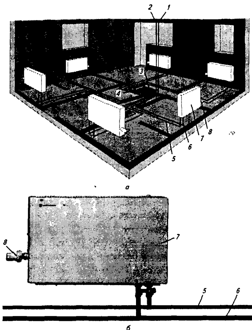
Рис. 4.6. Принципиальная схема квартирной двухтрубной системы отопления с нижней разводкой с применением в качестве отопительных приборов отечественных конвекторов «Сантехпром Авто»
