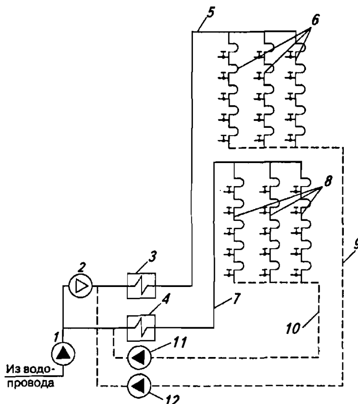
Рис. 6.40. Схема двухзонной системы ГВС высотного здания
