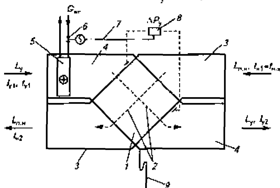
Рис. 9.9. Принципиальная схема применения пластинчатого теплоутилизатора в климате России
