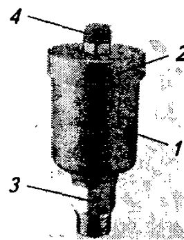
Рис. 4.14. Автоматический воздухоотводчик 1 — корпус; 2 — крышка; 3 — штуцер с резьбой диаметром 3/8" для присоединения к системе отопления; 4 — заглушка с воздуховыпускным отверстием
