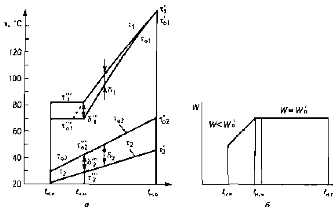
Рис. 10.22. Диспетчерские графики регулирования температур (а) и расхода горячей воды (б) (при центральном качественном регулировании совмещенной нагрузки отопления и горячего водоснабжения при закрытой системе ЦТ)
