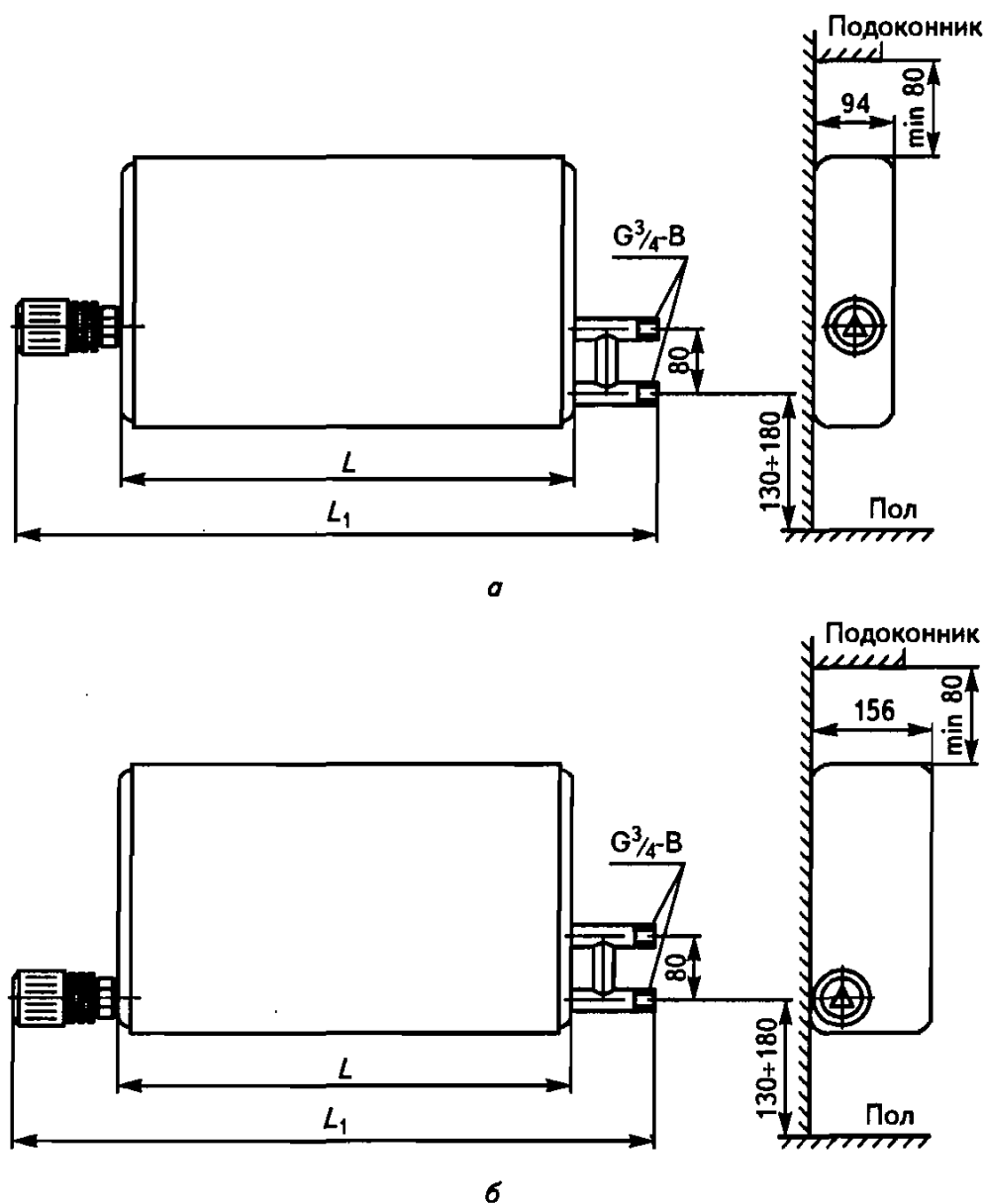
Рис. 3.12. Отечественная конструкция отопительных конвекторов со встроенным терморегулятором RTD для количественного регулирования теплопроизводительности
