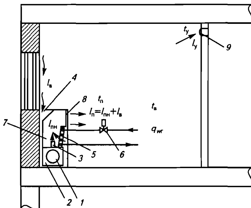
Рис. 3.11. Конструктивная схема встраивания доводчика эжекционного в подоконную нишу
