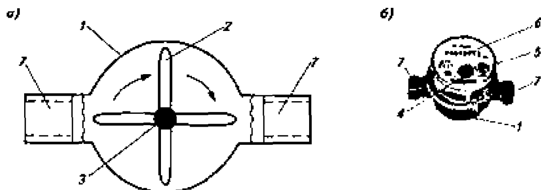
Рис. 7.6. Крыльчатый счетчик расхода воды
