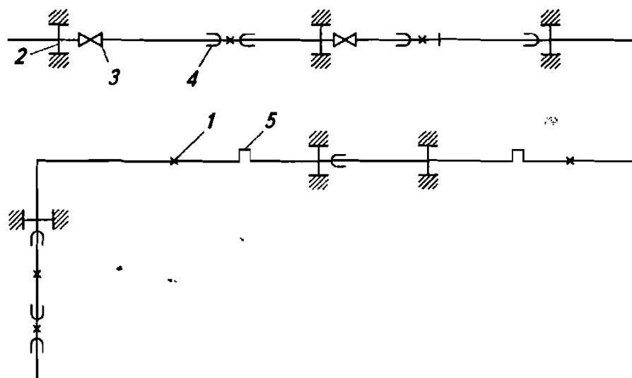
Рис. 6.23. Схемы разгруженных и неразгруженных опор трубопроводов 1 – разгруженная опора; 2 – неразгруженная опора; 3 – запорный орган; 4 – сальниковый компенсатор; 5 – гнутый компенсатор
