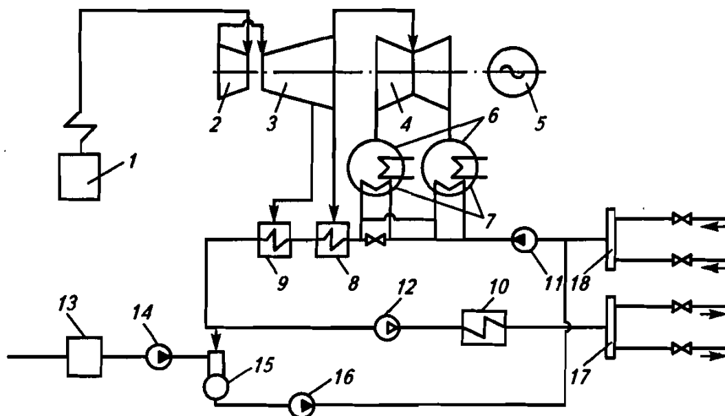
Рис. 6.4. Тепловая схема ТЭЦ с теплофикационной турбиной Т100-130 1 – паровой котел; 2, 3 и 4 – соответственно части высокого, среднего и низкого давления турбины; 5 – электрический генератор; 6 – конденсаторы; 7 – встроенные в конденсатор пучки для подогрева сетевой воды; 8 и 9 – подогреватели сетевой воды; 10 – водогрейный (пиковый) котел; 11 и 12 – сетевые насосы первого и второго подъема; 13 – химическая водоподготовка; 14 – насос; 15 – деаэратор; 16 – подпиточный насос; 17 и 18 – коллекторы подаваемой и возвращаемой воды
