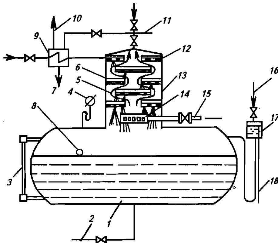
Рис. 6.45. Атмосферный-деаэратор смешивающего типа
