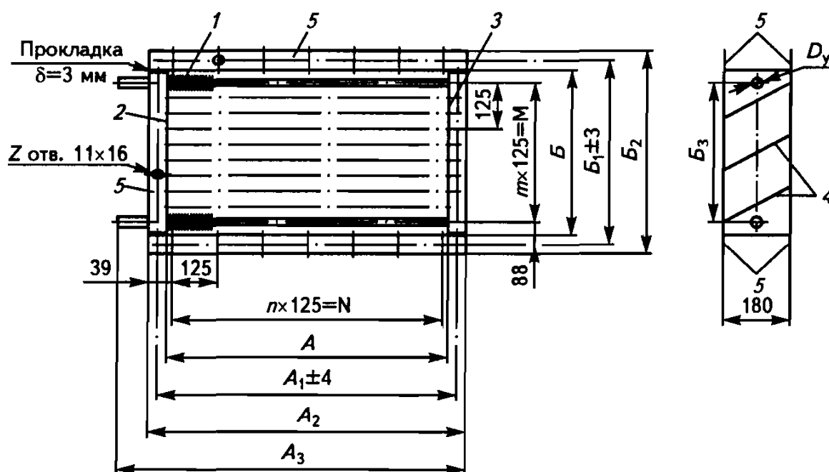
Рис. 3.6. Конструкция теплообменников для нагрева воздуха калориферов КСк3 и КСк4
