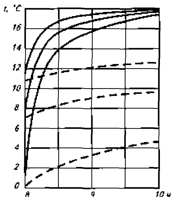
Рис. 10.2. Кривые изменения температуры внутреннего воздуха и внутренней поверхности наружной стены при включении отопления – нагоне
