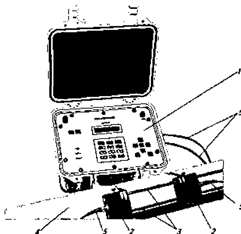
Рис. 7.11. Применение переносного ультразвукового расходомера Поз. 1–3 одинаковы с поз. рис. 7.10; 4 – трубопровод с проходящей по нему жидкостью; 5 – соединительные кабели между контактами 2 и измерительными приборами в кейсе 7
