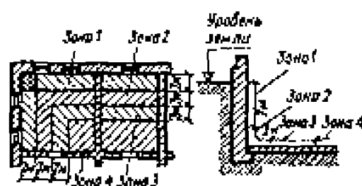
Рис. 9.2. Схема разбивки пола по грунту и заглубленных стен на зоны обмера и вычисления поверхностей
