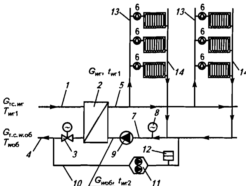
Рис. 4.22. Принципиальная схема включения независимо присоединенной системы отопления (с циркуляционным насосом) к централизованной системе теплоснабжения
