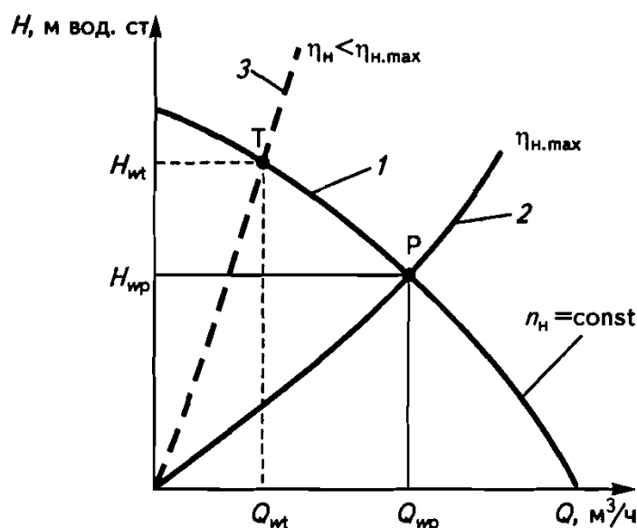
Рис. 3.13. Рабочие характеристики насоса (кривая 1) и характеристика трубопроводной сети (кривые 2 и 3) при постоянной частоте вращения рабочего колеса
