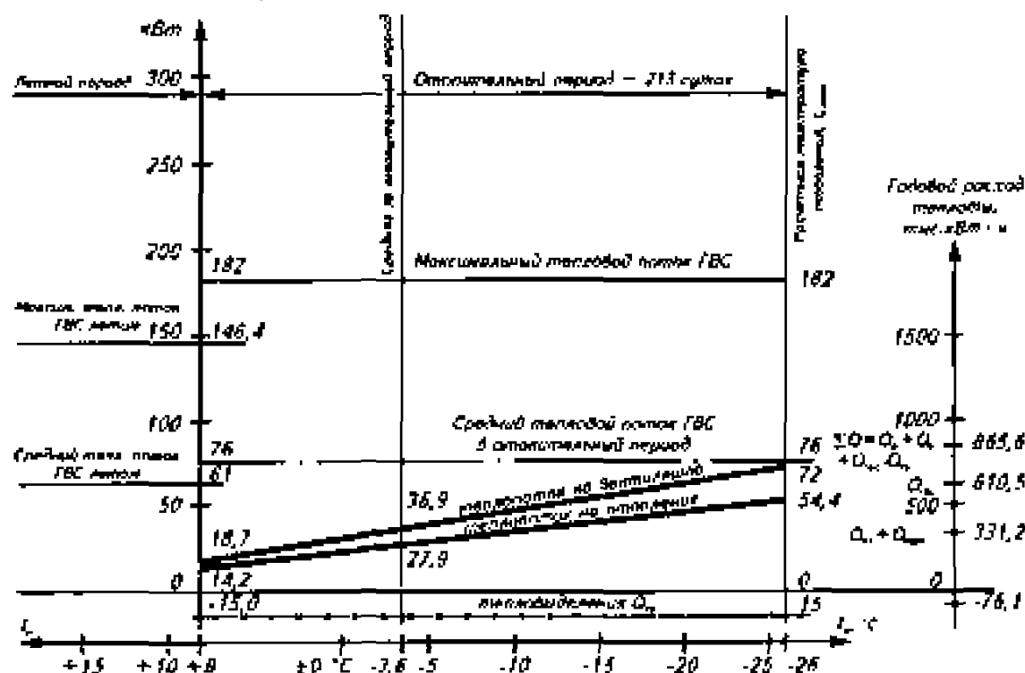
Рис. 10.3 Графики изменения тепловых нагрузок отопления, вентиляции и горячего водоснабжения жилого дома в зависимости от t_{\text{нар.средн}} (к примерам 6.1 и 7.1)
