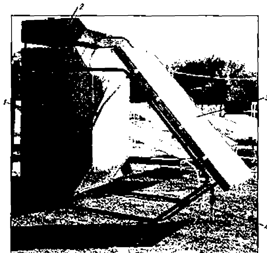
Рис. 8.7. Отечественная мобильная душевая кабина с горячим водоснабжением от солнечного коллектора
