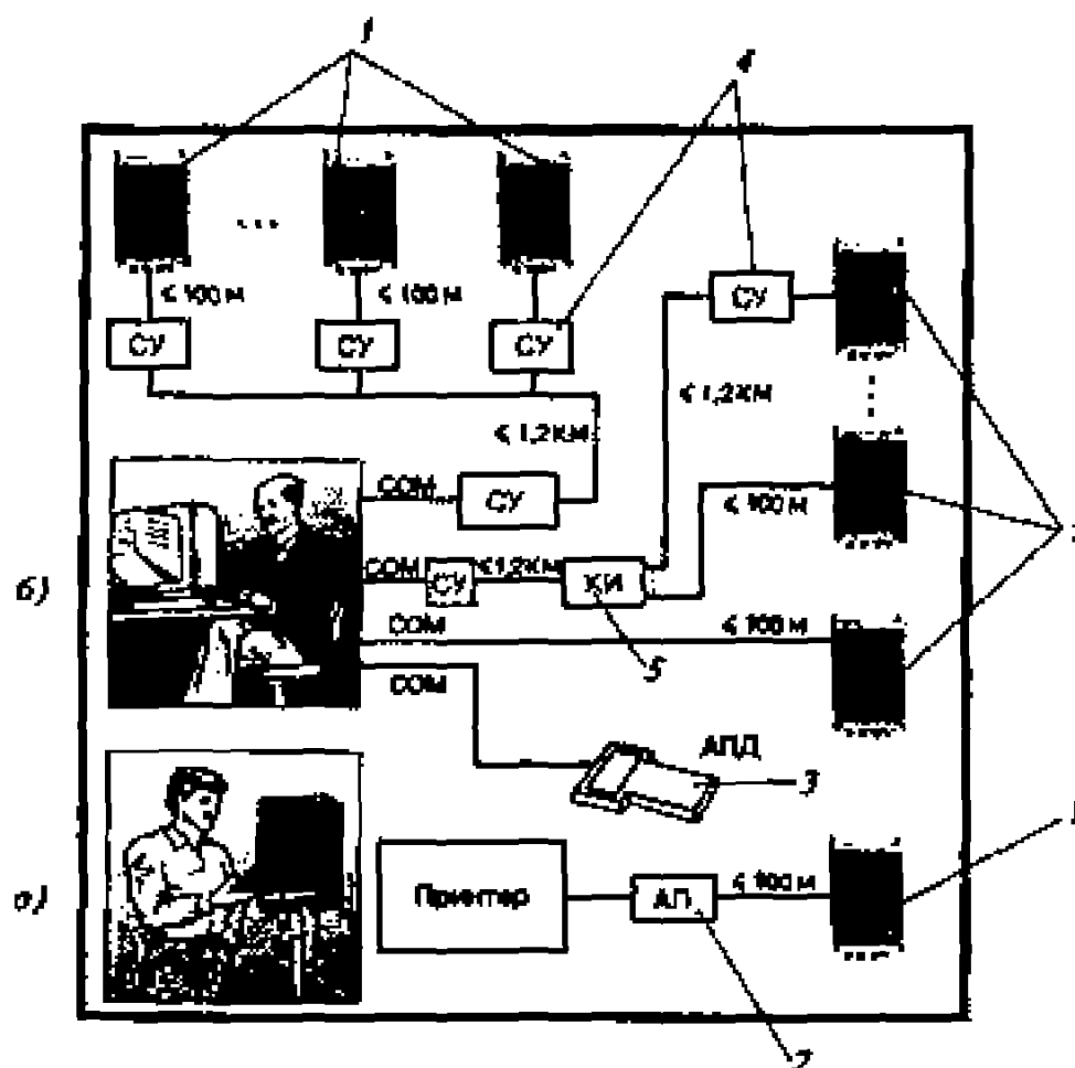
Рис. 7.4. Принципиальная схема присоединения теплосчетчика SA-94/2 к различным устройствам учета и информации ИТЭ а – индивидуальный учет; б – дистанционный групповой учет; 1 – теплосчетчик SA-94/2; 2 – адаптер принтера AD-3301; 3 – адаптер переноса данных AD-2301; 4 – согласующее устройство AD-1201; 5 – коммутатор интерфейса SAQ-1202
