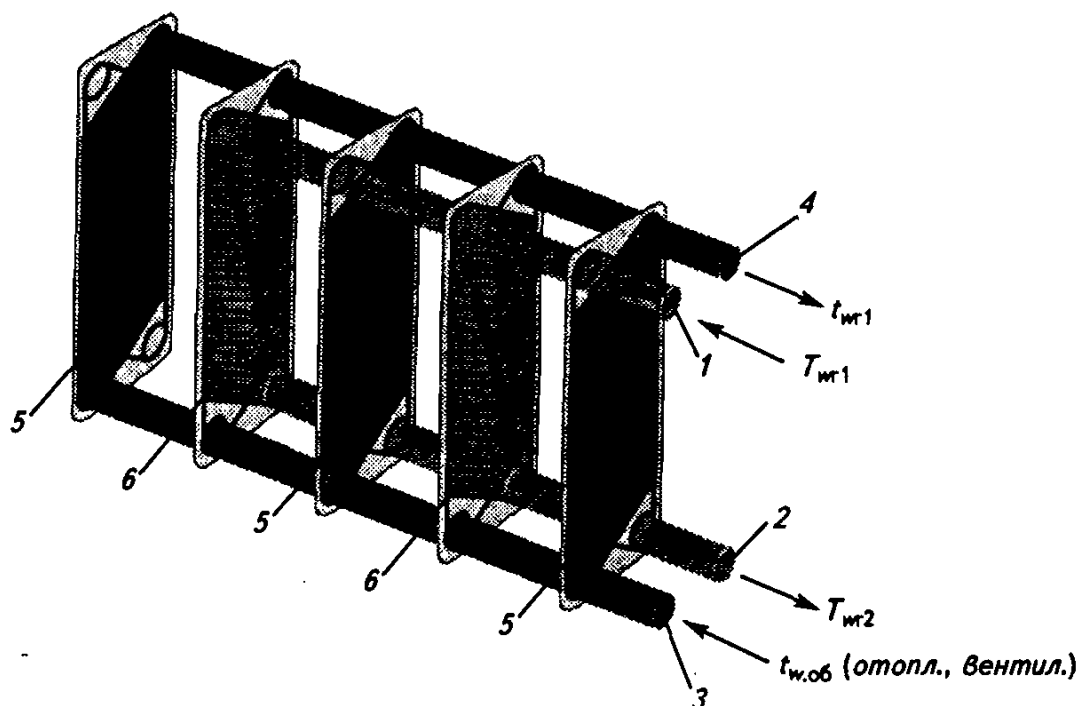
Рис. 4.24. Конструктивная схема движения потоков жидкости по каналам гофрированных пластин теплообменника «жидкость–жидкость»
