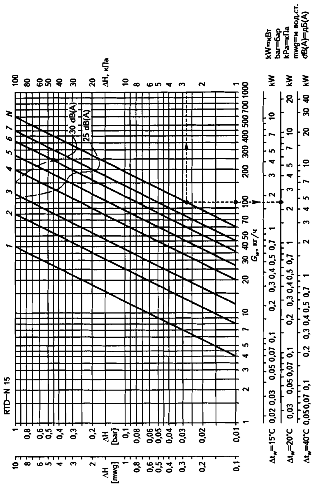
Рис. 4.19. Регулировочный график для настройки терморегулятора RTD-N 15
