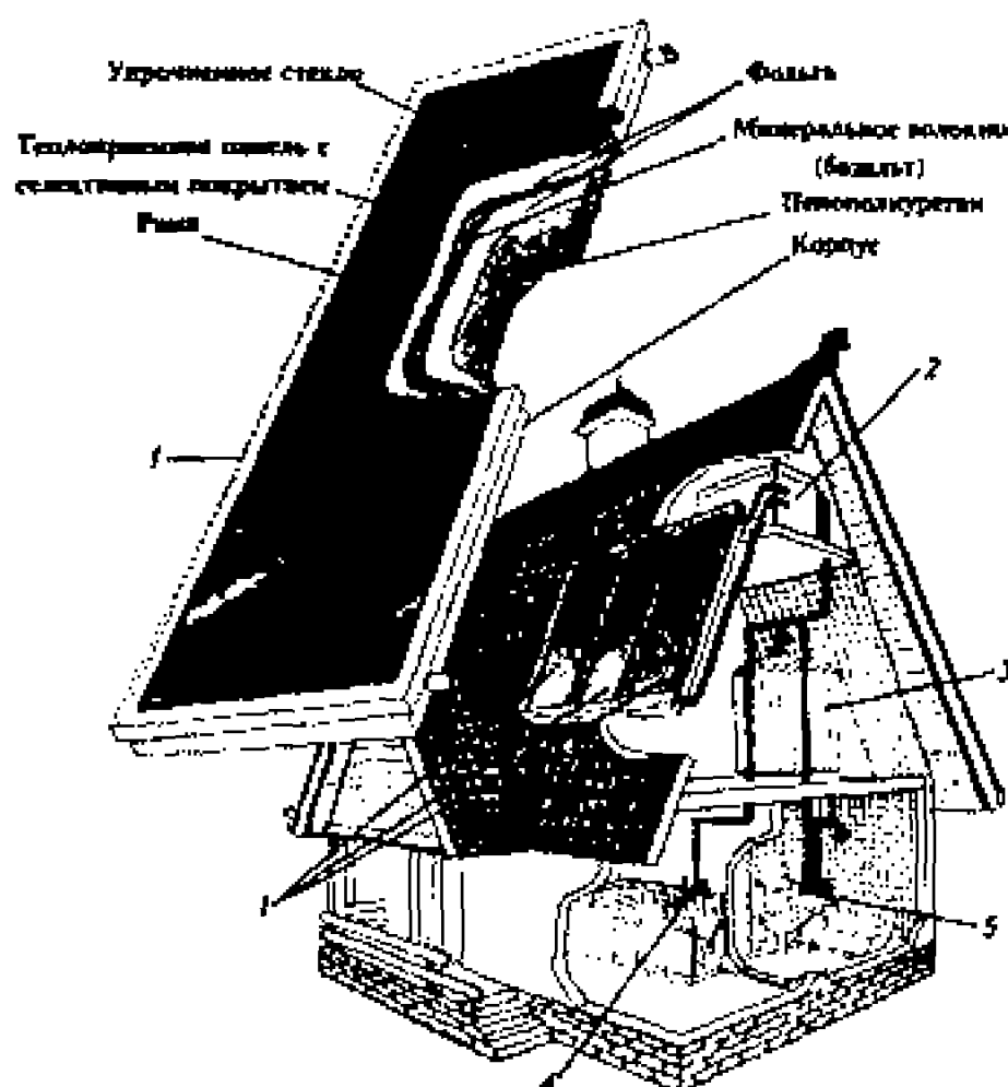
Рис. 8.6. Пример применения установки горячего водоснабжения от солнечной энергии на базе отечественного оборудования
