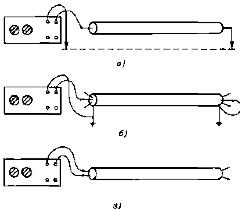
Рис. 10.18. Схемы подключения генератора при поиске отключенного кабеля
