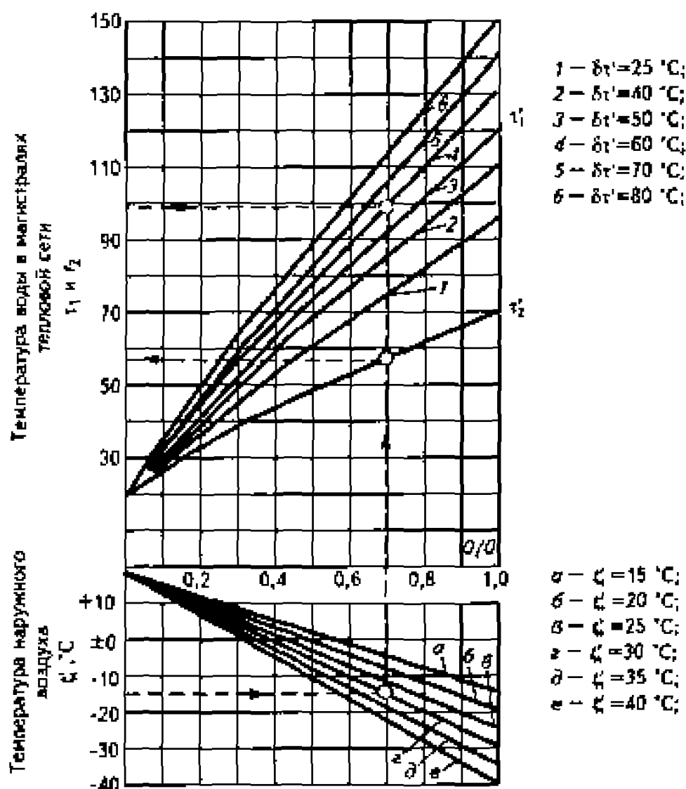
Рис. 10.7. График температуры воды в подающих и обратных магистралях тепловой сети при качественном регулировании отопительной нагрузки при T_{\text{нар}} = +18 ^\circ\text{C}
