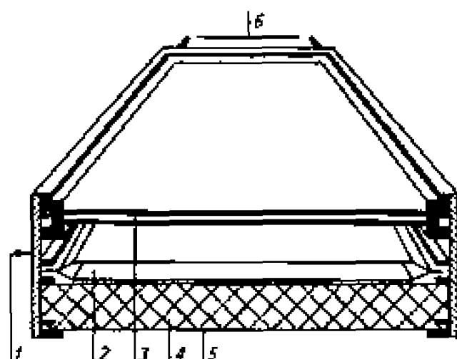
Рис. 8.5. Конструктивная схема солнечного водонагревателя – коллектора 1 – корпус из алюминиевых профилей; 2 – теплоприемная панель; 3 – рама с упрочненными стеклами; 4 – теплоизоляция; 5 – нижняя защитная стенка; 6 – патрубки для присоединения трубопроводов циркуляции воды
