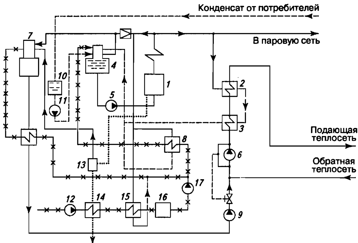
Рис. 6.7. Принципиальная тепловая схема паровой промышленной котельной 1 – паровой котел низкого давления; 2 – пароводяной подогреватель сетевой воды второй ступени; 3 – пароводяной подогреватель сетевой воды первой ступени (охладитель конденсата); 4 – термический деаэратор питательной воды котла; 5 – питательный насос котла; 6 – сетевой насос; 7 – вакуумный деаэратор подпиточной сетевой воды; 8 – подогреватели химически очищенной воды; 9 – подпиточный насос теплосети с регулятором подпитки; 10 – бак для сбора конденсата; 11 – конденсатный насос; 12 – повысительный насос водопроводной воды; 13 – сепаратор продувочной воды котлов; 14 – охладитель продувочной воды котлов; 15 – пароводяной подогреватель водопроводной воды; 16 – оборудование химводоподготовки; 17 – насос умягченной химически очищенной воды
