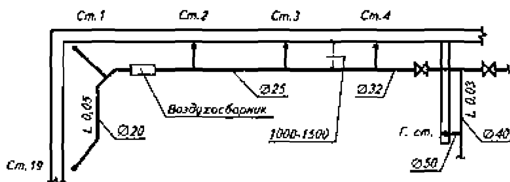
Рис. 9.4. Система с верхней разводкой с размещением распределительных магистральных трубопроводов к вертикальным стоякам на техническом этаже здания
