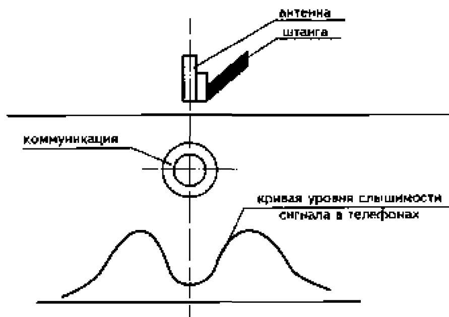
Рис. 10.15. Схема поиска коммуникации по минимуму звукового сигнала
