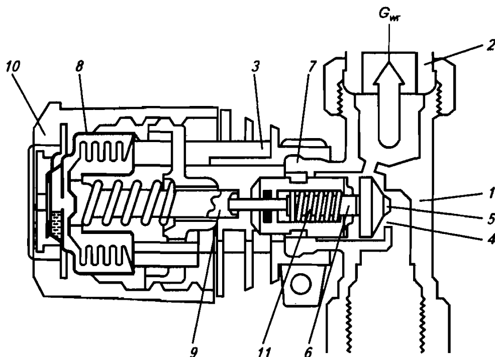
Рис. 3.10. Конструктивная схема терморегулятора
