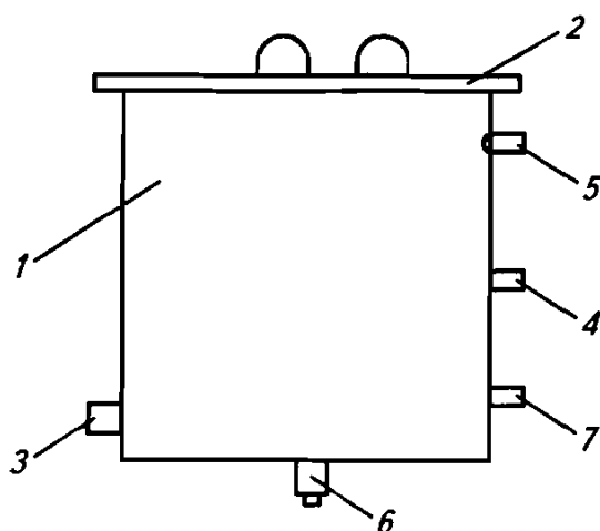
Рис. 4.12. Конструктивное решение расширительного бака
