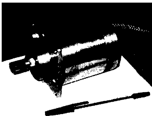
Рис. 6.12. Роторно-лопастной пневмомотор мощностью на 650 Вт при перепаде давления в 4,5 кгс/см 2 ; на 2 кВт при перепаде давления в 10 кгс/см 2 . Размер его сопоставим с шариковой ручкой
