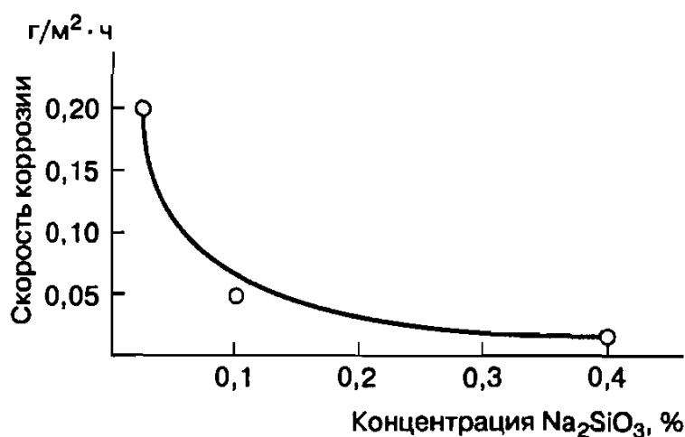
Рис. 6.48. Зависимость скорости коррозии стали в нейтральных водных растворах от концентрации \text{Na}_2\text{SiO}_3
