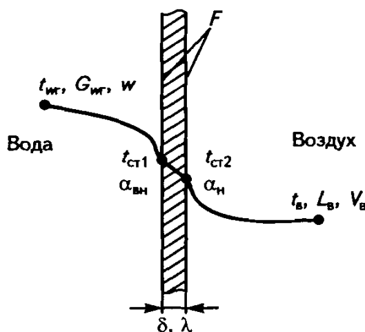
Рис. 1.5. Схема конвективного теплообмена «вода–воздух»
