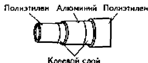
Рис. 9.11. Структура металлополимерной трубы
