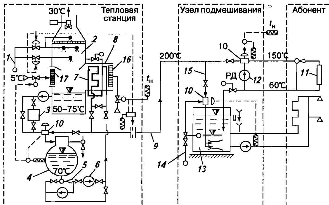
Рис. 6.13. Технологическая схема установки однострубно-го (200 °С) теплоснабжения на базе водотрубно-скрубберного котла ВКВ-6 1 – питательная водопроводная вода; 2 – скруббер котла; 3 – оборудование водоумягчения; 4 – вакуумный деаэратор; 5 – подпорный элеватор; 6 – сетевой насос; 7 – перегревающий трубный пучок; 8 – топка котла; 9 – однострубая тепловая сеть; 10 – смесительное устройство; 11 – система отопления потребителей; 12 – подмешивающий насос; 13 – бак-аккумулятор горячей воды; 14 – водопроводная вода; 15 – подмес сетевой воды; 16 и 17 – газовые горелки зимнего и летнего режимов
