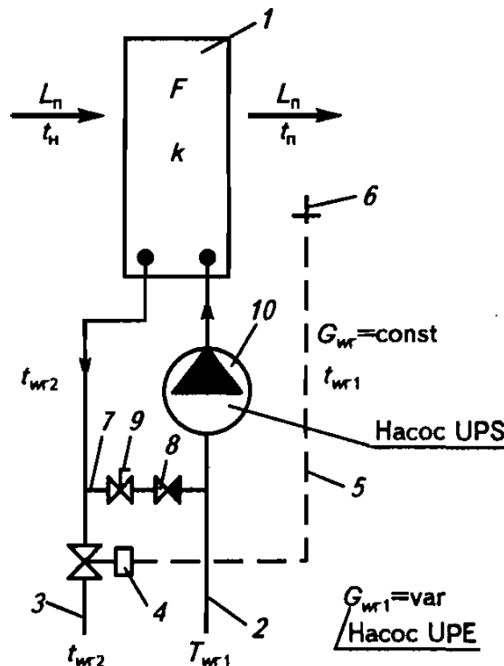
Рис. 3.15. Принципиальная схема качественного регулирования калорифера в системе воздушного отопления
