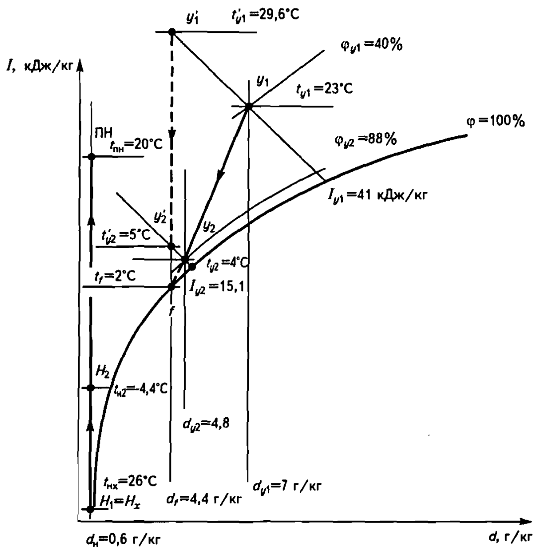
Рис. 3.8. Построение на I - d -диаграмме состояния влажного воздуха режимов последовательного нагрева приточного наружного воздуха в установке утилизации теплоты вытяжного воздуха и в калорифере, питаемом горячей водой H_1 - H_2 - нагрев приточного наружного воздуха теплотой, извлеченной из вытяжного воздуха; y_1 - y_2 - условно «сухой» режим охлаждения удаляемого вытяжного воздуха; H_2 - ПН - нагрев приточного наружного воздуха в калорифере, питаемом горячей водой
