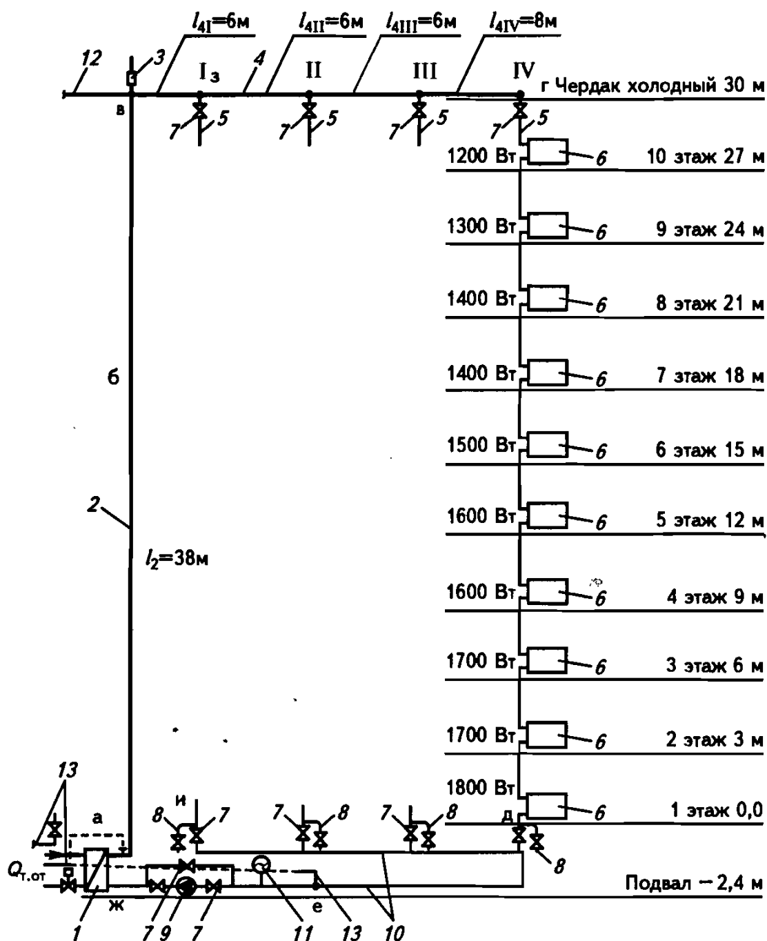
Рис. 4.26. Кольцо циркуляции горячей воды в однотрубной системе отопления с проточными вертикальными стояками и установкой в помещениях конвекторов «Сантехпром» с воздушным регулированием тепловой производительности 1 – пластинчатый водонагреватель; 2 – изолированный вертикальный магистральный трубопровод (главный стояк); 3 – воздухоотводчик; 4 – подающий горизонтальный изолированный магистральный трубопровод; 5 – вертикальный стояк; 6 – конвектор; 7 – краны запорные; 8 – сливные краны из стояков; 9 – циркуляционный насос; 10 – горизонтальный обратный магистральный трубопровод с попутным движением воды; 11 – герметичный расширительный бак; 12 – подающий горизонтальный изолированный магистральный трубопровод к левой части системы отопления (одинаковый с правой); 13 – горизонтальный обратный магистральный трубопровод от левой части системы отопления (одинаковый с правой)
