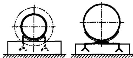
Низкие скользящие опоры: а – направленная; б – свободная
