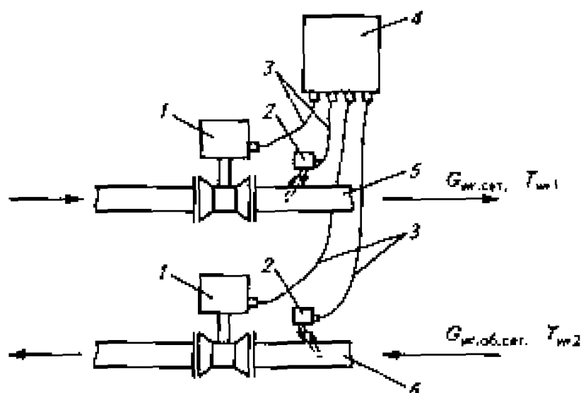
Рис. 7.2. Принципиальная схема установки счетчика расхода теплоты в ЦТП здания
