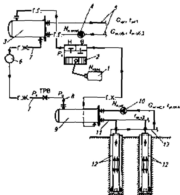
Рис. 8.2. Принципиальная схема теплового насоса при использовании в качестве источника низкопотенциальной теплоты грунта с применением грунтовых теплообменников типа «труба в трубе»
