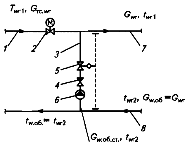
Рис. 4.21. Принципиальная схема включения смесительного насоса (на перемычке) в системе отопления
