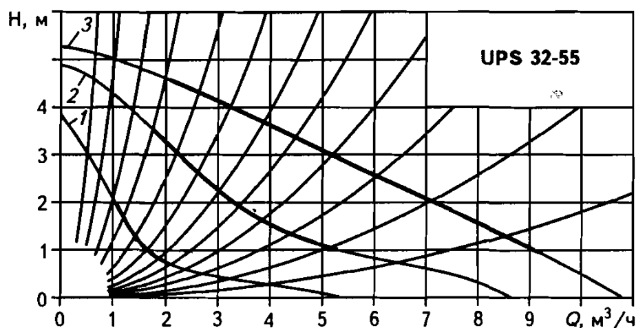
Рис. 4.3. Рабочие характеристики насоса UPS 32-55 при ручном управлении на три скорости вращения рабочего колеса 1 — для малой частоты вращения рабочего колеса при потреблении 0,09 кВт·ч электроэнергии; 2 — для средней частоты вращения рабочего колеса при потреблении 0,13 кВт·ч электроэнергии; 3 — для максимальной частоты вращения рабочего колеса при потреблении 0,14 кВт·ч электроэнергии
