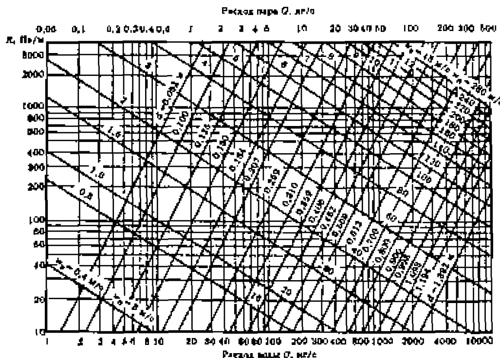
Рис. 10.9. Номограмма для гидравлического расчета трубопроводов
