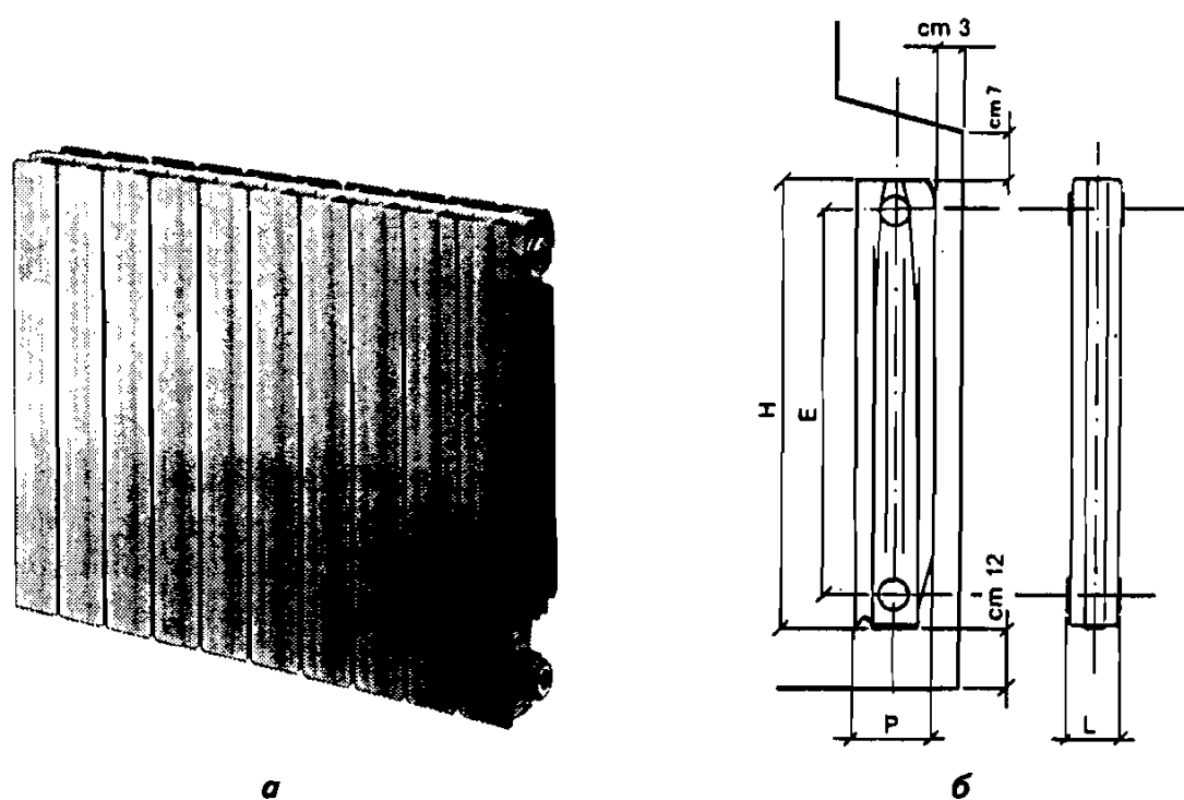
Рис. 3.3. Алюминиевый секционный радиатор ( а ) и рекомендуемые размеры его установки у строительных конструкций в помещении ( б )
