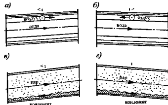
Рис. 5.6. Направление движения теплоносителя и уклона труб в системах отопления. а и б — рекомендуемые и допустимые для водяных магистралей верхней разводки; в и г — рекомендуемые и допустимые для паропроводов
