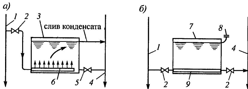
Рис. 9.14. Отопительные приборы децентрализованной пароводяной системы отопления: а - стандартный чугунный радиатор; б - стальной безнапорный радиатор; 1 - паровой стояк; 2 - паровой вентиль; 3 - конденсатный стояк; 4 - вентиль (нормально закрыт); 5 - перфорированная труба; 6 - водоналивной патрубкок; 7 - водонагревательная труба
