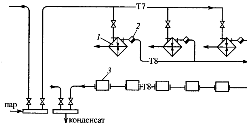
Рис. 9.13. Схема системы парового отопления высокого давления с использованием пароконденсатной смеси в местных отопительных приборах: 1 — калорифер воздушно-отопительного агрегата; 2 — конденсатоотводчик; 3 — местный отопительный прибор
