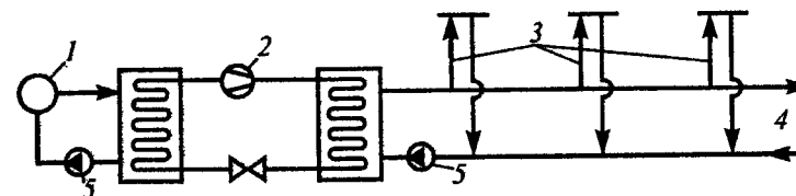
Рис. 20.12. Схема геотермальной теплосети с централизованным повышением температуры теплоносителя с помощью теплового насоса и закачкой отработанной воды в пласт: 1 - скважина; 2 - тепловой насос; 3 - потребители теплоты; 4 - геотермальная теплосеть; 5 - циркуляционные насосы
