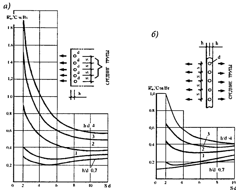
Рис. 4.15. Изменение термического сопротивления массива бетона R'_m , отнесенного к 1 м средних труб бетонного панельного радиатора: а - при односторонней теплоотдаче; б - при двусторонней теплоотдаче; теплопроводность бетона \lambda=1,0 Вт/(м·°C)
