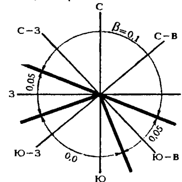
Рис. 2.1. Схема распределения добавок к основным теплопотерям на ориентацию наружных ограждений по странам света (сторонам горизонта)
