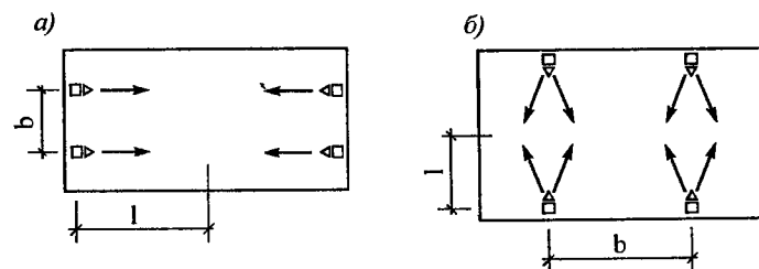
Рис. 10.6. Схема расположения отопительных агрегатов в плане помещения: а - при параллельных воздушных струях; б - при неполных веерных воздушных струях
