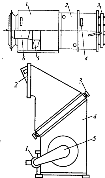
Рис. 10.3. Подвесной воздушно-рециркуляционный отопительный агрегат: 1 - корпус; 2 - воздушонагреватель; 3 - воздушный клапан; 4 - кронштейны; 5 - осевой вентилятор; 6 - электродвигатель
