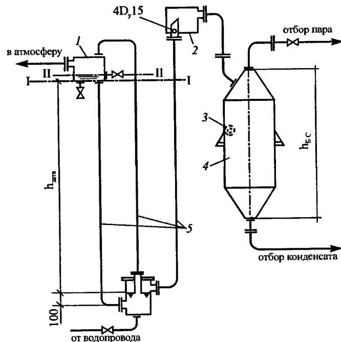
Рис. 9.10. Бак-сепаратор с гидравлическим затвором: 1 - бак возврата воды в затвор; 2 - бак защиты затвора от разрядки; 3 - поступление конденсата; 4 - бак-сепаратор; 5 - гидравлический затвор; I-I - уровень воды в затворе при его заполнении; II-II - то же при давлении пара
