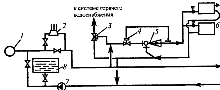
Рис. 20.11. Бессливная комбинированная геотермальная система теплоснабжения с "пиковым" догревом: 1 - скважина; 2 - дополнительный теплоисточник; 3 - смешительный вентиль; 4 - регулятор температуры; 5 - водоструйный элеватор; 6 - отопительные приборы; 7 - циркуляционный насос; 8 - бак-аккумулятор отработанной воды
