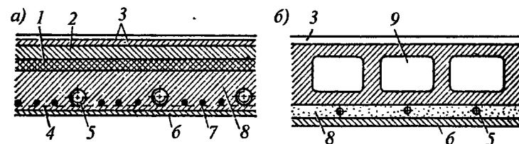
Рис. 11.5. Совмещенные потолочные бетонные панели: а - с расположением греющих труб в несущем бетонном слое; б - то же под несущими пустотелыми блоками; 1 - теплоизоляция; 2 - цементная стяжка; 3 - покрытие пола; 4 - сетка; 5 - греющая труба; 6 - штукатурка; 7 - арматура; 8 - бетонный слой; 9 - пустотелая панель перекрытия
