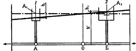
Рис. 7.14. Эпюра гидростатического давления в системе водяного отопления с двумя открытыми расширительными баками, последовательно присоединенными к теплопроводам: О - точка постоянного давления; A_1, A_2 - площадь поперечного сечения соответственно баков 1 и 2; h_1, h_2 - понижение и повышение уровня воды соответственно в баках 1 и 2
