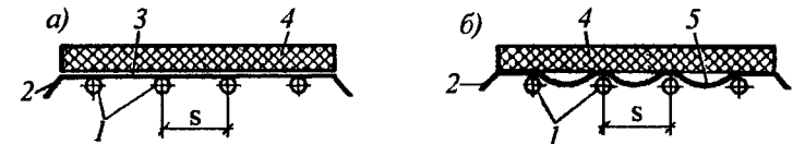
Рис. 11.3. Подвесная металлическая отопительная панель: а - с плоским экраном; б - с экраном волнообразной формы; 1 - греющие трубы; 2 - козырек; 3 - плоский экран; 4 - теплоизоляция; 5 - волнообразный экран
