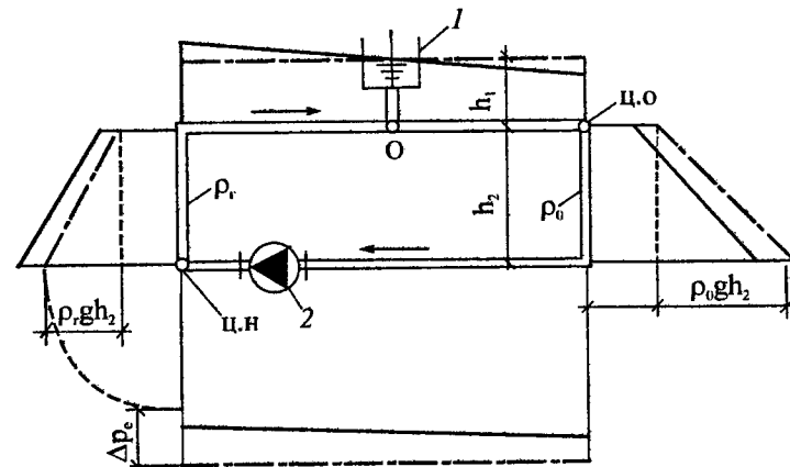
Рис. 7.5. Эпюра гидростатического давления в системе отопления с нагреваемой водой при бездействии циркуляционного насоса: 1 - открытый расширительный бак; 2 - циркуляционный насос; ц.н - центр нагревания; ц.о - центр охлаждения; О - точка постоянного давления
