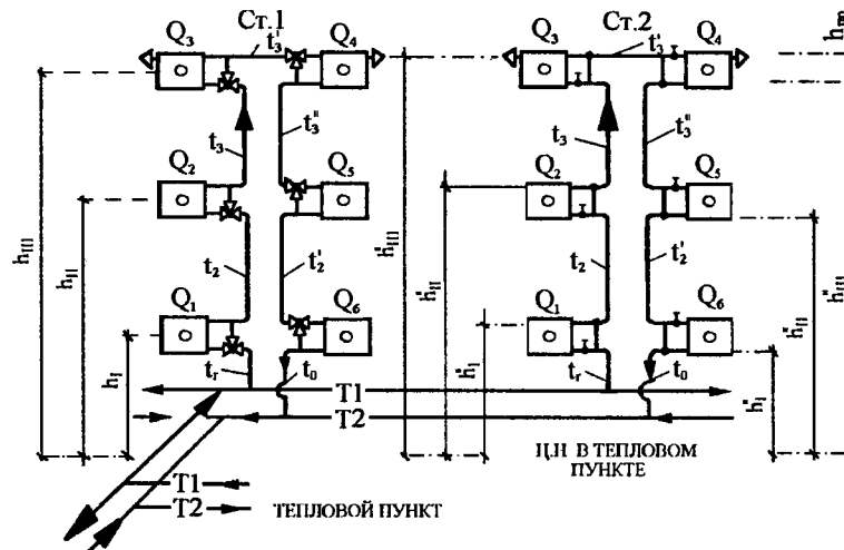
Рис. 7.21. Расчетная схема вертикальной однотрубной системы водяного отопления с нижней разводкой обеих магистралей (с П-образными стояками): Ст.1 - проточно-регулируемый стояк; Ст.2 - стояк с замыкающими участками
