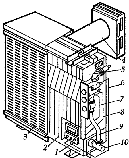
Рис. 13.4. Газовый отопительный камин конвективного действия: 1 - запальное устройство; 2 - камера сгорания; 3 - облицовка; 4 - стенной канал; 5 - экран; 6 - термопара; 7 - провод пьезоэлектрического запального устройства; 8 - трубка запальника; 9 - газопровод; 10 - горелка
