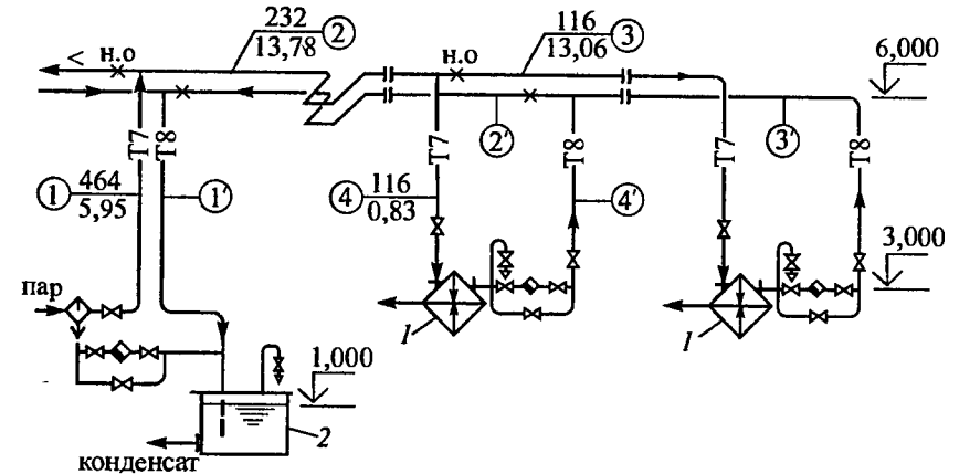
Рис. 9.12. Расчетная схема разомкнутой системы парового отопления высокого давления с закрытым конденсатным баком: 1 - калорифер воздушно-отопительного агрегата; 2 - конденсатный бак
