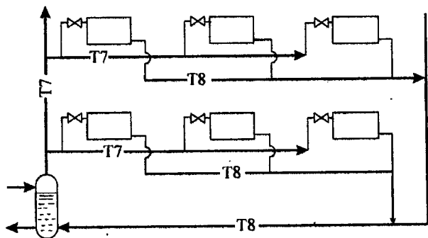
Рис. 20.4. Горизонтальная двухтрубная низкотемпературная система парового отопления
