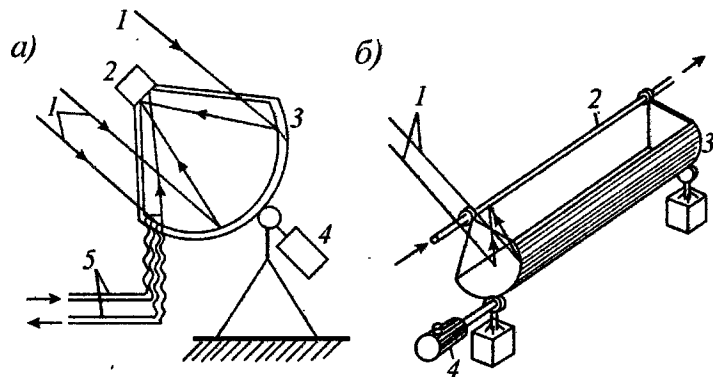
Рис. 20.6. Концентрирующие гелиоприемники: а - параболический концентратор; б - параболическоцилиндрический концентратор; 1 - солнечные лучи; 2 - тепловоспринимающий элемент (солнечный котел); 3 - зеркало; 4 - механизм привода системы слежения; 5 - теплопроводы, подводящие и отводящие теплоноситель
