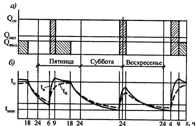
Рис. 19.6. Изменение теплового и температурного режимов рабочего помещения в течение четырех дней недели в зимнее время: а - изменение теплопоступлений; б - изменение температурных параметров
