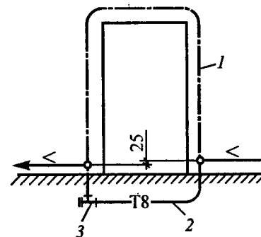
Рис. 9.4. Обвод сухим конденсатопроводом дверного проема: 1 - воздушная труба; 2 - изолированная труба в подпольном канале; 3 - тройник с пробкой
