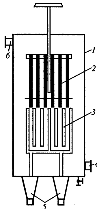
Рис. 14.15. Электродкотел: 1 - корпус; 2 - пакет диэлектрических пластин; 3 - пакет электродов; 4 - патрубок для входа нагреваемой воды; 5 - вводы электропитания; 6 - патрубок для выхода нагретой воды
