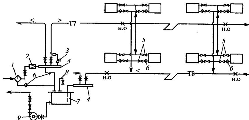
Рис. 9.5. Разомкнутая система парового отопления высокого давления со средней разводкой: 1 - водоотделитель; 2 - редукционный клапан; 3 - предохранительный клапан; 4 - коллектор; 5 - паровой вентиль; 6 - конденсатоотводчик; 7 - конденсатный бак; 8 - воздушная труба; 9 - конденсатный насос; н.о. - неподвижная опора
