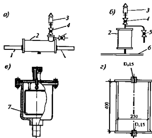
Рис. 5.23. Схемы установок воздухоотборников и воздухоотводчиков: а - с горизонтальным проточным воздухоотборником; б - с вертикальным непроточным воздухоотборником; в - автоматический воздухоотводчик; з - непроточный воздухоотборник; 1 - верхняя магистраль; 2 - воздухоотборник; 3 - автоматический воздухоотводчик; 4 - запорный кран; 5 - ручной воздухоотводчик; 6 - воздушная линия; 7 - поплавок
