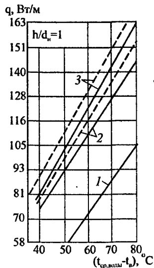
Рис. 11.4. Теплоотдача 1 м одиночной трубы D_n 15-20 ; 1 - открыто проложенная труба; 2 и 3 - труба в бетоне при его теплопроводности, соответственно, 1,05 и 1,28 Вт/(м·°С) (толщина слоя бетона h от оси трубы равна ее наружному диаметру d_n ); сплошные и пунктирные линии - соответственно, при односторонней и двухсторонней теплоотдаче
