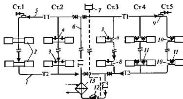
Рис. 6.1. Схема вертикальной одноконтурной системы водяного отопления с верхней разводкой подающей магистрали: Ст.1 — проточный стояк; Ст.2 и Ст.3 — стояки соответственно с осевыми и смещенными замыкающими участками; Ст.4 и Ст.5 — проточно-регулируемые стояки; 1 — обратная магистраль (Т2); 2 — отопительные приборы; 3 — краны типа КРП; 4 — осевой замыкающий участок; 5 — подающая магистраль (Т1); 6 — главный стояк (Г.ст.); 7 — открытый расширительный бак; 8 — смещенный замыкающий участок; 9 — проточный воздухооборник; 10 — обходной участок; 11 — краны типа КРТ; 12 — циркуляционный насос; 13 — теплообменник
