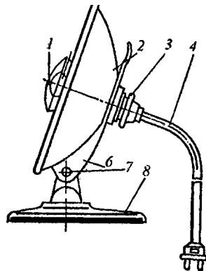
Рис. 14.4. Электрокамин со сферическим отражателем: 1 - декоративная защитная решетка; 2 - нагревательный элемент; 3 - отражатель; 4 - патрон; 5 - шнур электропитания; 6 - кронштейн; 7 - поворотный винт; 8 - подставка
