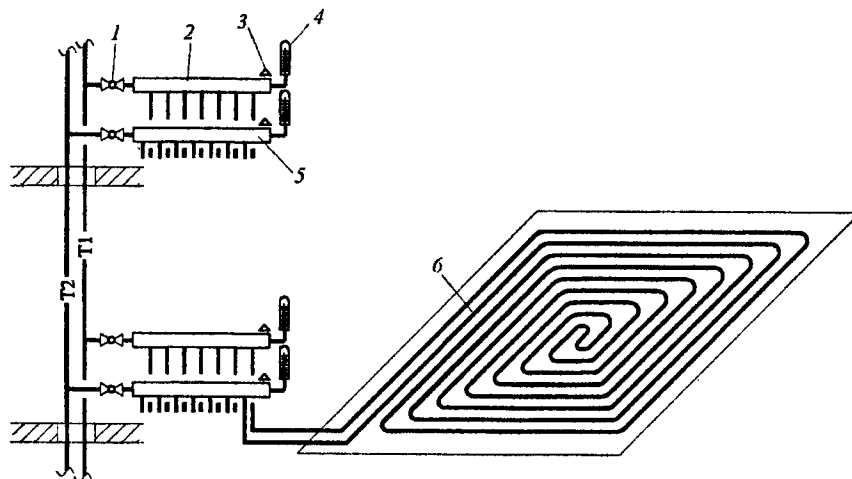
Рис. 11.12. Коллекторная схема системы напольного водяного отопления: 1 - запорная арматура; 2 - распределительный коллектор; 3 - воздухоотводчик; 4 - термометр; 5 - сборный коллектор; 6 - греющие трубы
