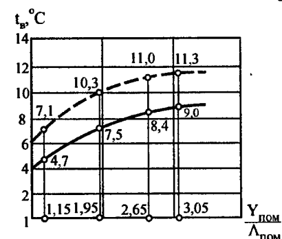
Рис. 19.7. Зависимость минимальной температуры воздуха после ночного охлаждения (без отопления) от теплоустойчивости помещений, имеющих окна с двойным (сплошная линия) и тройным (пунктирная линия) остеклением, при t_{\text{н}} = -20^\circ\text{C}
