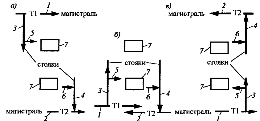
Рис. 5.1. Теплопроводы вертикальных систем центрального отопления: а - с верхней разводкой подающей магистрали; б - с нижней разводкой обеих магистралей; в - с "опрокинутой" циркуляцией; 1 и 2 - подающие (Т1) и обратные (Т2) магистрали; 3 и 4 - подающие и обратные стояки; 5 и 6 - подающие и обратные подводки; 7 - отопительные приборы (стрелками показано направление движения теплоносителя)
