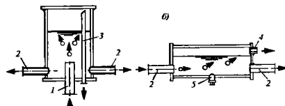
Рис. 5.22. Проточные воздухоборники: а - вертикальный на главном стояке; б - горизонтальный на верхней магистрали; 1 - главный стояк, 2 - магистрали, 3 - труба D_{15} (с краном) для выпуска воздуха; 4 - муфта D_{15} для воздухоотпускной трубы; 5 - муфта D_{15} с пробкой для удаления грязи
