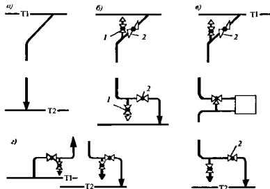
Рис. 5.4. Схемы присоединения стояков к магистралям систем водяного отопления различной этажности: а - двух-трехэтажных; б - четырех-семизэтажных при верхней разводке; в - той же при нижней разводке; г - восьмизэтажных и более высоких; 1 - спусковой кран (проходной или шаровый, внизу - со штуцером для подключения водоотводящего шланга); 2 - запорный (проходной или шаровый) кран
