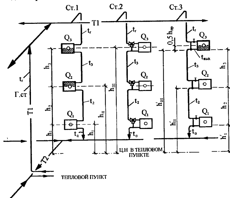
Рис. 7.20. Расчетная схема вертикальной однострубной системы водяного отопления с верхней разводкой: Ст.1 - проточный стояк; Ст.2 - проточно-регулируемый стояк; Ст.3 - стояк с замыкающими участками; кружки в контуре отопительных приборов - центры охлаждения воды в приборах; жирные точки на стояке 3 - центры охлаждения воды в стояке
