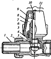
Рис. 5.12. Кран двойной регулировки типа "Термис": 1 – патрубок с наружной резьбой; 2 – соединительная гайка; 3 – клапан; 4 – корпус; 5 – гайка крышки; 6 – сальниковая набивка; 7 – крышка; 8 – гайка уплотнителя шпильки; 9 – шпилька; 10 – винт; 11 – муфта
