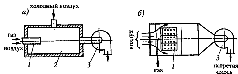
Рис. 13.6. Принципиальные схемы смесительных газовоздушных теплообменников: а - с разбавлением продуктов сгорания в специальной камере; б - со сжиганием газа непосредственно в потоке воздуха; 1 - блок газовых горелок; 2 - камера смешения; 3 - радиальный вентилятор
