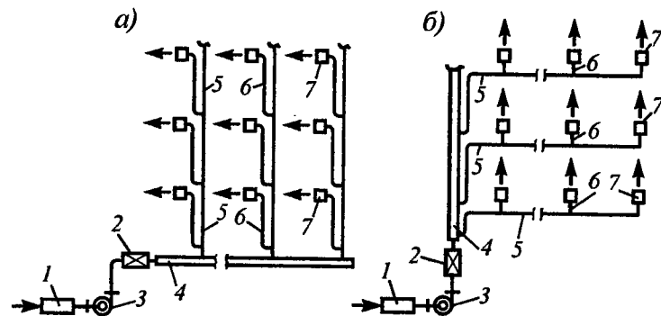
Рис. 18.2. Схемы высокоскоростных систем комбинированного воздушного отопления с доводчиками многоэтажных зданий: а - вертикальная система; б - горизонтальная система; 1 - центральный агрегат для подготовки воздуха; 2 - шумоглушитель; 3 - вентилятор; 4 - магистральный воздуховод; 5 - распределительный воздуховод; 6 - ответвление; 7 - доводчик
