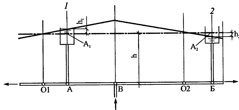
Рис. 7.16. Эпюра гидростатического давления в системе водяного отопления с двумя открытыми расширительными баками, параллельно присоединенными к теплопроводам: О1, О2 - точки постоянного давления; А1, А2 - площадь поперечного сечения соответственно баков 1 и 2; h_1 , h_2 - понижение и повышение уровня воды соответственно в баках 1 и 2
