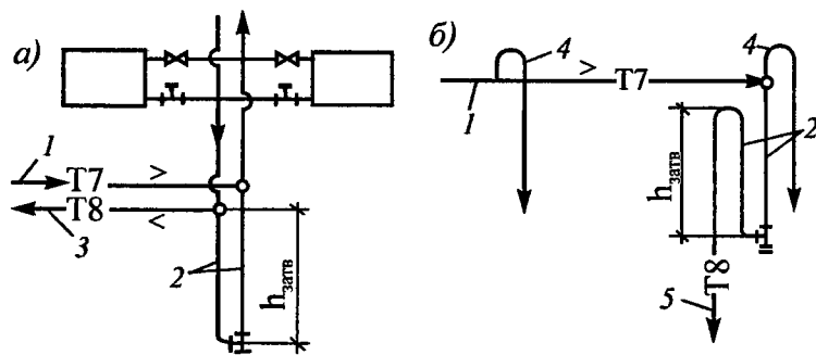
Рис. 9.3. Схема системы осушки пара : а - при нижней разводке паропроводов; б - при верхней разводке паропроводов; 1 - паропровод; 2 - гидравлический затвор; 3 - конденсатопровод; 4 - калач; 5 - конденсатный стояк
