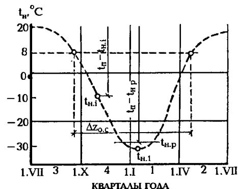
Рис. 1.2. Изменение среднесуточной температуры наружного воздуха в течение года в Москве: t_n – температура помещения; t_{н.1} – минимальная среднесуточная температура наружного воздуха
