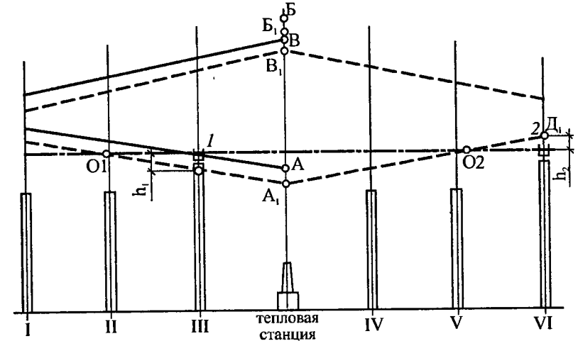
Рис. 7.17. Изменение гидростатического давления в теплопроводах районной системы теплоснабжения при ее расширении с установкой второго расширительного бака: 1 и 2 — соответственно существующий и дополнительный расширительные баки; О1 и О2 — новые точки постоянного давления
