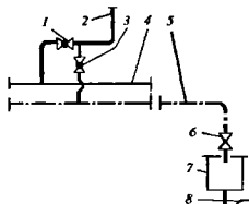
Рис. 5.20. Схема дренажа стояков систем водяного отопления. 1 - запорный кран; 2 - стояк; 3 - спускной кран; 4 - магистраль; 5 - дренажная линия; 6 - общий запорный вентиль; 7 - открытый перепускной бачок; 8 - выпуск через сифон в водосток
