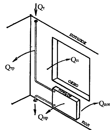
Рис. 4.1. Схема теплоотдачи отопительного прибора Q_{пр} и труб Q_{тр} для возмещения теплопотерь помещения Q_n и дополнительных теплопотерь Q_{доп} при теплоподаче со стороны теплоносителя Q_T
