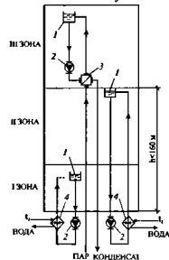
Рис. 6.9. Схема водяного отопления высотного здания: I и II - зоны здания с водо-водяным отоплением; III - зона здания с пароводяным отоплением; 1 - расширительный бак; 2 - циркуляционный насос; 3 - пароводяной теплообменник; 4 - водо-водяный теплообменник
