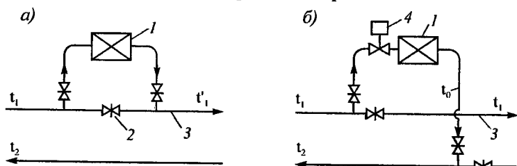
Рис. 10.10. Схемы присоединения воздушонагревателя к теплопроводам: а - последовательная схема; б - параллельная схема; 1 - воздушонагреватель; 2 - нормально закрытая задвижка на обводной трубе; 3 - подающая магистраль основной системы отопления; 4 - регулятор расхода воды
