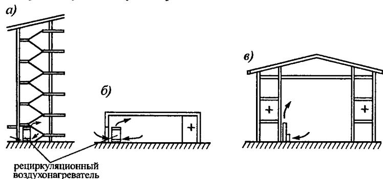
Рис. 10.8. Применение рециркуляционного воздушонагревателя для отопления: а - лестничной клетки в многоэтажном здании; б - низкого помещения; в - высокого помещения
