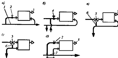
Рис. 5.10. Присоединение труб к отопительным приборам систем водяного отопления: а - к горизонтальной однотрубной с замыкающим участком ветви; б и в - к верхним приборам в стояках с нижним расположением обеих магистралей (с нижней разводкой) соответственно двухтрубной и однотрубной проточно-регулируемой; г и д - при деаэрированной воде соответственно в однотрубном проточно-регулируемом стояке (верхние приборы) и горизонтальной однотрубной с замыкающими участками ветви; 1 - осевой замыкающий участок; 2 - кран типа КРП; 3 - воздушный кран; 4 - кран типа КРД; 5 - кран типа КРТ; 6 - смешанный обходной участок; 7 - редуцирующая вставка
