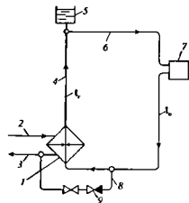
Рис. 6.7. Схема гравитационной системы водяного отопления: 1 - теплообменник (или теплогенератор - водогрейный котел); 2 и 3 - наружные, соответственно, подающий и обратный теплопроводы; 4 - главный стояк; 5 - открытый расширительный бак; 6 - подающая магистраль; 7 - отопительный прибор; 8 - наполнительно-подпиточная труба; 9 - обратный клапан
