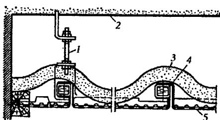
Рис. 11.6. Подвесная потолочная отопительная панель: 1 - подвеска; 2 - перекрытие; 3 - теплоизоляция; 4 - труба для теплоносителя; 5 - перфорированный металлический лист
