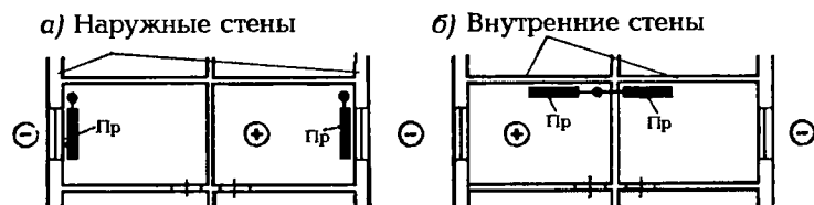
Рис. 4.8. Размещение отопительных приборов в помещениях (в плане): а - под окнами; б - у внутренних стен; Пр - отопительный прибор
