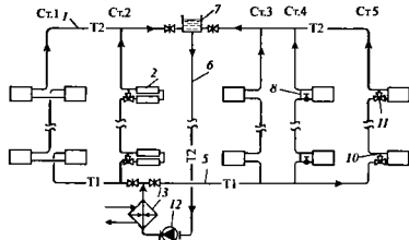
Рис. 6.3. Схема вертикальной однотрубной системы водяного отопления с "опрокинутой" циркуляцией воды и проточным открытым расширительным баком: Ст.1 - проточный стояк с конвекторами с кожухом; Ст.2 и Ст.5 - проточно-регулируемые стояки соответственно с конвекторами без кожуха и радиаторами; Ст.3 - проточный стояк с радиаторами; Ст.4 - стояк со смещенными к радиаторам замыкающими участками; обозначения 1-13 - см. рис. 6.1
