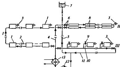
Рис. 6.5. Схемы горизонтальной однотрубной системы водяного отопления: I - проточная ветвь для приборов, расположенных на разных этажах; II - проточная бифидная ветвь; III - ветвь с замыкающими участками; 1 - радиаторы; 2 - воздушная труба; 3 - воздушные краны; 4 - подающий стояк; 5 - обратный стояк; 6 - запорно-регулирующая арматура; 7 - открытый расширительный бак; 8 - конвекторы двухтрубные; 9 - краны типа КРП; 10 - осевая замыкающая вставка; 11 - обратная магистраль; 12 - циркуляционный насос; 13 - теплообменник
