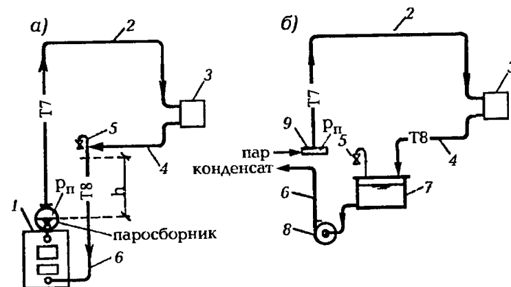
Рис. 1.6. Схемы системы парового отопления: а – замкнутая схема; 1 – паровой котел с паросборником; 2 – паропровод (Т7); 3 – отопительный прибор; 4 и 6 – самотечный и напорный конденсатопроводы (Т8); 5 – воздушовыпускная труба; 7 – конденсатный бак; 8 – конденсатный насос; 9 – парораспределительный коллектор
