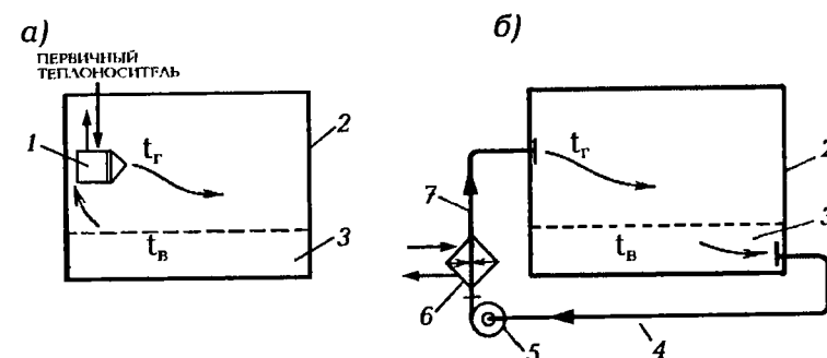
Рис. 1.7. Схемы системы воздушного отопления: а - местная система; б - центральная система; 1 - отопительный агрегат; 2 - обогреваемое помещение (помещения на рис. б); 3 - рабочая (обслуживаемая) зона помещения; 4 - обратный воздуховод; 5 - вентилятор; 6 - теплообменник (калорифер); 7 - подающий воздуховод
