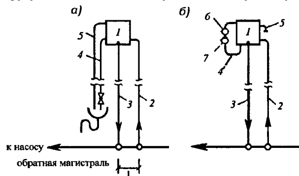
Рис. 3.19. Присоединение открытого расширительного бака к системе отопления: а - с ручным (визуальным) контролем; б - с автоматизированной сигнализацией и регулированием уровня воды в баке; 1 - расширительный бак; 2, 3, 4, 5 - соответственно, расширительная, циркуляционная, контрольная и переливная трубы; 6, 7 - реле, соответственно, верхнего и нижнего уровней воды в баке (соединены с баком трубой 4')
