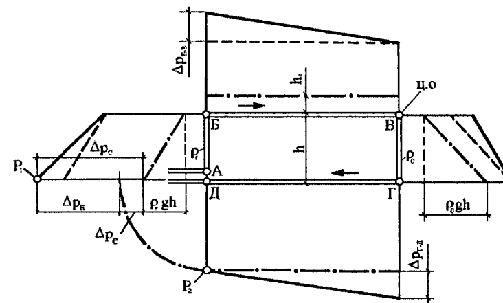
Рис. 7.13. Изменение гидростатического давления в системе водяного отопления, непосредственно присоединенной к наружным теплопроводам (без расширительного бака): Д - точка постоянного давления P_2
