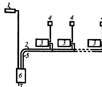
Рис. 14.9. Электротеплоаккумуляционная система отопления одноквартирного дома: 1 - датчик температуры наружного воздуха; 2 - электрокабель; 3 - электротеплоаккумуляционный отопительный прибор; 4 - датчик температуры внутреннего воздуха; 5 - кабель управления; 6 - блок автоматического регулирования; 7 - трехфазный электроввод
