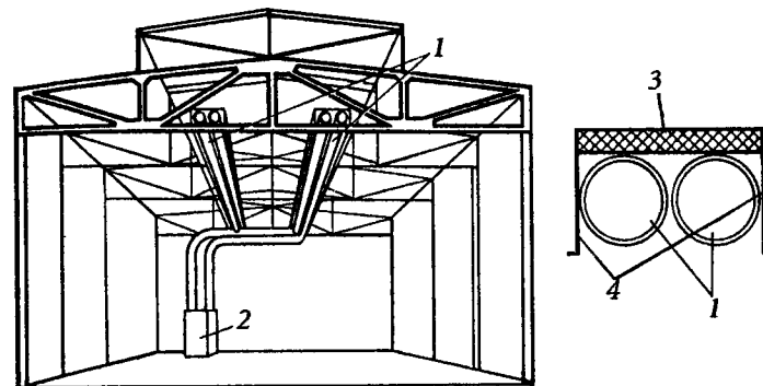
Рис. 13.7. Система газовоздушного отопления с теплоизлучающими трубами в межферменном пространстве цеха: 1 - теплоизлучающие трубы; 2 - теплогенератор; 3 - теплоизоляция; 4 - козырьки
