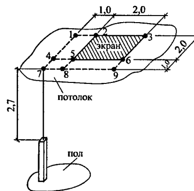
Рис. 11.1. Схема взаимного расположения в помещении человека и потолочного отопительного экрана (к примеру 11.1)
