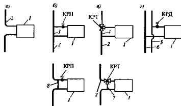
Рис. 5.7. Одностороннее присоединение труб к отопительным приборам вертикальных систем отопления: а, б, в - однотрубная система; г - двухтрубная система; 1 - отопительные приборы; 2 - однотрубные стояки; 3 - осевой замыкающий участок; 4 - осевой обходной участок; 5 и 6 - подающая и обратные трубы двухтрубного стояка; 7 - смещенный обходной участок; 8 - смещенный замыкающий участок
