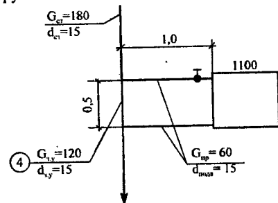
Рис. 8.7. Схема узла малого циркуляционного кольца в стояке с осевыми замыкающими участками вертикальной однетрубной системы водяного отопления с верхней разводкой (к примеру 8.5): 1100 - тепловая нагрузка отопительного прибора, Вт
