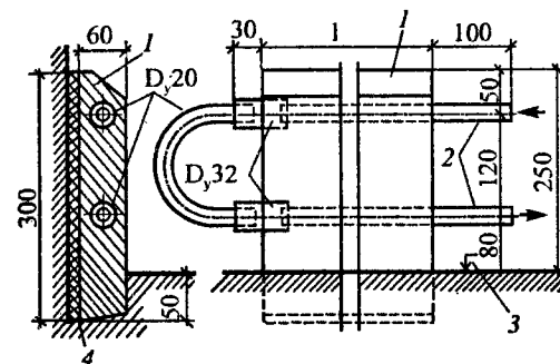
Рис. 11.9. Плинтусная приставная бетонная отопительная панель: 1 - бетон; 2 - концы греющих труб для присоединения к стояку; 3 - поверхность чистого пола; 4 - тепловая изоляция
