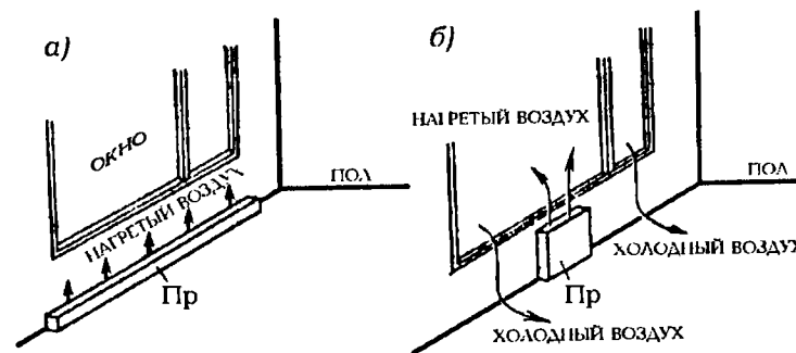
Рис. 4.10. Размещение под окном помещения отопительного прибора: а - низкого и длинного (желательно); б - высокого и короткого (нежелательно); Пр - отопительный прибор
