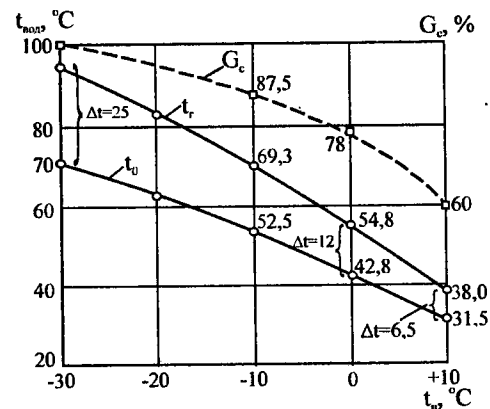
Рис. 7.25. График изменения температуры и расхода воды в вертикальной однотрубной системе отопления в течение отопительного сезона: расчетные значения t_r=95 °C и t_o=70 °C соответствуют t_{н,р}=-30 °C
