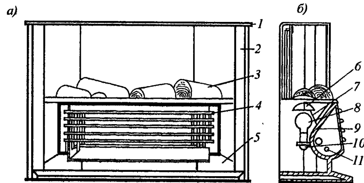
Рис. 14.5. Декоративно-функциональный электрокамин: а - вид спереди; б - вид сбоку; 1 - декоративный внешний корпус; 2 - внутренний металлический корпус; 3 - панель имитации топлива; 4 - декоративно-защитная решетка; 5 - полупрозрачный экран; 6 - вертушка; 7 - кронштейн с иглой; 8 - красная лампа; 9 - отражатель; 10 - патрон; 11 - нагревательные элементы
