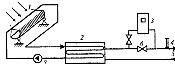
Рис. 20.7. Жидкостная комбинированная двухконтурная низкотемпературная система отопления с параболическоцилиндрическим концентратором и жидкостным теплоаккумулятором: 1 - параболическоцилиндрический концентратор; 2 - жидкостный теплоаккумулятор; 3 - дополнительный теплоисточник; 4 - термометр; 5 - контур системы отопления; 6 - регулирующий вентиль; 7 - циркуляционный насос
