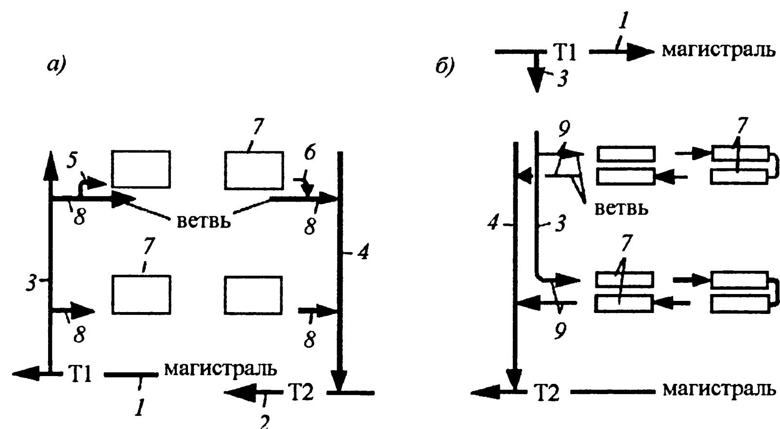
Рис. 5.2. Теплопроводы горизонтальных систем центрального отопления: а - с нижней разводкой обеих магистралей; б - с верхней разводкой подающей магистрали; 1 и 2 - подающие (Т1) и обратные (Т2) магистрали; 3 и 4 - подающие и обратные стояки; 5 и 6 - подающие и обратные подводки; 7 - отопительные приборы; 8 - однотрубные ветви; 9 - бифилярные ветви (стрелками показано направление движения теплоносителя)
