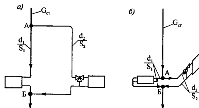
Рис. 8.4. Схемы нетиповых узлов однотрубных стояков: а - с ответвлением к прибору, удаленному от стояка; б - с приборами различного вида; S_1 и S_2 - характеристики сопротивления параллельно соединенных участков между точками А и Б
