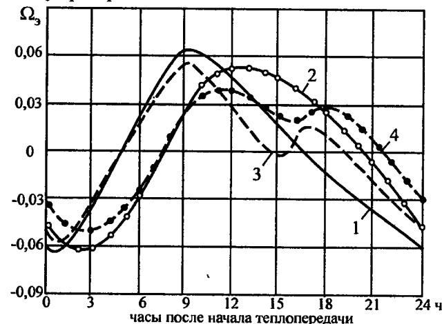
Рис. 14.11. Расчетные значения коэффициента прерывистости теплового потока электроаккумулирующего отопительного прибора: кривые 1, 3 - прибор с показателем затухания тепловой волны 7,9; 2, 4 - то же с показателем 10; 1, 2 - при периоде зарядки прибора 8 ч; 3, 4 - то же при дополнительной 2-часовой подзарядке
