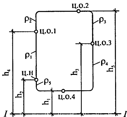
Рис. 7.19. Схема вертикального циркуляционного кольца теплопроводов без отопительных приборов с произвольно расположенными центрами нагревания (ц.н) и охлаждения (ц.о) теплоносителя воды
