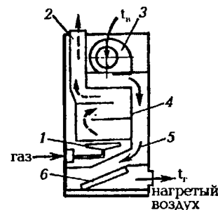
Рис. 1.3. Схема газозудного отопительного агрегата: 1 – газовая горелка; 2 – дымоход; 3 – вентилятор; 4 – газозудный теплообменник; 5 – теплопроводы (каналы); 6 – воздушный фильтр
