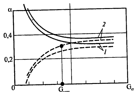
Рис. 8.5. Изменение коэффициента затекания воды в отопительные приборы однострубных стояков: 1 – с осевыми замыкающими участками; 2 – со смещенными замыкающими участками; сплошная линия – движение воды в стояках сверху вниз; пунктирная линия – то же снизу вверх
