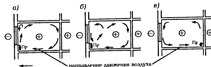
Рис. 4.9. Схема циркуляции воздуха в помещении при различном месте размещения отопительного прибора: а - под окнами без подоконника; б - под окнами с подоконником; в - у внутренней стены; Пр - отопительный прибор
