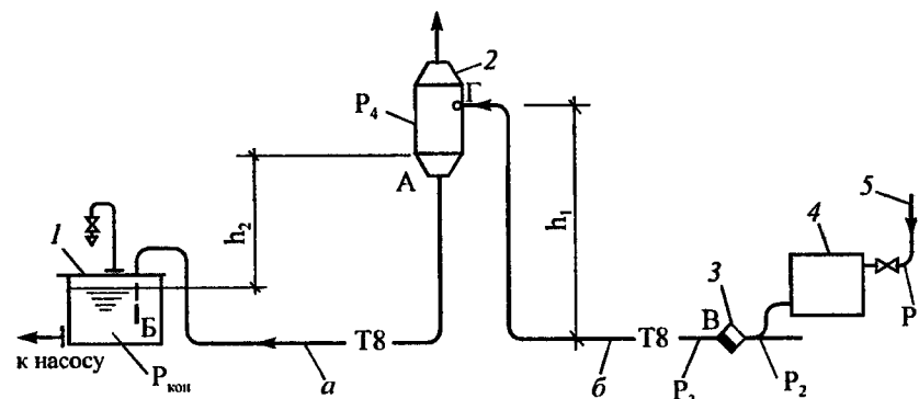
Рис. 9.11. Схема конденсатопроводов: a - напорный; b - двухфазный; 1 - конденсатный бак; 2 - бак-сепаратор; 3 - конденсатоотводчик; 4 - отопительные приборы системы парового отопления высокого давления; 5 - паропровод
