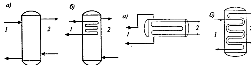
Рис. 20.1. Зависимое включение теплоаккумулятора в контур системы отопления: а - с зависимым подключением греющего контура; б - с независимым подключением греющего контура; 1 - греющий контур; 2 - контур системы отопления
