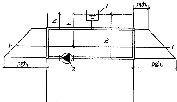
Рис. 7.4. Эпюра гидростатического давления в системе отопления с не нагреваемой водой при бездействии циркуляционного насоса: 1 - открытый расширительный бак; 2 - циркуляционный насос
