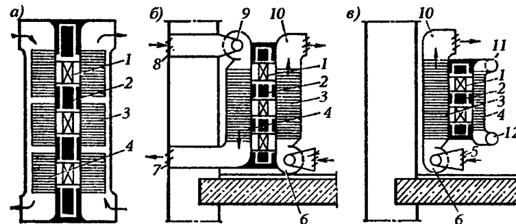
Рис. 14.14. Конструкции тепловых насосов: а - тепловой насос, работающий на полупроводниках; б - насос, действующий по принципу "воздух-воздух"; в - то же по принципу "воздух-вода"; 1 - полупроводник; 2 - тепловая изоляция; 3 - оребрение горячих спаев; 4 - оребрение холодных спаев; 5 - патрубок с решеткой для входа нагретого воздуха; 6 - вентилятор для перемещения внутреннего воздуха; 7, 8 - решетки для входа и выхода наружного воздуха; 9 - вентилятор для перемещения наружного воздуха; 10 - патрубок с решеткой для выхода нагретого воздуха; 11, 12 - патрубки для подачи и отвода низкотемпературной воды
