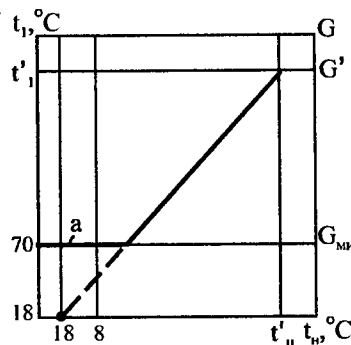
Рис. 17.3. Принцип построения графика регулирования температуры или расхода теплоносителя в системе водяного теплоснабжения в течение отопительного сезона
