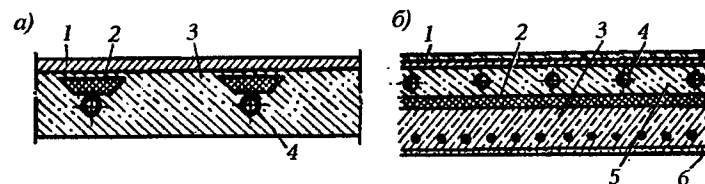
Рис. 11.7. Напольные бетонные отопительные панели: а - с расположением греющих труб в несущей части перекрытия; б - то же на несущем перекрытии; 1 - покрытие пола; 2 - теплоизоляционный материал; 3 - железобетонное несущее перекрытие; 4 - греющая труба; 5 - бетонная панель; 6 - штукатурка
