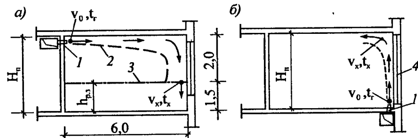
Рис. 10.12. Центральное воздушное отопление помещения : а - с подачей нагретого воздуха через подпотолочный щелевой воздухоораспределитель (к примеру 10.11); б - то же через напольный (к примеру 10.12); 1 - воздухоораспределитель; 2 - граница настилающейся воздушной струи; 3 - граница рабочей зоны; 4 - наружное ограждение
