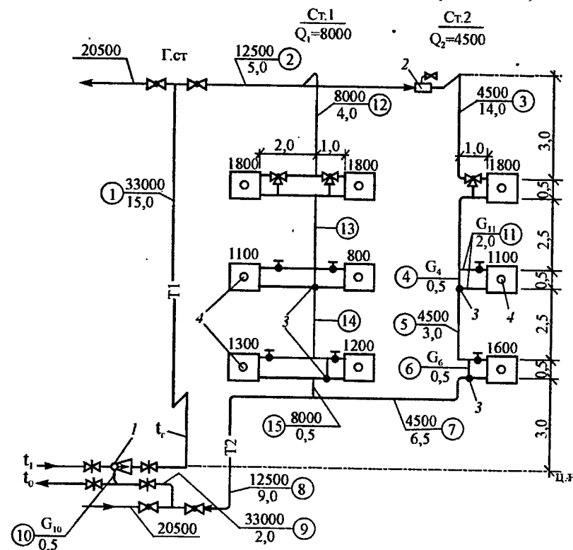
Рис. 8.6. Схема вертикальной однострубной системы водяного отопления с верхней разводкой и тупиковым движением воды в магистралях (к примеру 8.3): 1 – водоструйный элеватор; 2 – воздушник; 3 и 4 – центры охлаждения воды (ц.о.) соответственно в стояках и отопительных приборах; ц.н. – условный центр нагревания воды; цифра над отопительным прибором и под номером стояка – их тепловая нагрузка (Вт)
