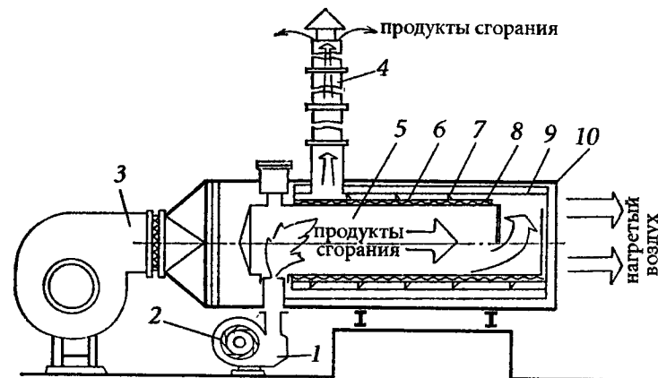
Рис. 13.5. Газовоздушный теплообменник: 1 - газовая горелка; 2 - воздушный патрубок горелки; 3 - радиальный вентилятор; 4 - дымовая труба; 5 - камера сгорания; 6 - кольцевой теплообменник; 7 - винтообразная перегородка; 8 - проволочная сетка; 9 - экран; 10 - наружный кожух
