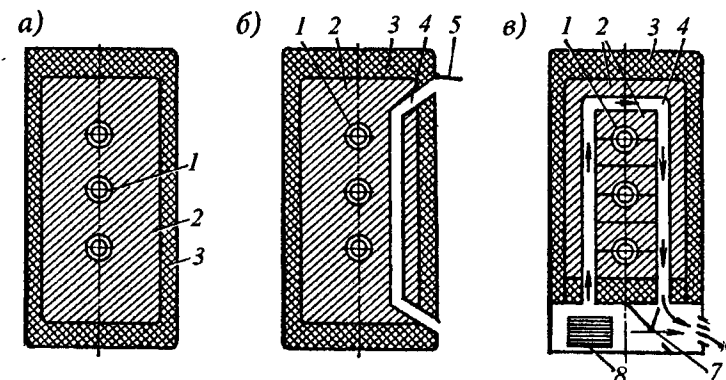
Рис. 14.8. Электрические теплоаккумуляционные печи: а - нерегулируемая печь; б - аккумулирующий конвектор; в - динамический теплоаккумулятор; 1 - нагревательные элементы; 2 - теплоаккумулялирующий слой; 3 - теплоизоляция; 4 - воздушный канал; 5 - клапан; 6 - решетка; 7 - байпасные воздушные клапаны; 8 - вентилятор
