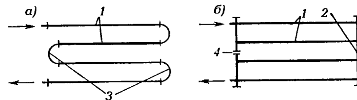
Рис. 4.5. Формы соединения труб в гладкотрубных отопительных приборах: а - змеевиковая форма; б - регистровая форма; 1 - нитки; 2 - колонка; 3 - калачи; 4 - заглушка
