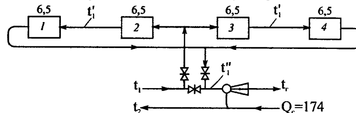
Рис. 10.11. Схема теплопроводов рециркуляционных возду­нагревателей для отопле­ния лестничных клеток жилого здания с элеваторной системой водяного отопле­ния (к примеру 10.9): 1 - 4 - рециркуляционные возду­нагреватели
