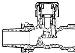
Рис. 5.17. Запорно - регулирующий кран, устанавливаемый на обратной подводе отопительного прибора
