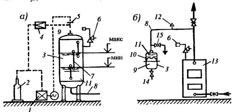
Рис. 3.20. Установка закрытого расширительного бака: а - бак без мембраны; б - бак с мембраной; 1 - воздушный компрессор (вариант 1); 2 - баллон с инертным газом (вариант 2); 3 - расширительный бак; 4 - редукционный клапан; 5 - датчик давления; 6 - предохранительный клапан; 7 - водомерное стекло; 8 - соединительная труба; 9 - инертный газ; 10 - мембрана; 11 - вода; 12 - воздушный кран; 13 - водогрейный котел; 14 - штуцер для заполнения бака инертным газом; 15 - кран для слива воды
