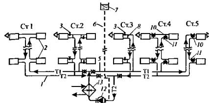
Рис. 6.2. Схема вертикальной одноконтурной системы водяного отопления с нижней разводкой обеих магистралей и П-образными стояками: Ст.1 — проточный стояк, Ст.2 и Ст.3 — стояки со смещенными замыкающими участками; Ст.4 и Ст.5 — проточно-регулируемые стояки, обозначения 1-13 — см. рис. 6.1
