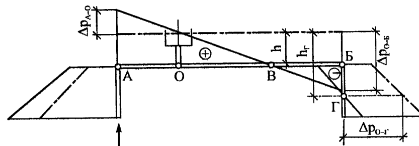
Рис. 7.7. Изменение гидростатического давления в верхней подающей магистрали системы водяного отопления: О - точка постоянного давления; А - точка в зоне нагнетания; Б - точка наибольшего разрежения; В-Г - зона разрежения
