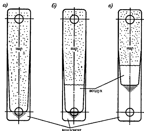
Рис. 9.1. Распределение пара, конденсата и воздуха в отопительном приборе: а - при подаче пара в расчетном количестве; б, в - то же в уменьшенном количестве
