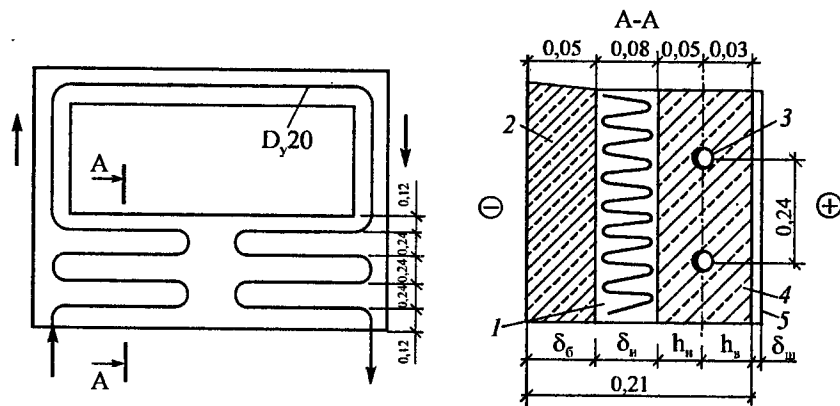
Рис. 11.8. Бифилярный стояк системы водяного отопления с греющими элементами змеевиковой формы, совмещенные с трехслойной наружной стеновой панелью: 1 - тепловая изоляция; 2 - наружный железобетонный слой; 3 - греющая труба; 4 - внутренний железобетонный слой; 5 - штукатурка
