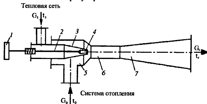
Рис. 3.17. Водоструйный элеватор с регулируемым соплом: 1 - механизм для перемещения регулирующей иглы; 2 - шток регулирующей иглы; 3 - сопло; 4 - регулирующая игла; 5 - камера всасывания; 6 - горловина; 7 - диффузор
