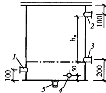
Рис. 3.18. Открытый расширительный бак: 1, 2, 3, 4 - патрубки для присоединения, соответственно, расширительной, переливной, контрольной и циркуляционной труб; 5 - патрубок с пробкой для опорожнения бака
