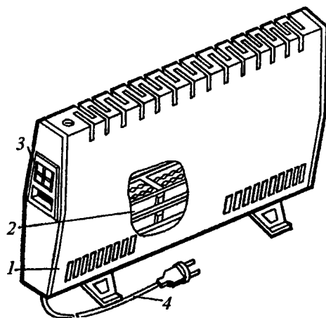
Рис. 14.7. Электроконвектор: 1 - корпус; 2 - нагревательный элемент в виде стальных пластин; 3 - выключатели; 4 - шнур электропитания
