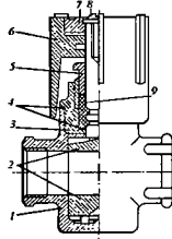
Рис. 5.14. Кран регулирующий трехходовой типа КРТГП: 1 - корпус; 2 - заслонка; 3 - крышка; 4 - прокладка; 5 - гайка сальника; 6 - рукоятка; 7 - крышка-указатель; 8 - винт с шайбой; 9 - сальниковое уплотнение
