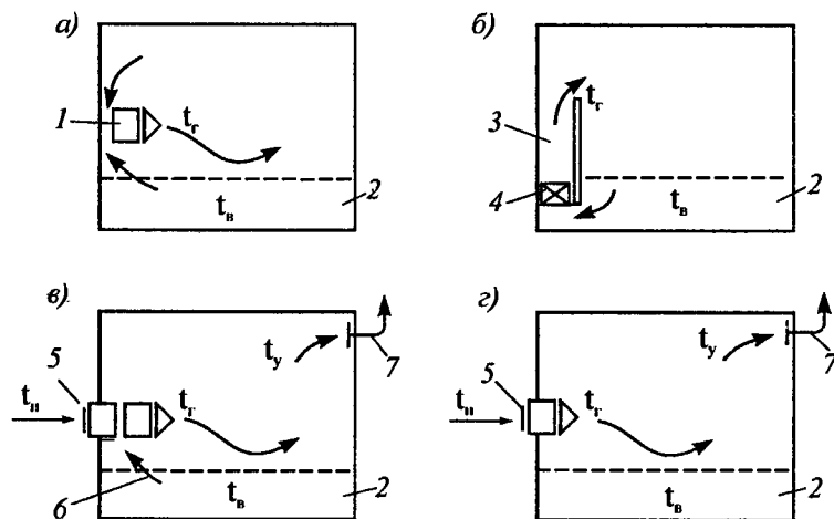
Рис. 10.1. Принципиальные схемы местной системы воздушного отопления: а, б - полностью рециркуляционные; в - частично рециркуляционная; г - прямоточная; 1 - отопительный агрегат; 2 - рабочая (обслуживаемая) зона; 3 - канал с нагретым воздухом; 4 - теплообменник (калорифер); 5 - наружный воздухозабор; 6 - рециркулирующий воздух; 7 - вытяжная вентиляция
