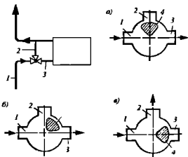
Рис. 5.15. Регулирование расхода воды в отопительном приборе трехходовым краном: а - вода из однострубного стояка полностью протекает в прибор через подводу (заслонка в кране закрывает обходной участок); б - вода частично затекает в прибор; в - вода обходит прибор (заслонка закрывает подводу), протекает полностью в обходной участок и далее в стояк; 1 - однострубный стояк; 2 - обходной участок; 3 - подвода; 4 - заслонка
