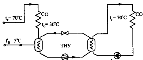
Рис. 19.5. Схема децентрализованного отбора теплоты из обратной магистрали системы центрального отопления (теплоснабжения) с помощью теплового насоса
