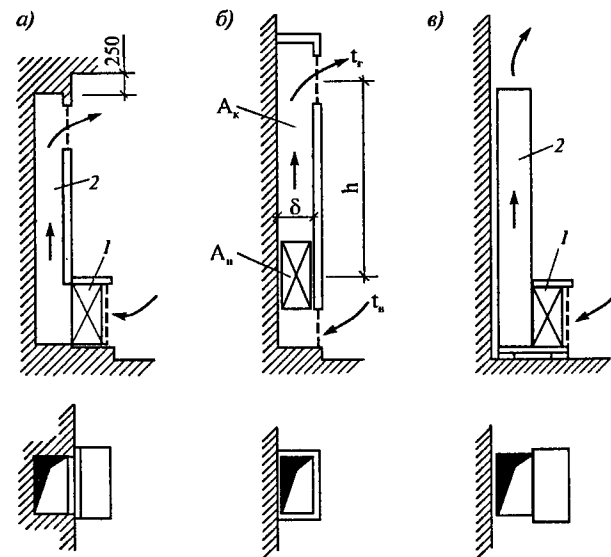
Рис. 10.9. Конструкции рециркуляционных воздушонагревателей: а - со встроенным каналом; б - приставной с каналом из строительных материалов; в - приставной металлический; 1 - нагреватель; 2 - канал горячего воздуха; A_n - площадь нагревателя; A_k - площадь поперечного сечения канала
