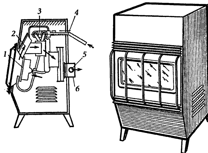
Рис. 13.3. Газовый отопительный камин радиационного действия: 1 - горелка инфракрасного излучения; 2 - теплообменник; 3 - блок автоматики безопасности; 4 - газопровод; 5 - автоматический регулятор тяги; 6 - дымоотводящий патрубок
