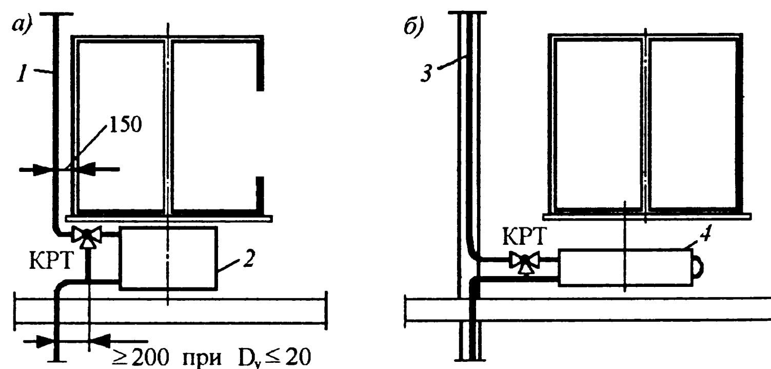
Рис. 5.3 Этажестояки вертикальной однострунной системы водяного отопления с трехходовыми кранами у приборов: а - с приоконным размещением стояка и радиатором (вертикальные оси окна и радиатора совпадают); б - с замоноличенным стояком и конвектором (конвектор смещен к стояку от вертикальной оси окна); 1 - приоконный стояк; 2 - радиатор; 3 - замоноличенный стояк; 4 - конвектор
