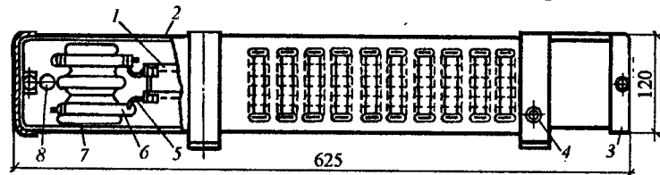
Рис. 14.3. Электронагревательная печь (боковой вид): 1 - трубчатые электронагреватели; 2 - стальной кожух; 3 - крышки; 4 - контакт заземления; 5 - перемычки; 6 - токоведущие шпильки; 7 - дно; 8 - отверстие для ввода электропитания
