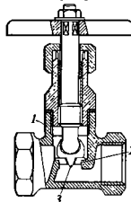
Рис. 5.13. Кран регулирующий с дросселирующим устройством: 1 – сборка корпуса муфтового запорного вентили с крышкой, шпильками, накидной гайкой и рукояткой; 2 – калиброванная диафрагма; 3 – запорно-регулирующий клапан
