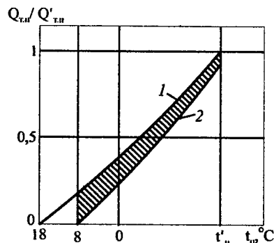
Рис. 17.2. Изменение теплотребности зданий в течение отопительного сезона: 1 - без учета технологических и внутренних тепlopоступлений и солнечной радиации; 2 - с учетом технологических и внутренних тепlopоступлений и солнечной радиации
