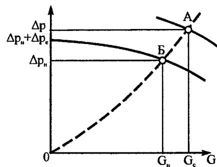
Рис. 7.26. Характеристика насоса (рабочая точка Б) и суммарная характеристика (с учетом естественного циркуляционного давления \Delta p_{\text{с}} , рабочая точка А) применительно к вертикальной однотрубной системе отопления (расход воды изменяется от G_{\text{н}} до G_{\text{с}} )
