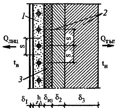
Рис. 11.14. Разрез наружного ограждения с приставной бетонной отопительной панелью: 1 - отопительная панель с односторонней теплоотдачей; 2 - слой наружного ограждения; 3 - тепловая изоляция
