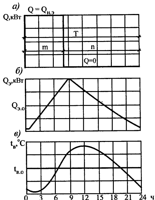
Рис. 14.10. Динамика теплового режима электроаккумулирующего отопительного прибора при 8-часовой зарядке: а - тепловой поток от нагревательных элементов; б - теплопоступление от наружной поверхности отопительного прибора; в - температура воздуха в отапливаемом помещении
