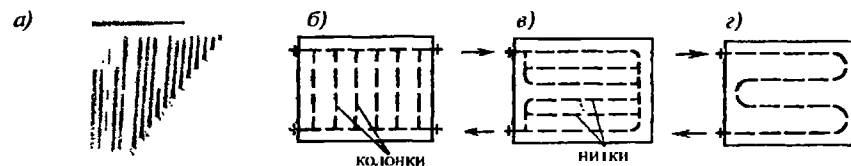
Рис. 4.4. Конструкция стандартного стального панельного радиатора и возможные схемы каналов для теплоносителя в их блоках: а - панельный радиатор марки 22; б - каналы колончатой формы; в - каналы регистровой формы; г - каналы змеевиковой формы
