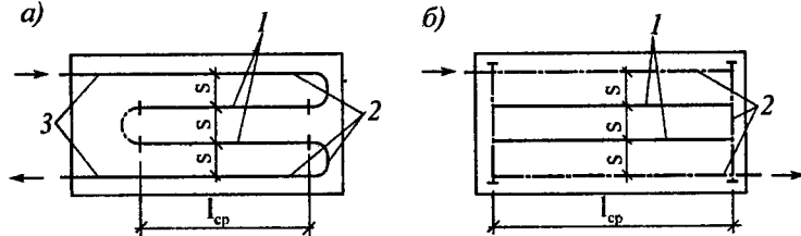
Рис. 11.2. Схемы размещения нагревательных элементов в отопительной панели: а - змеевиковой формы; б - регистровой формы; 1, 2, 3 - соответственно, средние, крайние и одиночные трубы
