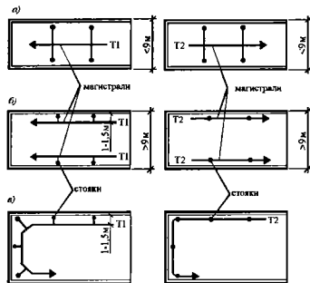
Рис. 5.5. Размещение магистралей систем отопления в чердачных (слева), подвальных и технических (справа) помещениях зданий: а - в зданиях шириной ≤ 9 м; б - в зданиях шириной > 9 м при тупиковом движении теплоносителя в магистралях; в - то же при попутном движении
