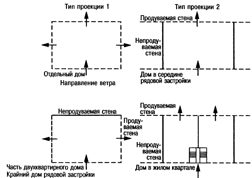
Рис. 3.3. Типы проекций зданий согласно DIN 4701
