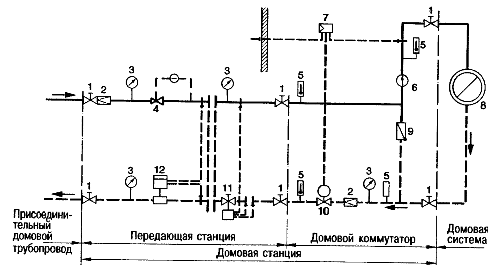
Рис. 11.2. Домовая станция с прямым подключением [4.1]:
