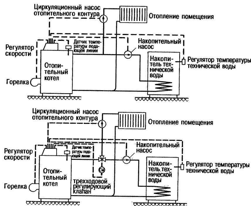
Рис. 9.27. Варианты подключения нагревателя технической воды [4.1]
