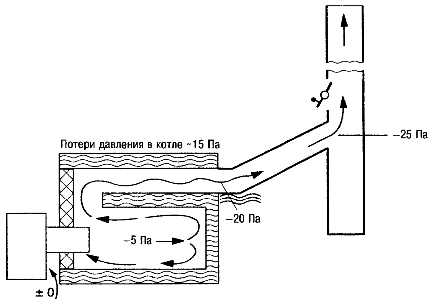
Рис. 5.1. Котел с естественной тягой [5.1]
