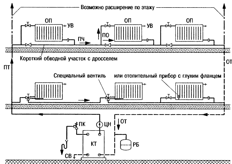
Рис. 9.2. Однотрубная система отопления с нижней разводкой:
