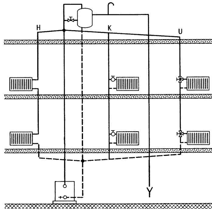
Рис. 9.11. Однотрубная отопительная система с вертикальной разводкой: U — перепускной вентиль; K — короткий обводной участок; H — основной стояк
