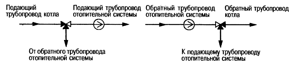
Рис. 8.4. Схема смесительного и распределительного регулирования
