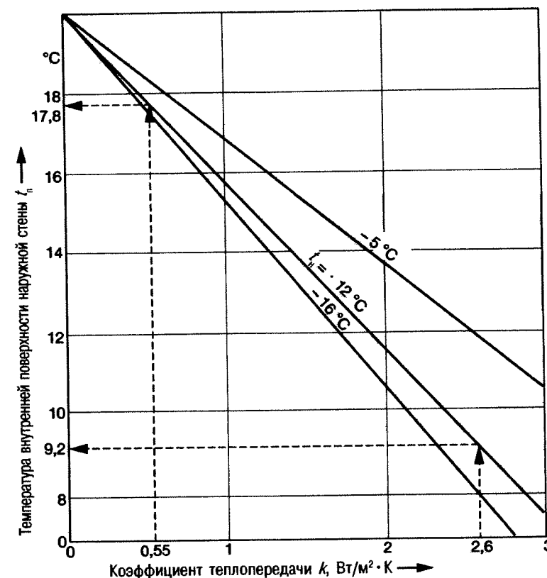
Рис. 1.7. Температура внутренней поверхности наружной стены в зависимости от коэффициента теплопередачи наружной стены k и температуры наружного воздуха [1.4]
