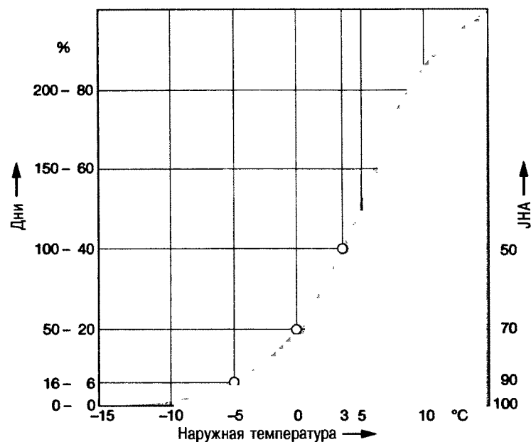
Рис. 5.11. Годовая кривая отопления [5.2]: JNA — суммарный расход теплоты за отопительный период (площадь, ограниченная кривой и осями ординат)
