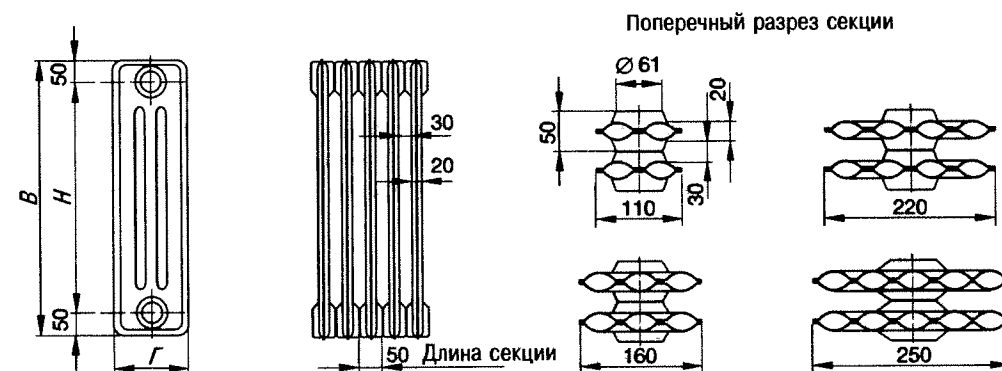
Рис. 4.2. Стальной радиатор DIN 4703 [4.1]: B — высота; H — номинальный размер; G — глубина
