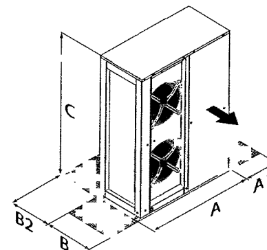
Рис. 12. Размеры блоков WBAN
