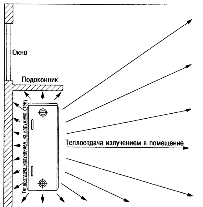
Рис. 4.12. Поступление теплоты от отопительного прибора
