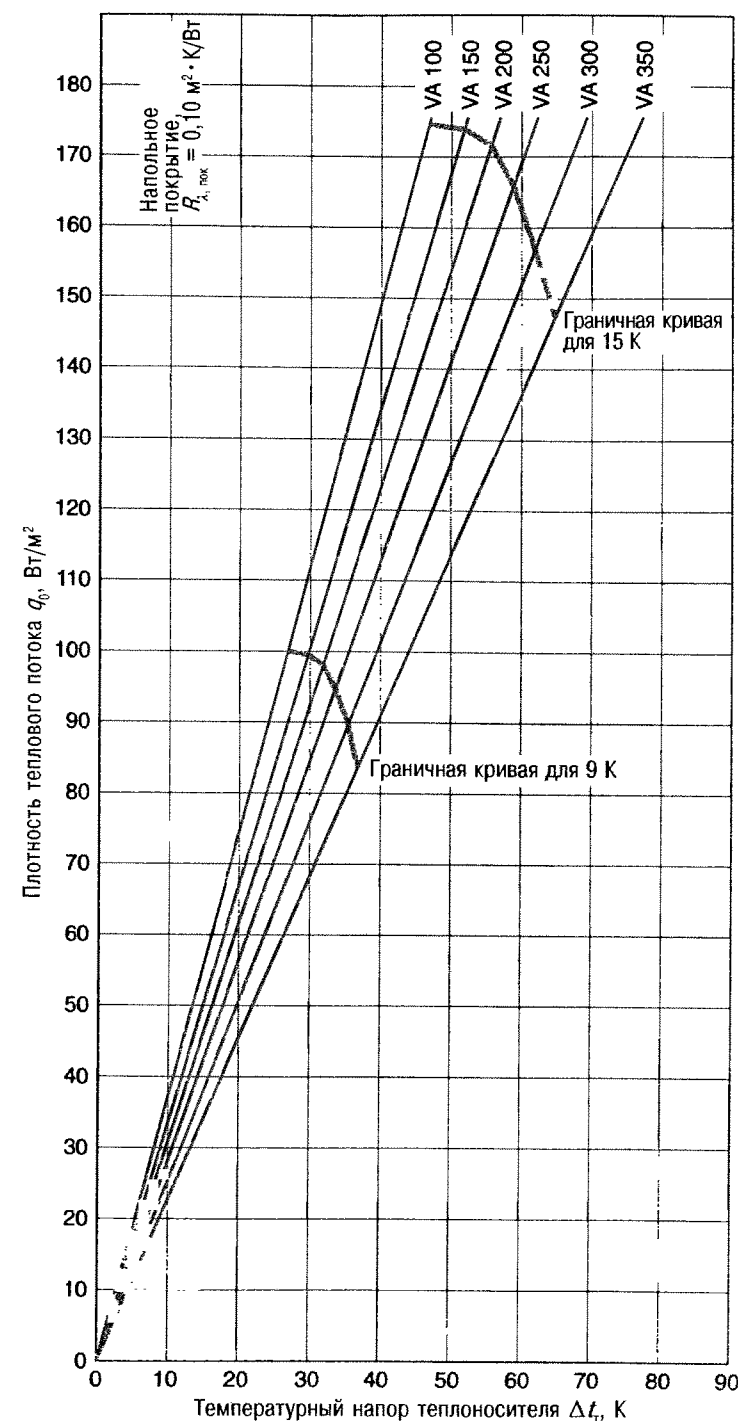
Рис. 9.18. Термическое сопротивление напольного покрытия [9.3]; R_{\lambda, \text{пок}} = 0,10 \text{ м}^2 \cdot \text{К/Вт} ; VA — шаг укладки, мм
