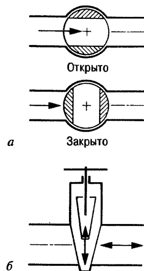
Рис. 8.5. Кран (а) и шибер (б), схематическое изображение
