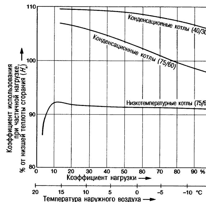
Рис. 5.13. Коэффициент использования [5.2]
