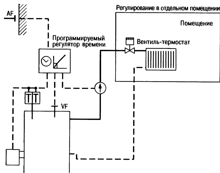
Рис. 9.24. Типовой вариант регулирования температуры воды в подающей линии в зависимости от температуры наружного воздуха:
