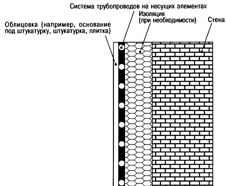
Рис. 4.10. Возможный способ установки на стену
