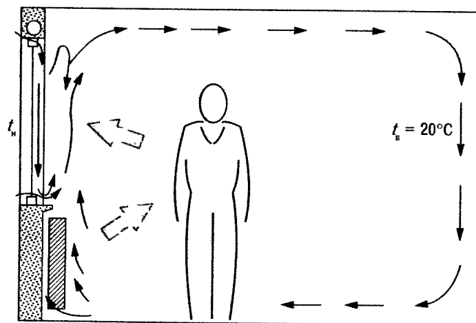
Рис. 1.8. Воздушный поток в помещении, которое отопляется с помощью радиатора [1.4]
