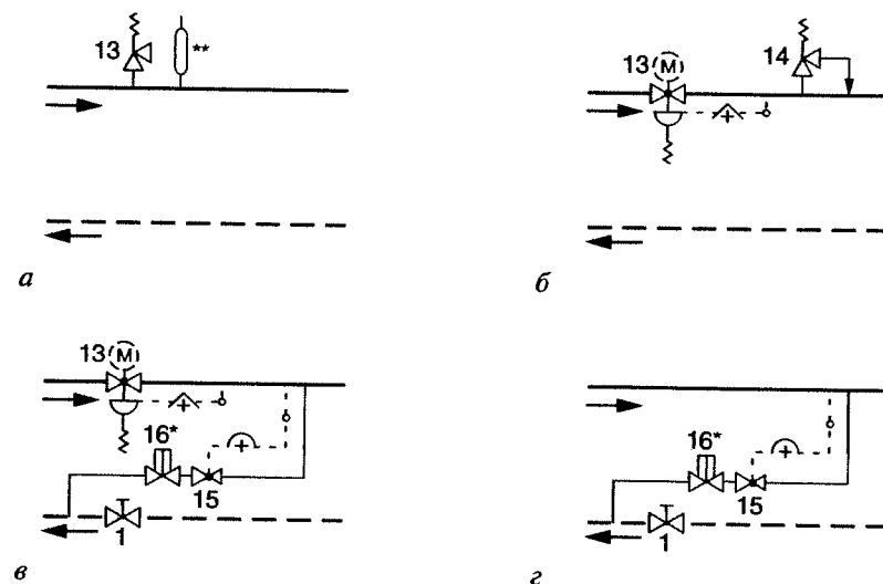
Рис. 11.3. Предохранительное оборудование [4.1]: а — с предохранительным клапаном (ПК); б — с запорным предохранительным вентилем (ЗПВ) в соединении с предохранительным клапаном (ПК) (импульс на закрытие ЗПВ дает датчик давления); в — с запорным предохранительным вентилем (ЗПВ) в соединении с предохранительным перепускным вентилем (ППВ); г — с предохранительным перепускным вентилем (ППВ).
