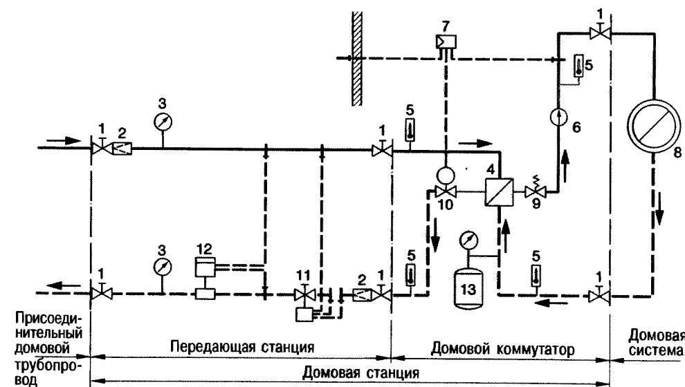
Рис. 11.4. Домовая станция с непрямым подключением [4.1]:
