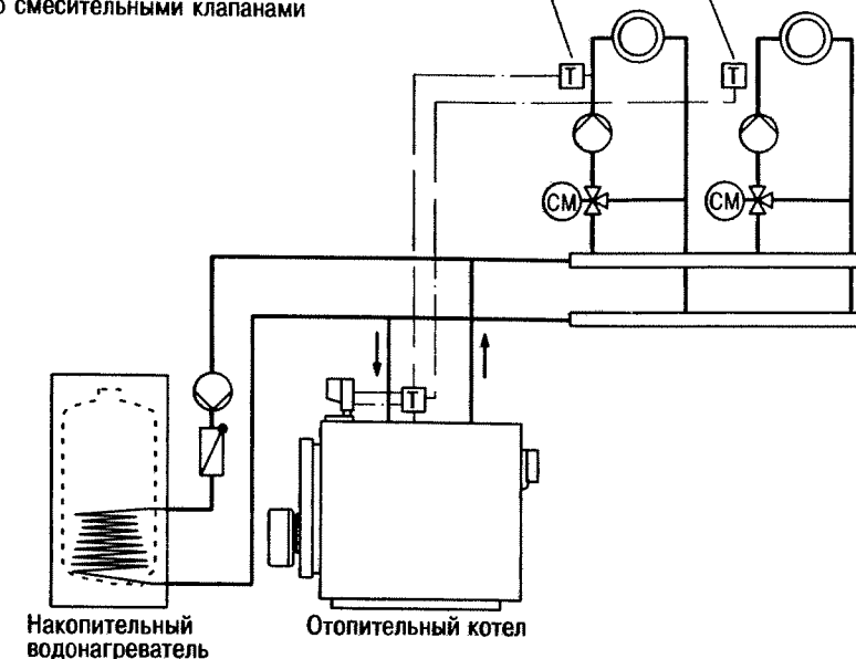
Рис. 9.25. Пример подключения [9.5]:
