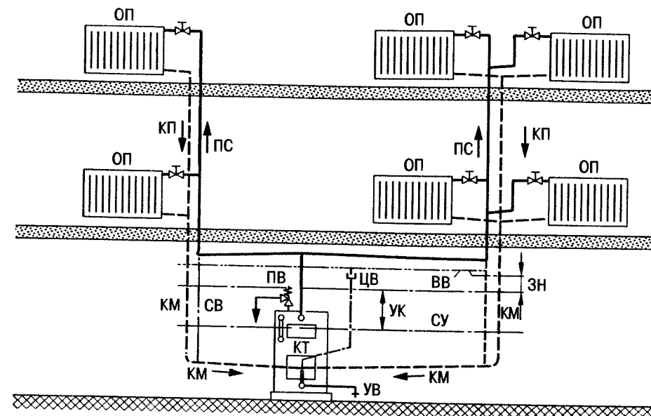
Рис. 10.3. Нижняя разводка с мокрым конденсатопроводом [4.1]:
