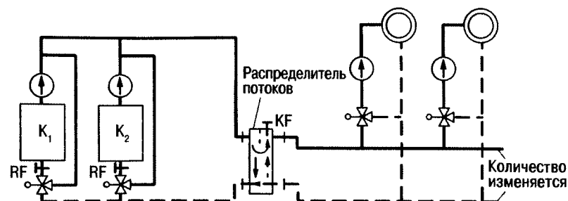
Рис. 9.32. Схема теплоснабжения с распределителем потоков воды [9.4]: KF — датчик регулирования температуры в котле (КД); RF — датчик регулирования температуры обратной линии (ОД); K 1 , K 2 — котел 1, 2
