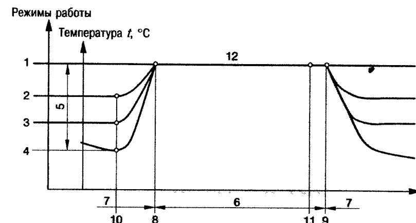
Рис. 9.28. Виды режимов [9.2]:
