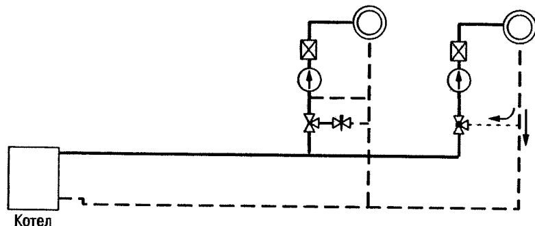
Рис. 9.30. Разводка без основного насоса [9.4]
