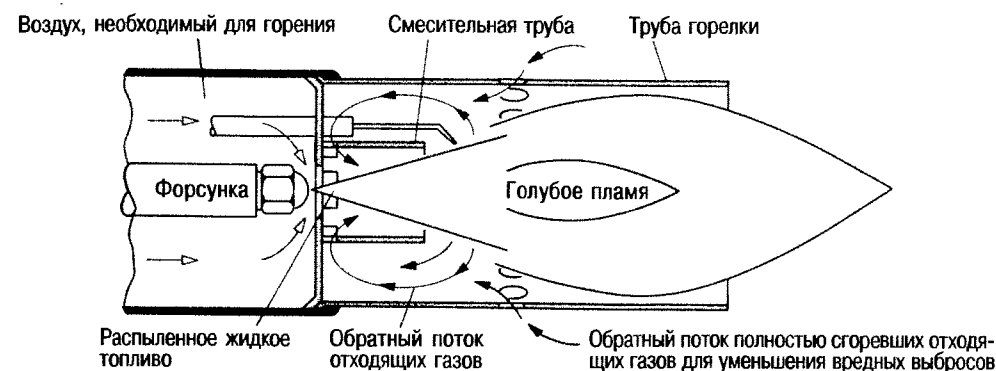
Рис. 5.4. Реактивный принцип смешения с обратным потоком отходящих газов [4.1]
