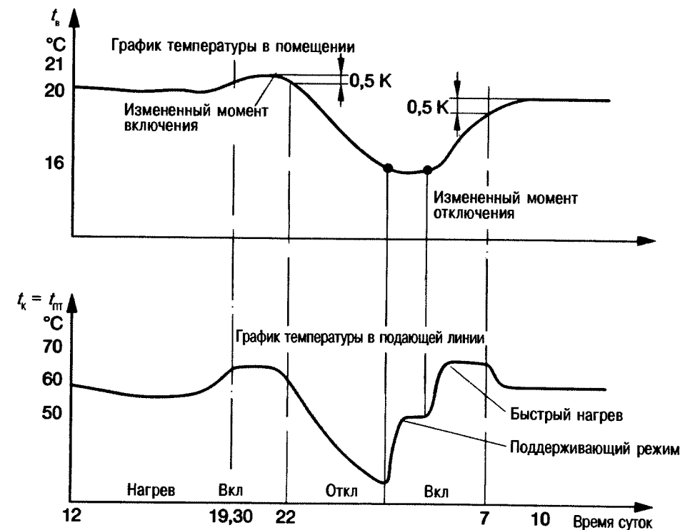
Рис. 9.29. Различные представления графиков изменения температуры [9.4]
