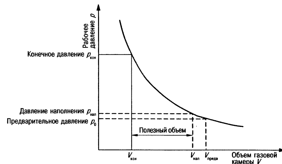
Рис. 9.6. Мембранные расширительные баки
