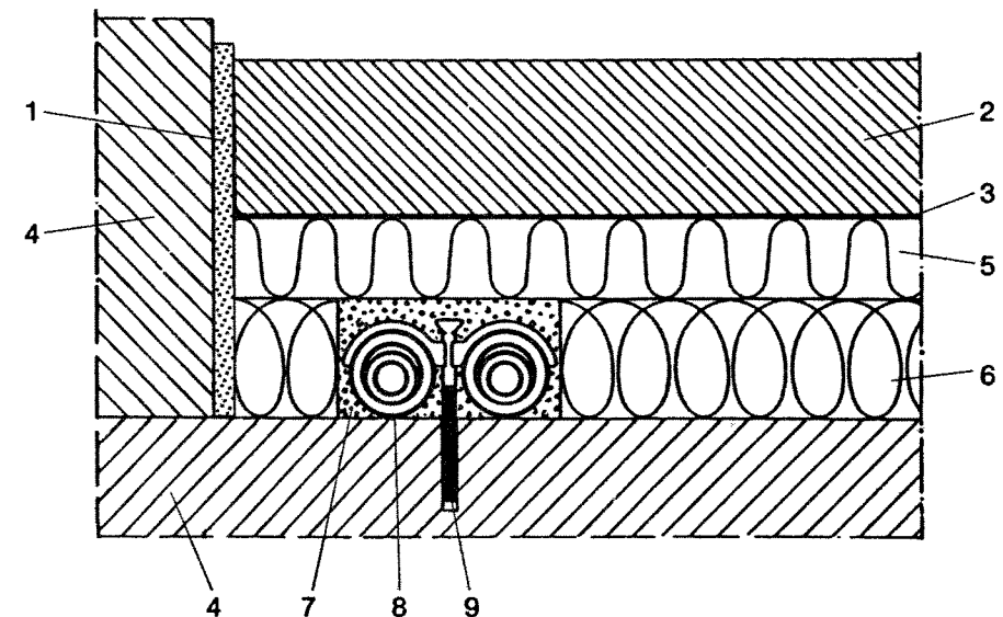
Рис. 8.1. Пример прокладки трубопроводов в полу [8.1]:
