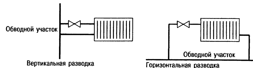
Рис. 9.13. Схематическое представление коротких обводных участков
