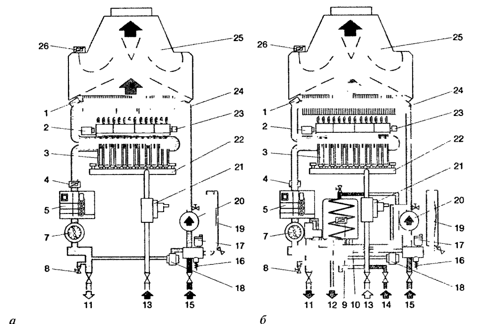
Рис. 5.14. Принципиальная схема настенного отопительного котла [5.3]:
