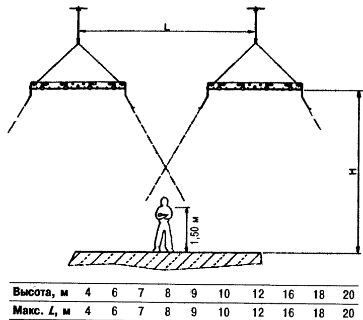
Рис. 6. Максимальное расстояние между панелями
