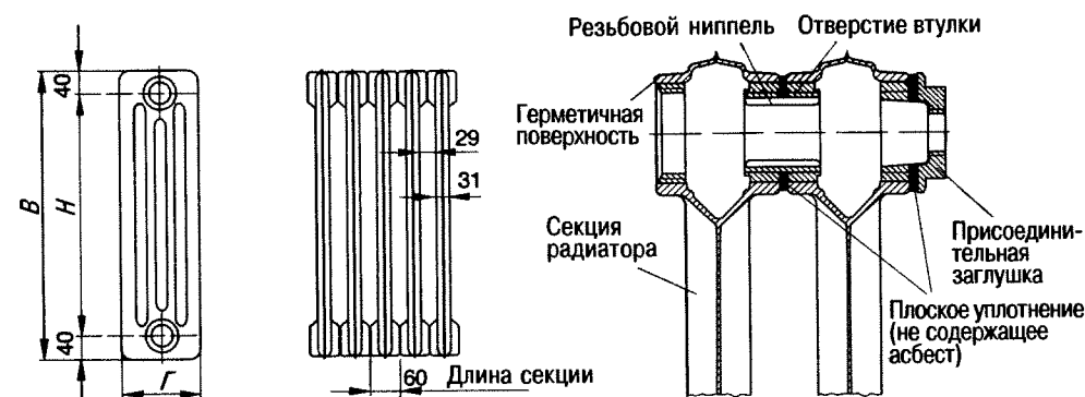
Рис. 4.1. Чугунный радиатор DIN 4703 [4.1]: B — высота; H — номинальный размер; G — глубина
