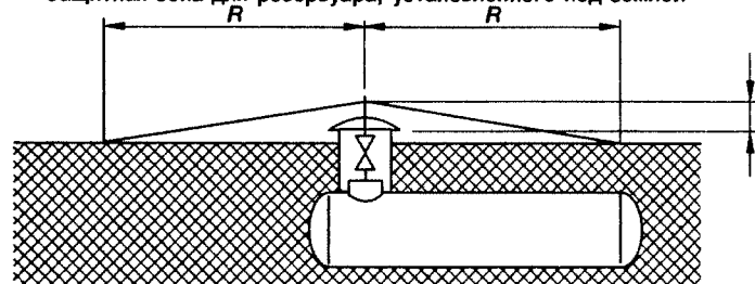
Рис. 7.1. Защитные зоны согласно Распоряжению о топочных системах
