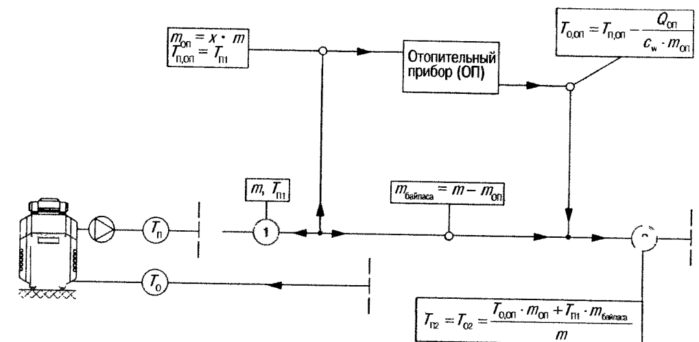
Рис. 9.15. Баланс температуры и массового потока воды: T_п — температура в подающей линии; T_о — температура в обратной линии
