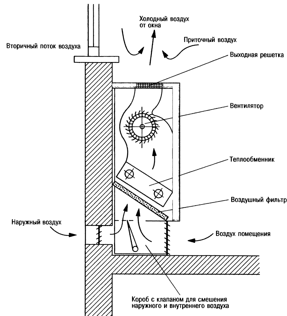
Рис. 4.6. Принципиальная схема вентиляторного конвектора [4.1]
