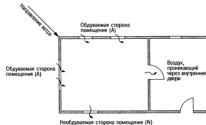
Рис. 3.2. Обдуваемые и необдуваемые стороны помещения, согласно DIN 4701
