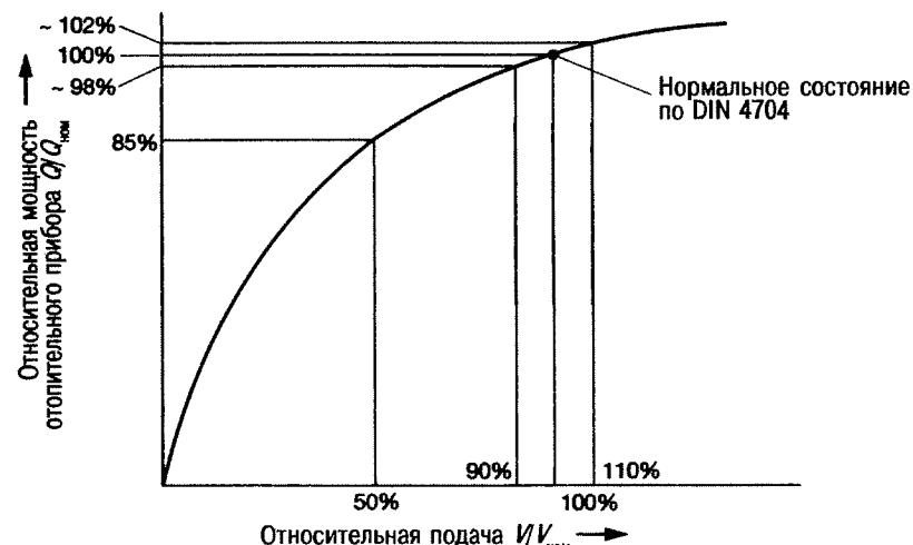
Рис. 8.10. Диаграмма мощности отопительного прибора [8.3]
