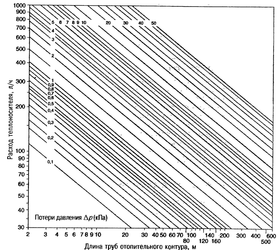
Рис. 9.20. Потери давления: системная отопительная труба Roth-PEX / соединительная труба Roth-Alu-Laserpex 17 мм [9.3]
