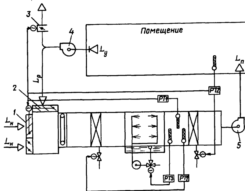
Рис. 13.7. Схема СКВ с первой рециркуляцией: 1 — двустворчатый утепленный клапан; 2 — одностворчатый клапан; 3 — дроссельный клапан; 4 — вытяжной вентилятор; 5 — приточный вентилятор
