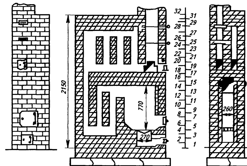
Рис. 3.2. Печь ПТО-4800
