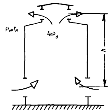
Рис. 5.1. Аэрация здания под воздействием гравитационного давления ( t_n < t_v )
