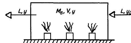
Рис. 6.1. Расчетная схема к выводу уравнения воздухообмена
