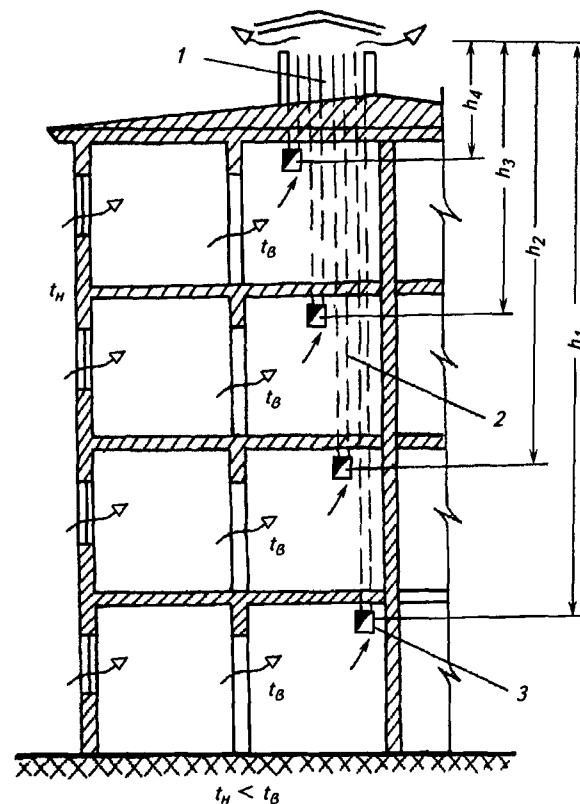
Рис. 5.5. Естественная гравитационная система вентиляции помещений многоэтажного здания: 1 — воздуховыбросная шахта; 2 — каналы; 3 — воздухоприемное отверстие
