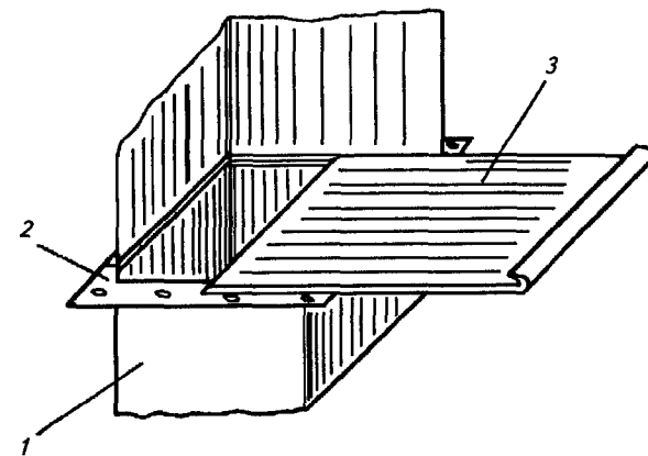
Рис. 5.21. Шибер:
