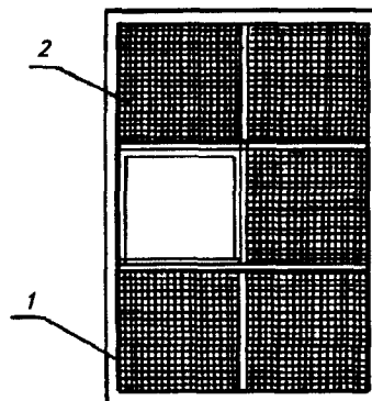
Рис. 8.4. Панель из ячейковых фильтров: 1 — корпус; 2 — ячейка фильтра
