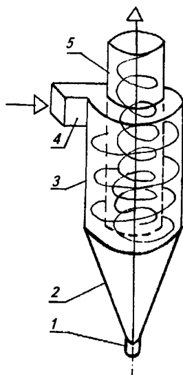
Рис. 8.8. Циклон:
