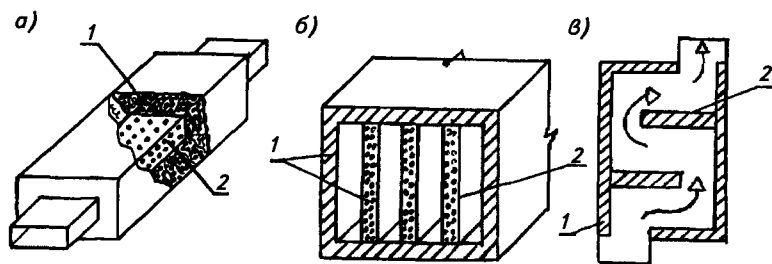
Рис. 7.9. Шумоглушители: а — трубчатый; б — пластинчатый; в — камерный; 1 — звукопоглощающий материал; 2 — сетка или перфорированная оболочка
