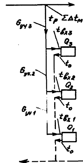
Рис. 4.24. Расчетная схема двухтрубного стояка с верхним расположением подающей магистрали
