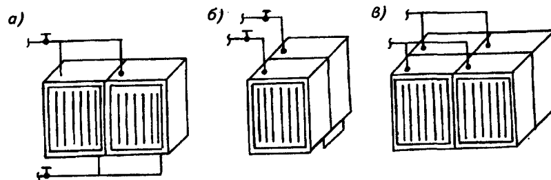
Рис. 11.2. Схема установки одноходовых калориферов: а — параллельная по воздуху и теплоносителю воде или пару; б — последовательная по воздуху и теплоносителю воде; в — смешанная по воздуху и теплоносителю воде
