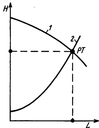
Рис. 7.7. Наложение характеристики сети на характеристику вентилятора: 1 — характеристика вентилятора; 2 — характеристика сети воздухопроводов; PT — рабочая точка
