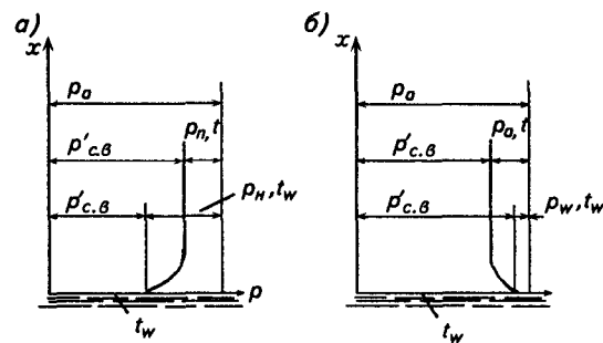
Рис. 9.8. Распределение парциальных давлений сухого воздуха и водяного пара в результате взаимодействия воздуха и воды при их непосредственном контакте: а — при конденсации водяного пара на поверхности воды; б — при испарении воды
