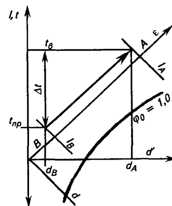
Рис. 6.2. Построение на I-d -диаграмме процесса изменения состояния воздуха при ассимиляции избытков теплоты и влаги
