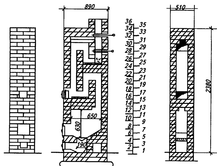
Рис. 3.3. Печь ПТО-2500
