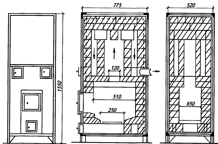
Рис. 3.4. Печь ПТК-3000
