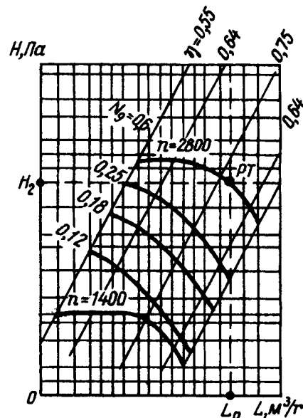
Рис. 7.8. Выбор вентилятора по его характеристике: H — расчетное давление; L — расчетный расход воздуха; n — частота вращения, об/с; N_d — мощность двигателя вентилятора
