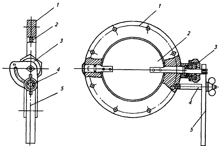
Рис. 5.22. Дроссельный клапан:
