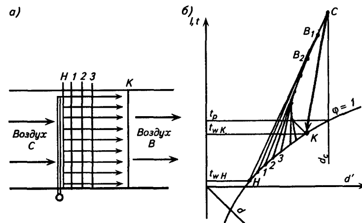
Рис. 10.3. Охлаждение воздуха водой при их попутном параллельном движении: а — схема движения воздуха и капель воды; б — построение на t-d' -диаграмме процесса изменения состояния воздуха
