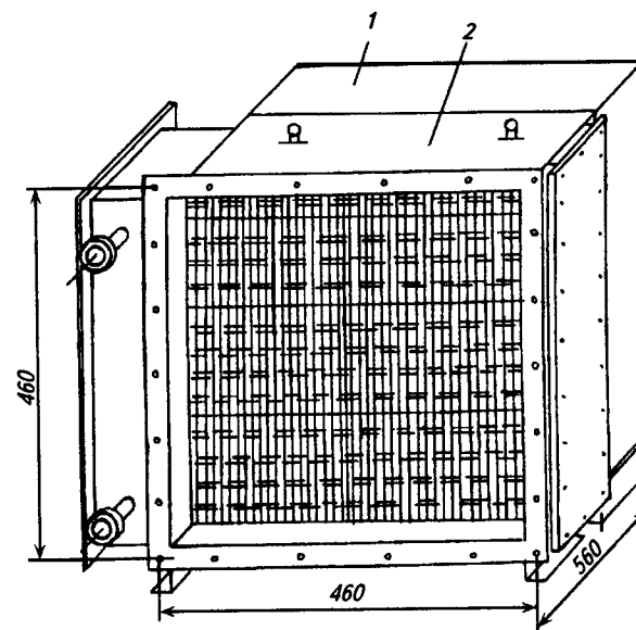
Рис. 11.8. Воздухоохладитель:
