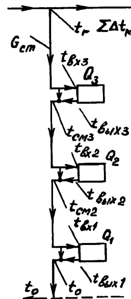
Рис. 4.26. Расчетная схема однострубного стояка с замыкающими участками
