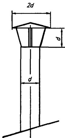
Рис. 5.28. Воздуховыбросная шахта
