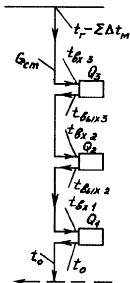
Рис. 4.25. Расчетная схема проточного стояка однострубной системы водяного отопления
