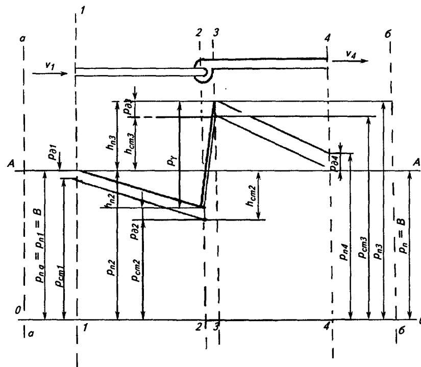
Рис. 7.4. Эпюра давлений воздуха в воздухопроводе постоянного сечения ( p_{\text{г}} — напор, развиваемый вентилятором)
