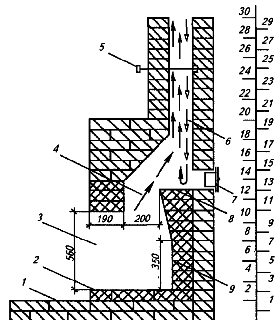
Рис. 3.5. Камин с прямым газоходом:
