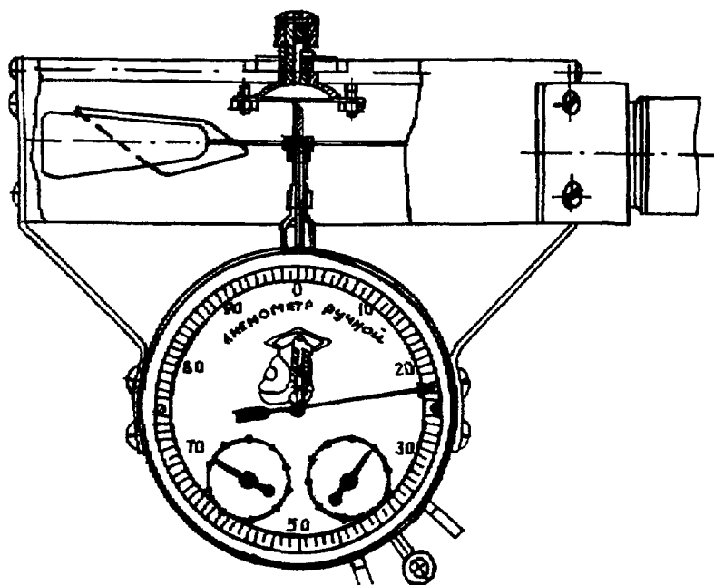
Рис. 14.3. Крыльчатый анемометр
