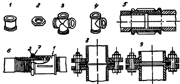
Рис. 4.11. Фасонные части труб и способы соединения труб:
