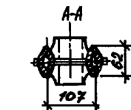
Рис. 4.12. Чугунный радиатор МО-140-108 (МС-140-98)
