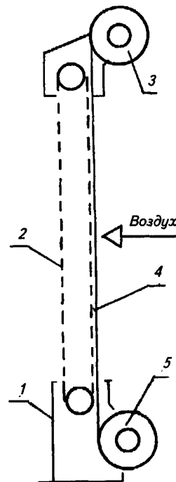
Рис. 8.2. Рулонный фильтр:
