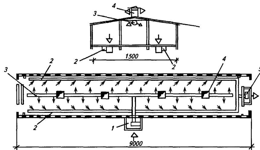
Рис. 5.37. Система вентиляции помещений животноводческого здания: 1 — приточная камера; 2 — воздуховоды для вытяжки из навозных каналов; 3 — приточный воздуховод; 4 — вытяжная шахта; 5 — вытяжная камера
