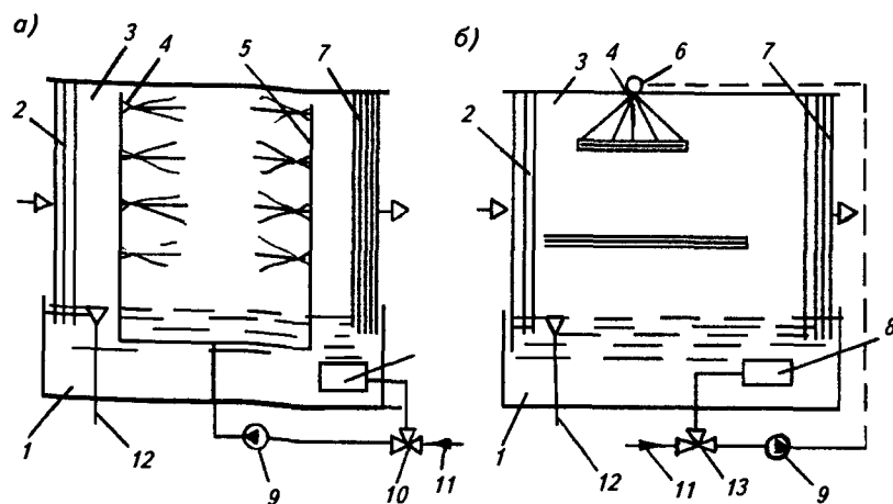
Рис. 10.1. Принципиальные схемы форсуночных камер орошения: а — с вертикальными стойками; б — с горизонтальным коллектором;
