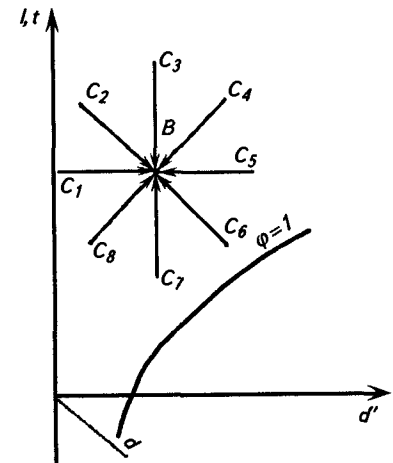
Рис. 9.2. Изображение на I-d -диаграмме возможных процессов тепловлажностной обработки воздуха при кондиционировании
