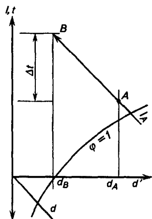
Рис.12.3. Изображение на I - d -диаграмме процесса осушки воздуха в слое твердого сорбента
