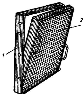
Рис. 8.3. Ячейковый фильтр ФяР: 1 — установочная рамка; 2 — ячейка фильтра
