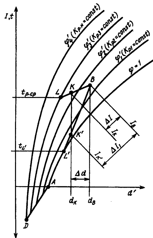
Рис. 12.5. Изображение на I - d -диаграмме процесса осушки
