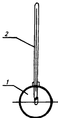
Рис. 14.8. Шаровой термометр: 1 — пустотелый шар; 2 — термометр
