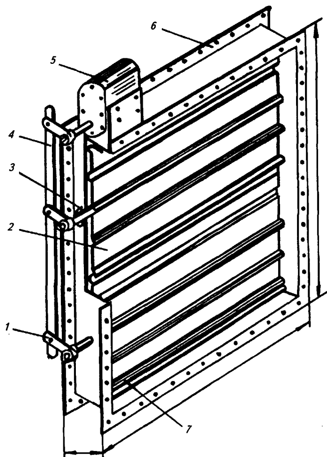
Рис. 5.25. Многостворчатый клапан: 1 — рычаг; 2 — створка; 3 — полуось; 4 — тяга; 5 — электропровод; 6 — корпус; 7 — пластина-ограничитель
