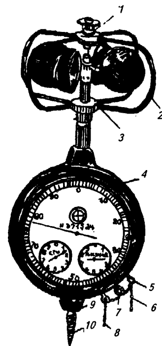
Рис. 14.4. Чашечный анемометр:
