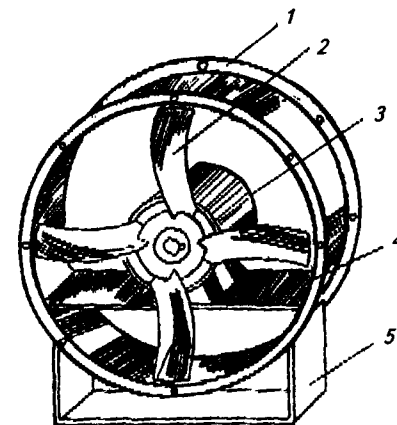
Рис. 5.15. Осевой вентилятор:
