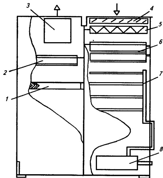
Рис. 5.34. Неавтономный кондиционер:
