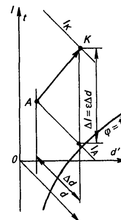
Рис. 1.7. Построение линий изменения состояния воздуха
