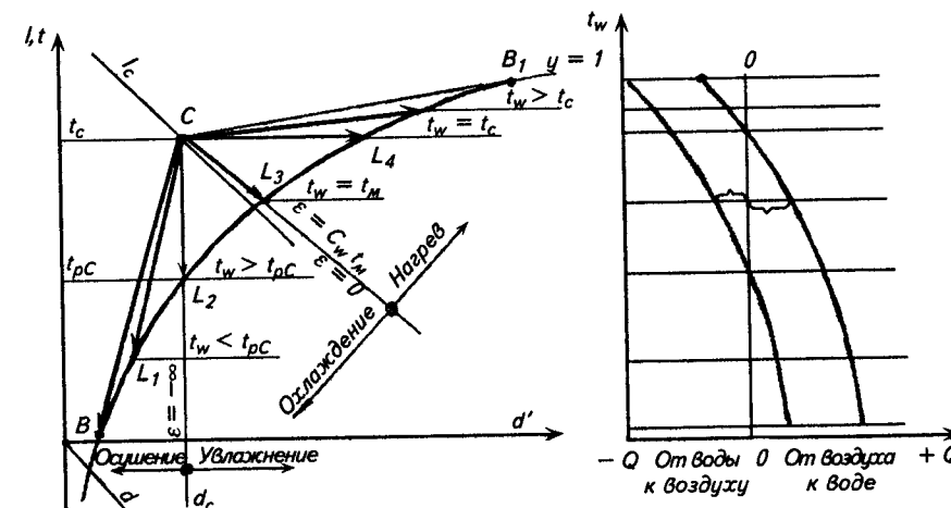
Рис. 9.10. Область возможных процессов тепловлажностной обработки воздуха водой
