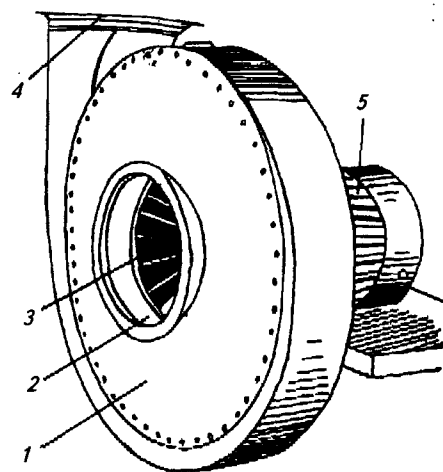
Рис. 5.14. Радиальный вентилятор:
