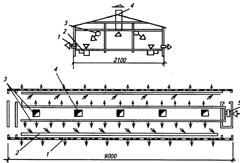
Рис. 5.39. Система вентиляции помещений животноводческого здания: 1 — осевые вентиляторы; 2 — воздуховоды для вытяжки воздуха из навозных каналов; 3 — приточные воздуховоды; 4 — вытяжные шахты; 5 — приточная камера
