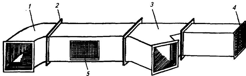
Рис. 5.20. Элементы воздуховода:
