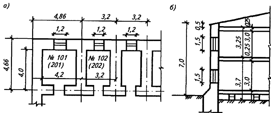
Рис. 2.3. План (а) и разрез (б) двухэтажного здания общежития
