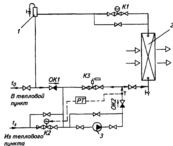
Рис. 13.10. Принципиальная схема смесительной установки теплоснабжения воздухонагревателей второго подогрева: 1 — воздухооборник; 2 — воздухонагреватель второго подогрева; 3 — насос
