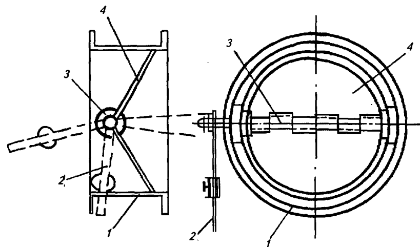
Рис. 5.24. Обратный клапан:
