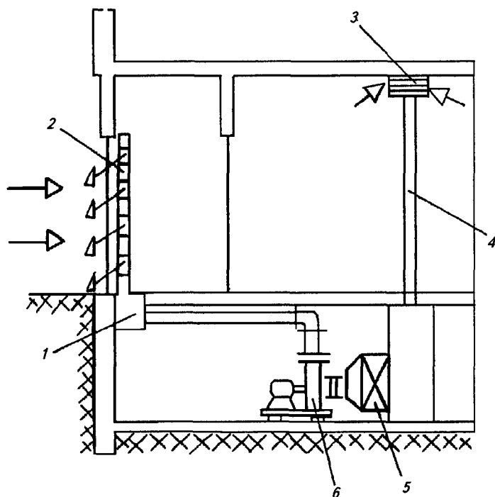
Рис. 5.8. Воздушно-тепловая завеса:
