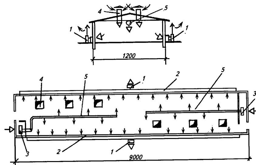
Рис. 5.40. Система вентиляции птицеводческого здания: 1 — вытяжной вентилятор; 2 — вытяжные воздуховоды; 3 — приточные камеры; 4 — приточные шахты; 5 — приточные воздуховоды
