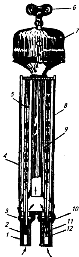
Рис. 14.7. Аспирационный психрометр:
