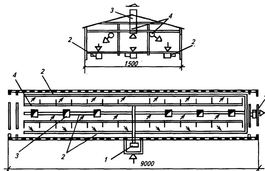
Рис. 5.38. Система вентиляции помещений животноводческого здания: 1 — приточная камера; 2 — воздуховоды для вытяжки из навозных каналов; 3 — вытяжные шахты; 4 — приточные воздуховоды; 5 — вытяжная камера
