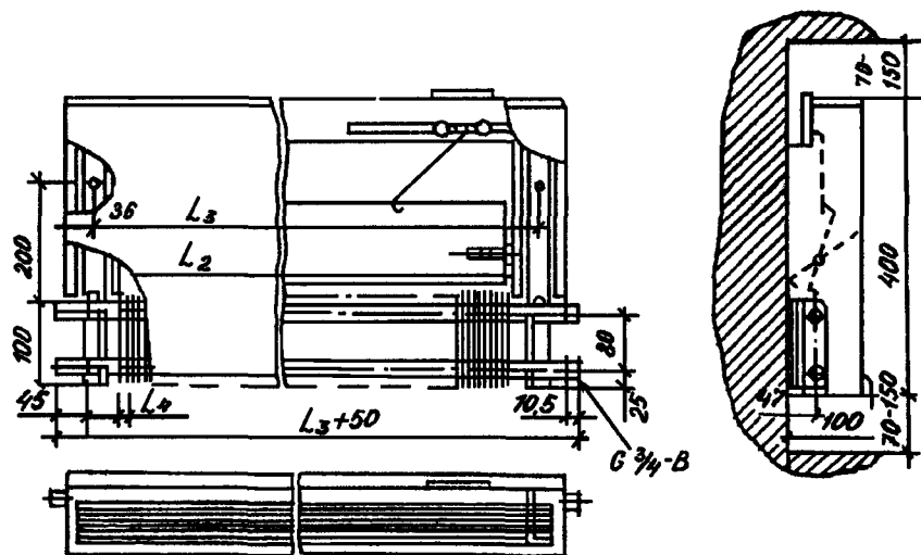
Рис. 4.14. Конвектор «Универсал» проходной
