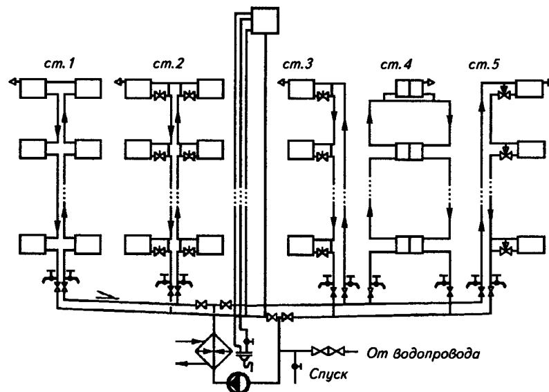
Рис. 4.5. Однетрубная система водяного отопления с нижней разводкой П-образными стояками и искусственной циркуляцией воды:
