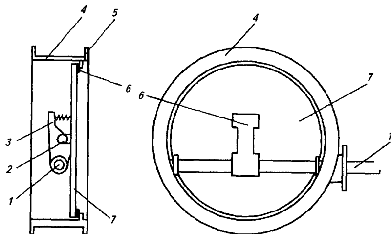
Рис. 5.23. Герметический клапан:
