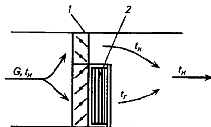
Рис. 11.7. Схема регулирования теплоотдачи воздушонагревательной установки: 1 — двохвальный секционный клапан; 2 — воздушонагреватель; t_r — температура горячего воздуха после калорифера
