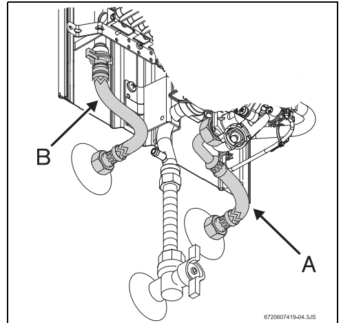
Рис. 10 Подключение водопровода
