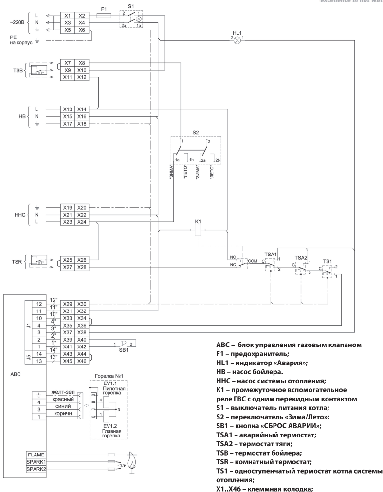
Рисунок 9. Электрическая схема котла ALFA COMFORT E 25; ALFA COMFORT E 35; ALFA COMFORT E 40; ALFA COMFORT E 45 (одноступенчатого).
