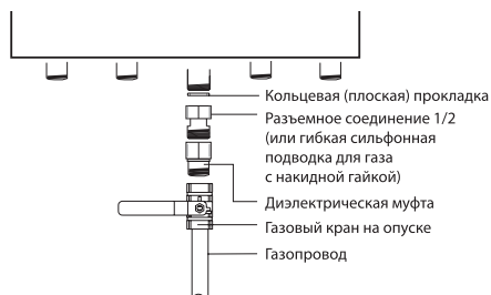
Подсоединение газопровода
