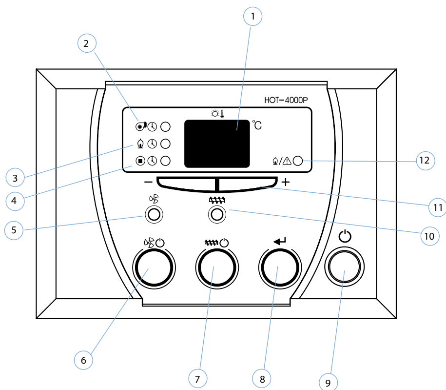
Рисунок 2. Блок управления HOT-4000P
