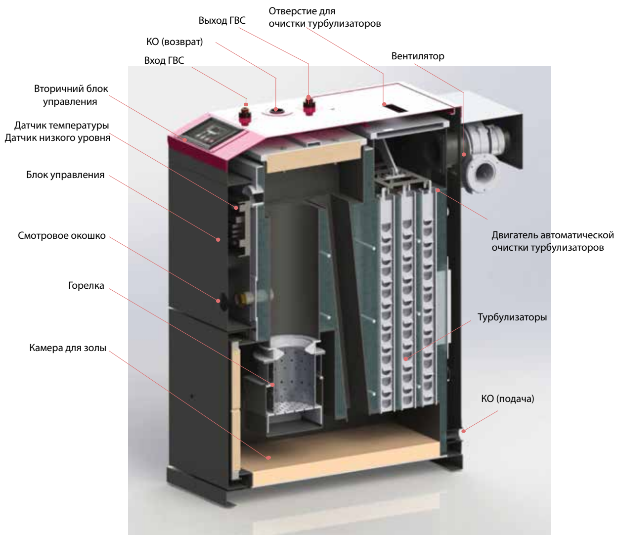
Рисунок 4. Функциональная схема котла
