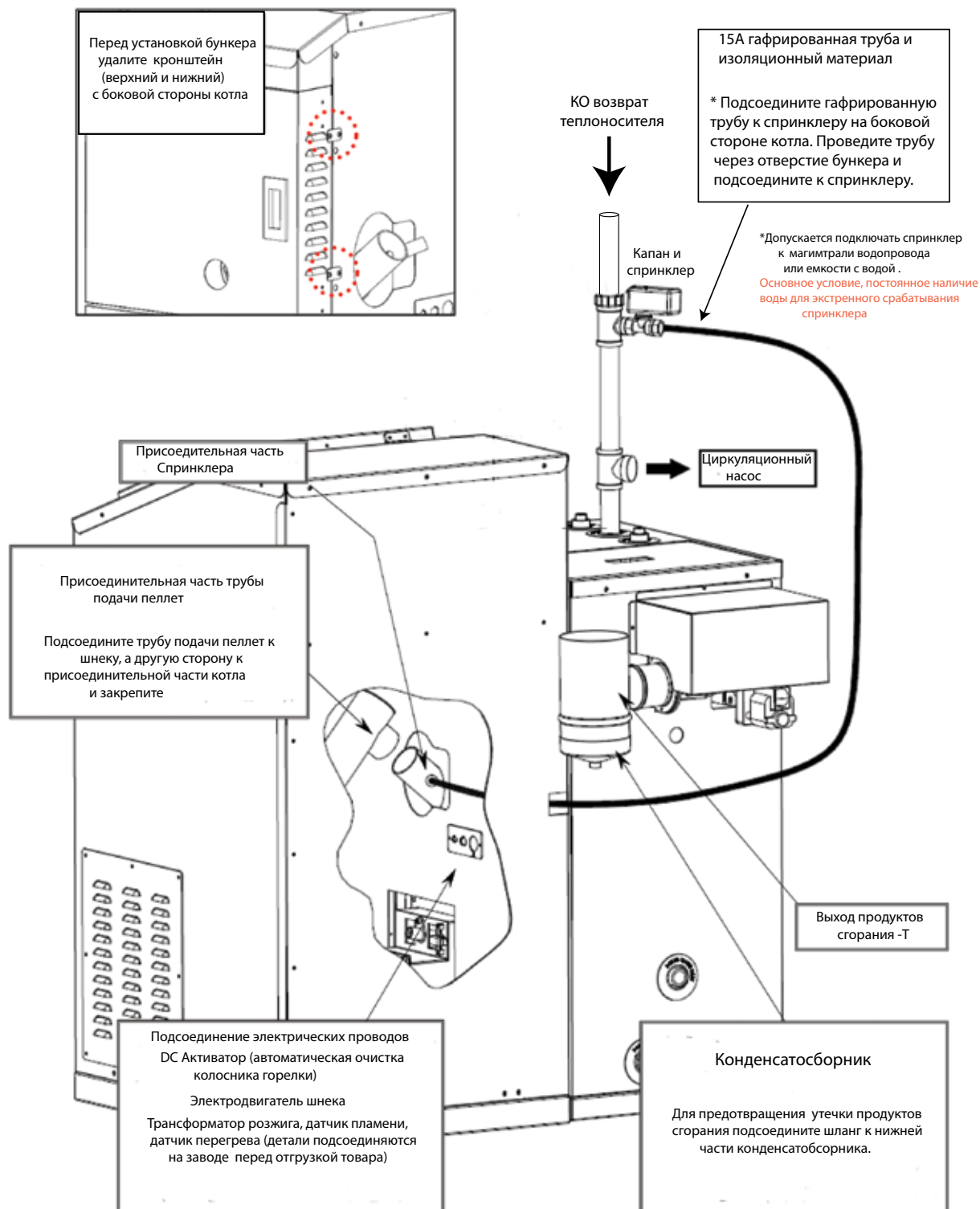
Рисунок 18 Порядок сборки бункера для пеллет и акссесуаров ( вид котла с тыла)
