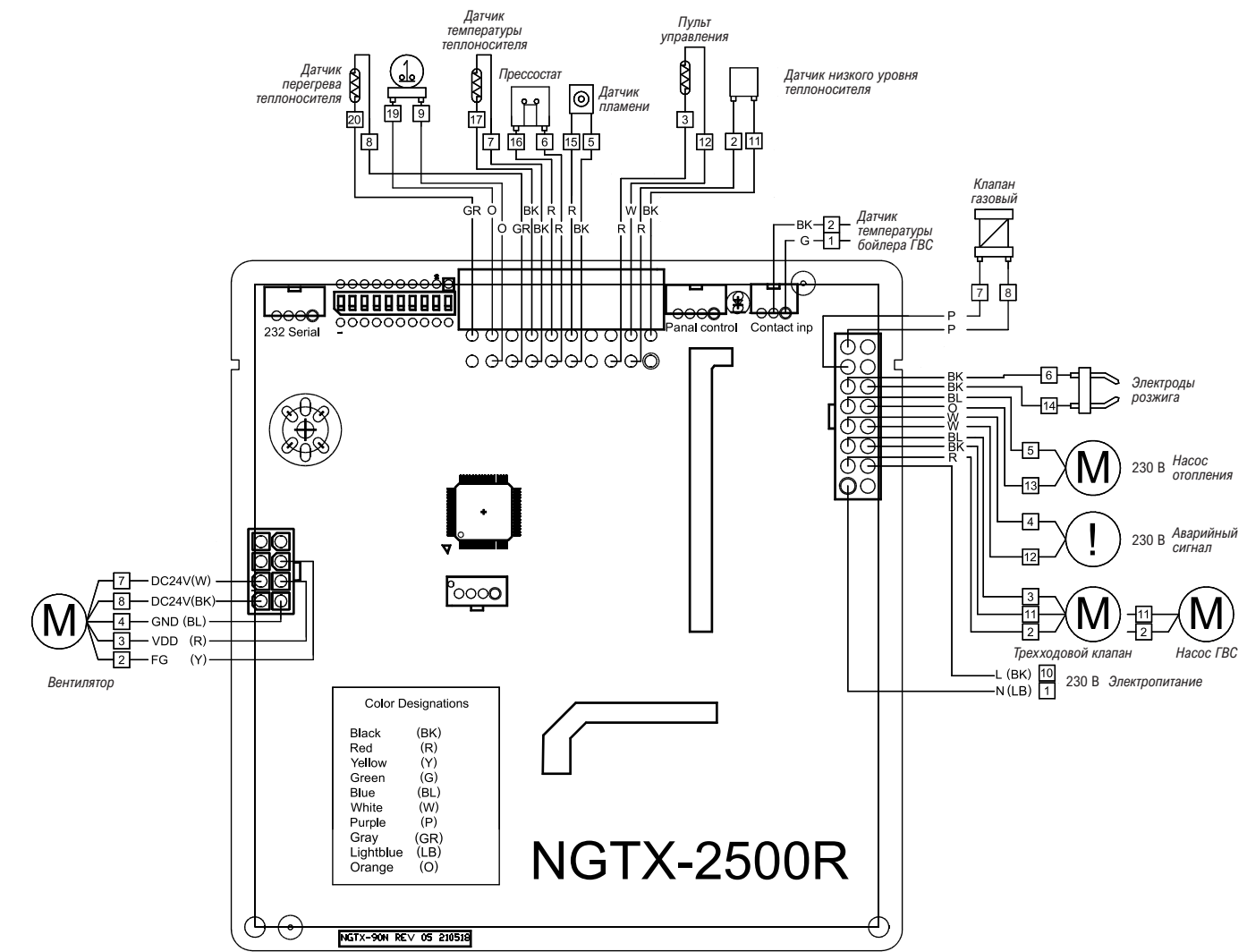
Рисунок 13. Схема электрических соединений.
