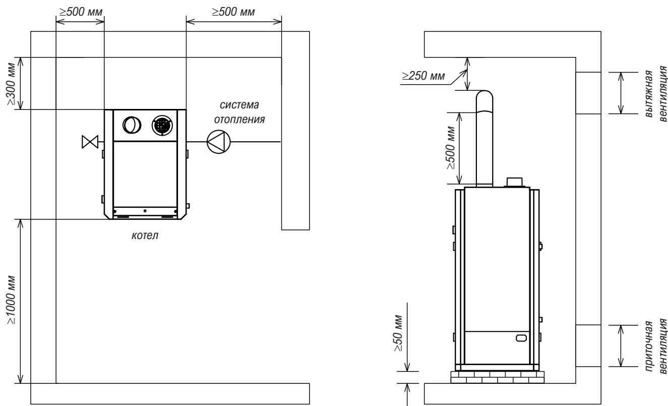
Рисунок 6. Пространство для технического обслуживания.
