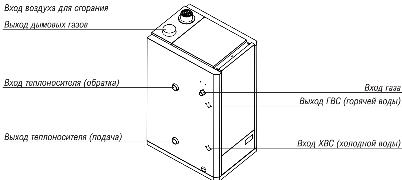
Рисунок 2. Подключение системы дымоудаления, газоснабжения, труб системы отопления и ГВС.
