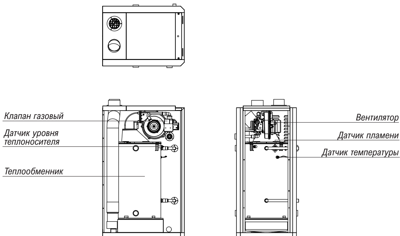
Рисунок 3. Основные узлы STSG-47.
