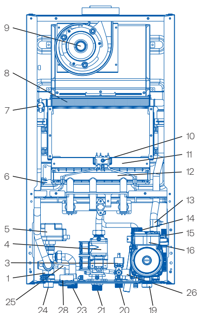
Одноконтурные котлы: TechLine S 1.14/1.18/1.24/1.28TW
