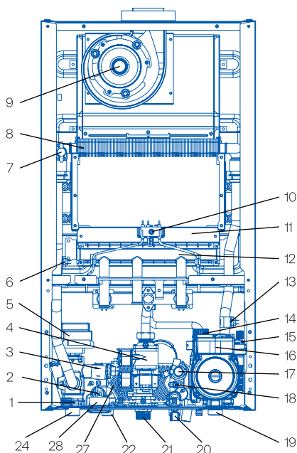
Екі контурлы қазандықтар: TechLine S 2.10/2.14/2.18/2.24/2.28TW(TWs)
