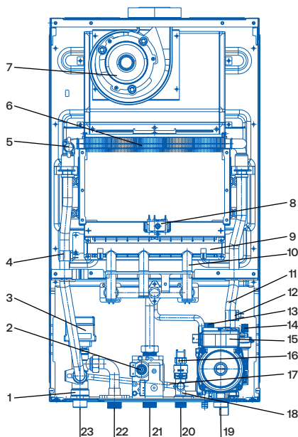
Одноконтурные котлы: EliteLine 1.24TW
