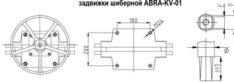
DN500-600 вид сверху и размер штока для задвижки шиберной ABRA-KV-02
