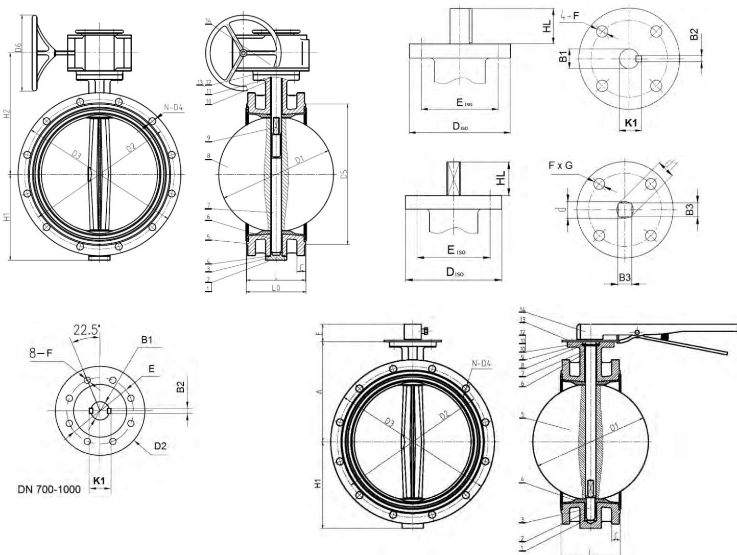
Чертеж габаритный затвора поворотного дискового чугунного фланцевого с рукояткой (Н) или редуктором (Г) ABRA-BUV-FLzzz и посадочными присоединительными размерами
