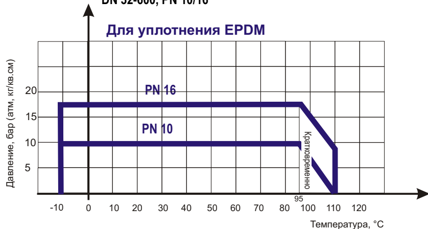
Диаграмма Давление / Температура для затвора поворотного дискового ABRA-BUV-VF826Dxxx и ABRA-BUV-VF866D DN 32-600, PN 10/16
