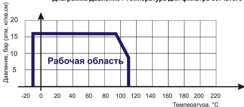
Диаграмма Давление / Температура для фильтра сетчатого латунного резьбового ABRA-YS-3000-E
