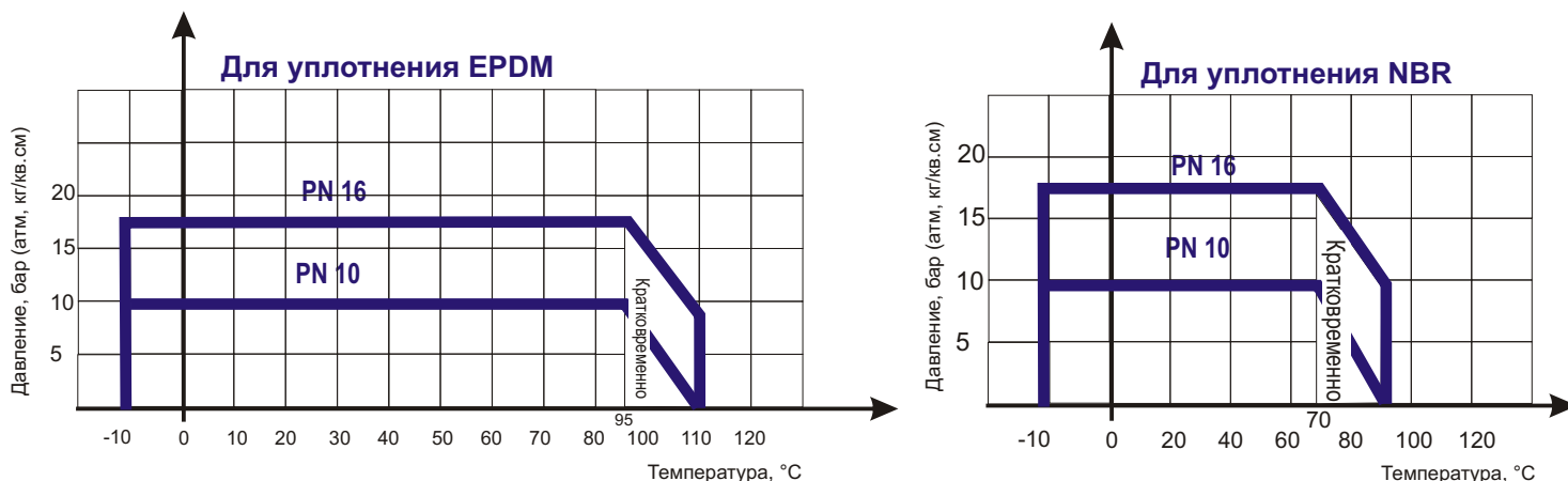
Диаграмма Давление / Температура для затвора поворотного дискового ABRA-BUV-VFzzzG DN 700-1400, PN 10 и PN 16
