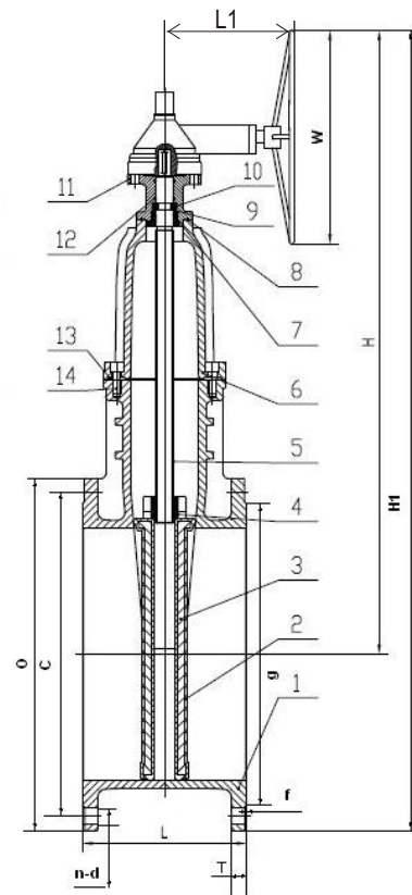
Чертеж габаритный задвижки клиновой с обрезиненным клином и невымываемым штоком ABRA-A4016XXXG DN 350-1000 чугунной ABRA-A4010XXXG DN 350-1000 чугунной (размеры в таблице ниже)
