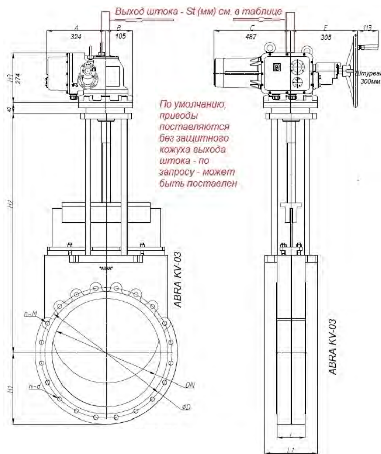
Габаритные размеры, рабочие давления и температуры, вес и Kv (таблица) задвижки шиберной ABRA-KV-03. Размеры в мм.
