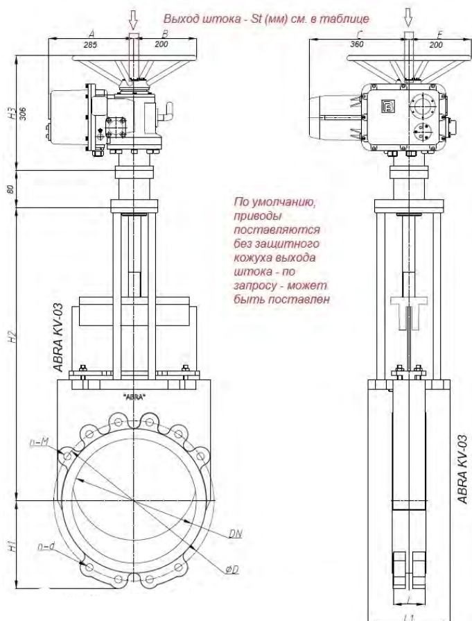
Габаритные размеры, рабочие давления и температуры, вес и Kv (таблица) задвижки шиберной ABRA-KV-03. Размеры в мм.
