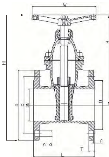
Чертеж габаритный задвижки чугунной с обрезиненным клином и невыдвижным штоком ABRA-A-4010 (размеры в таблице ниже):
