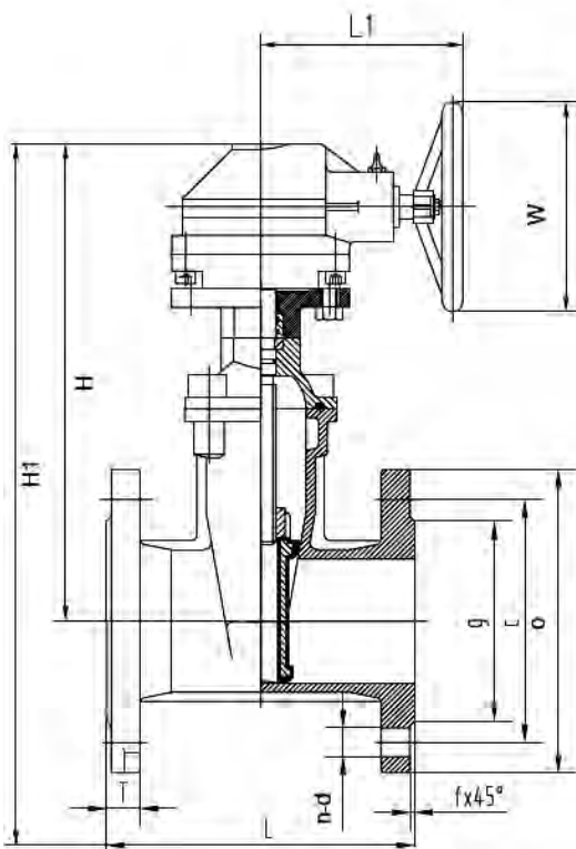
Чертеж габаритный задвижки клиновой с обрезиненным клином и невымываемым штоком ABRA-A4016XXXG DN 40-150 чугунной ABRA-A4010XXXG DN 200-300 чугунной (размеры в таблице ниже)
