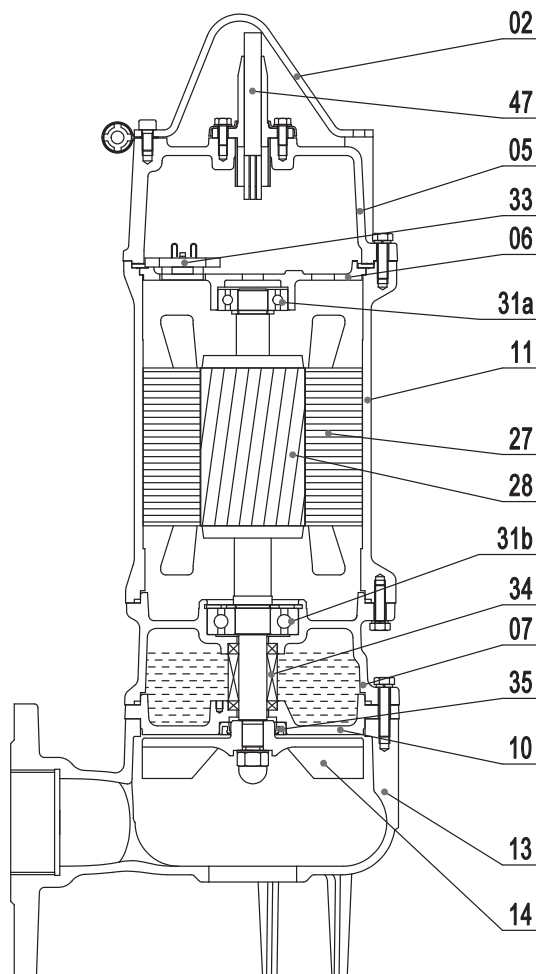
3-фазное исполнение
