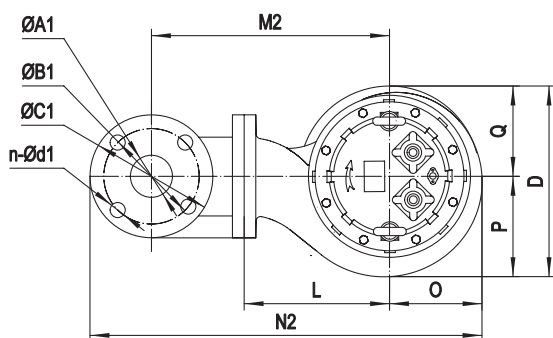
Размеры напорного патрубка насоса
