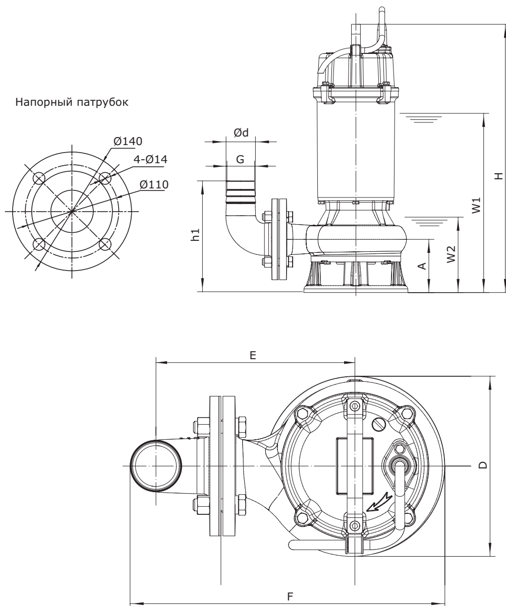
Рис. 19 Габаритные размеры насосов VSL.50.075.2.5.0D.T и VSL.50.15.2.5.0D.T
