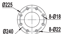
Фланец переходника DN100/ DN150 PN6/ PN10 со стороны автоматической трубной муфты (входит в комплект поставки насоса)
