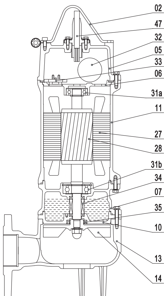
1-фазное исполнение
