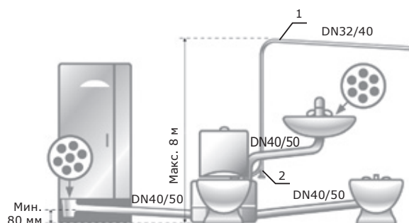
Рис. 32 Рекомендуемая схема монтажа напорного трубопровода
