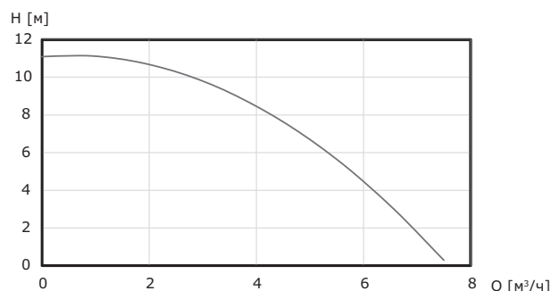
Рис. 34 Рабочие характеристики CITILIFT TRIO
