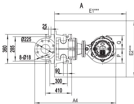
Фланец переходника DN100/ DN150 PN6/ PN10 со стороны автоматической трубной муфты (входит в комплект поставки насоса)
