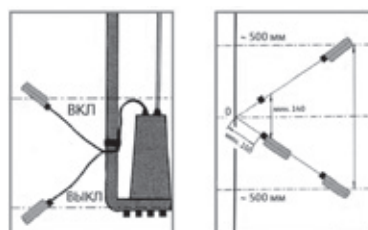
Рис. 27 Монтаж поплавкового выключателя KR1, KR1S
