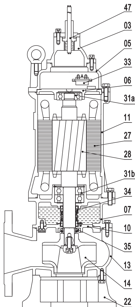
4,0–5,5 кВт
