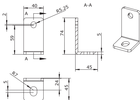
Рис. 37 Уголок для крепления резервуара установки Prolift к полу
