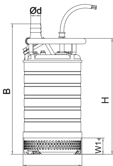
ØD 3,7–5,5 кВт
