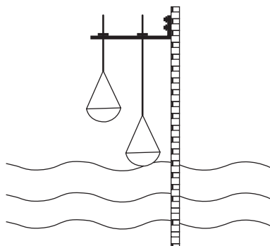
Рис. 23 Монтаж поплавкового выключателя MS1
