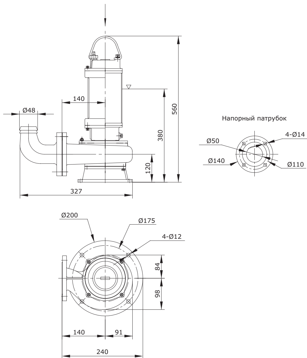
Рис. 20 Габаритные размеры VSL.50.11.2.5.0D.T
