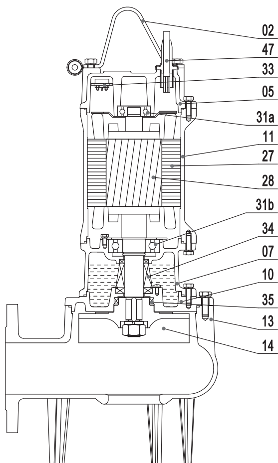
VSV 1,5–3,7 кВт
