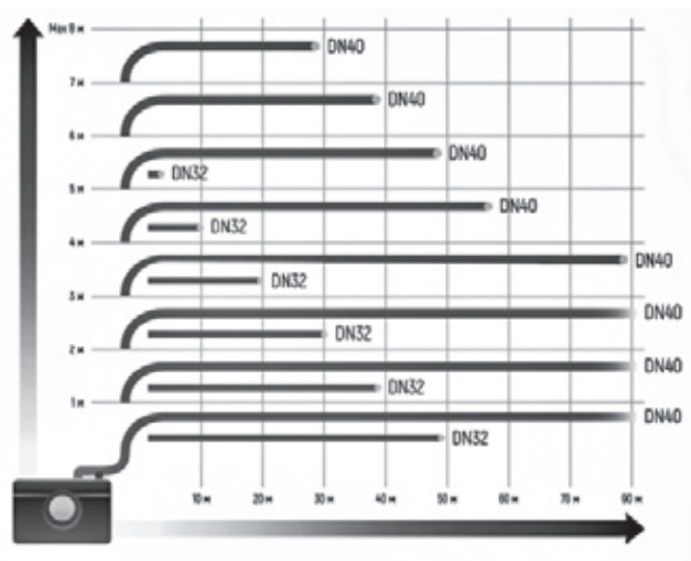
Рис. 33 Максимальная длина напорного трубопровода
