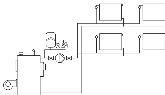
Рис. 36 Двухтрубная система отопления
