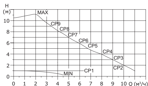
Рис. 55 Кривые режима управления с постоянным значением давления (на примере MEGA 40-10F)
