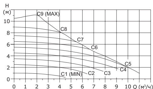
Рис. 56 Кривые режима управления при фиксированной частоте вращения (на примере MEGA 40-10F)
