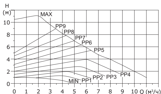
Рис. 54 Кривые режима управления пропорционального изменения давления (на примере MEGA 40-10F)
