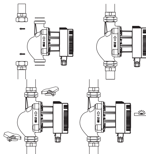
Рис. 50 Монтаж насоса (на примере MEGA)
