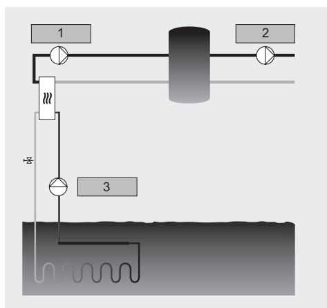
Рис. 67 Функциональная схема системы отопления на основе использования теплоты грунта
