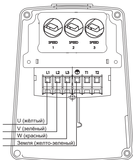
Рис. 32 Модуль переключения частоты вращения
