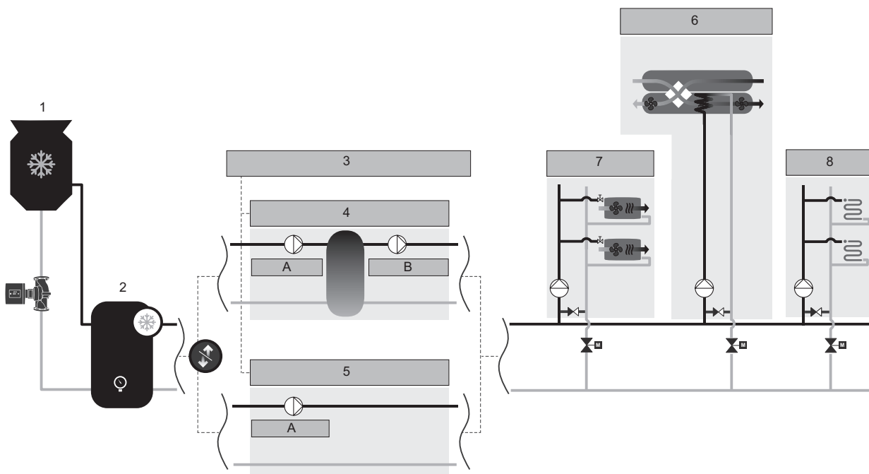
Рис. 66 Функциональная схема системы охлаждения в коммерческом здании
