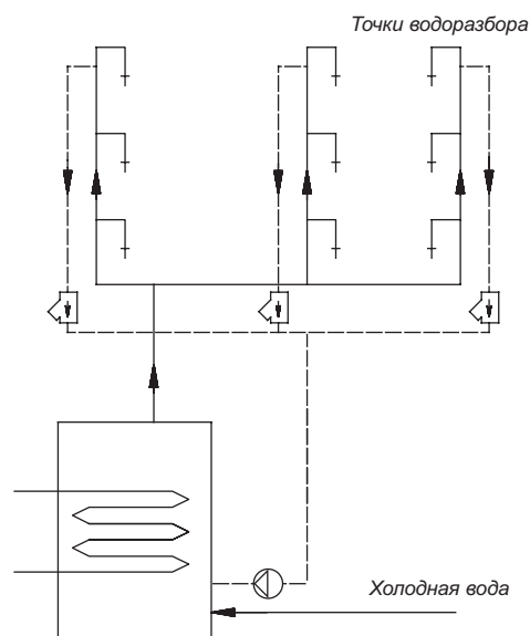
Рис. 21 Многоконтурная схема рециркуляции горячей воды
