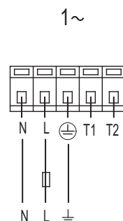
Рис. 29 Схема подключения однофазного насоса
