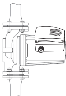
Рис. 27 Положение вала электродвигателя
