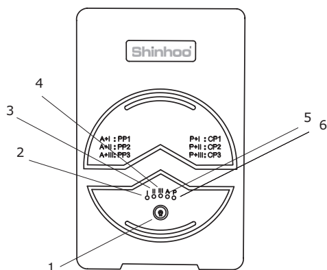
Рис. 58 Элементы управления насоса MEGA+
