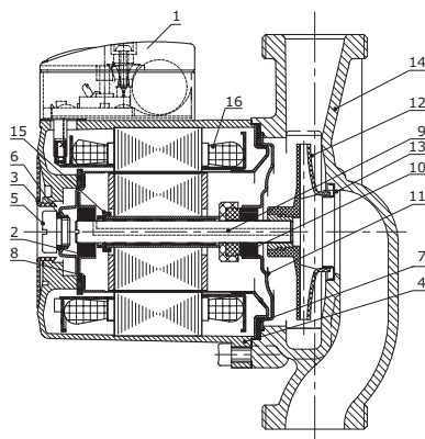
Рис. 15 Трехскоростной насос BASIC S
