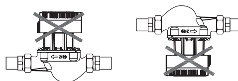
Рис. 49 Недопустимое расположение вала насоса (на примере MEGA)
