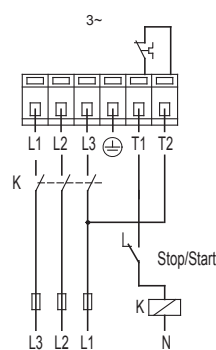
Рис. 31 Схема подключения трехфазного насоса при использовании внешнего механического пускателя ВКЛ/ВЫКЛ
