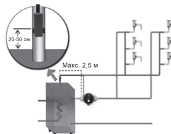
Рис. 23 Установка датчика температуры насоса INSTANT PRO
