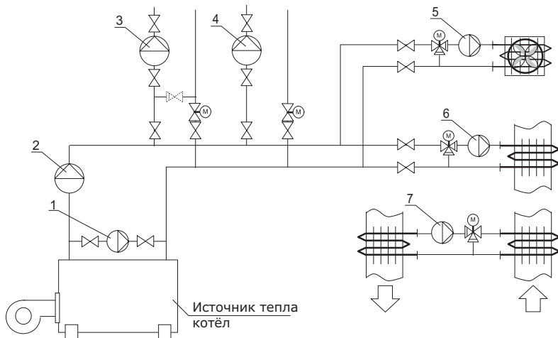
Рис. 46 Схема системы отопления
