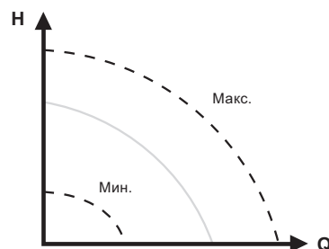
Рис. 69 Максимальная и минимальная характеристики
