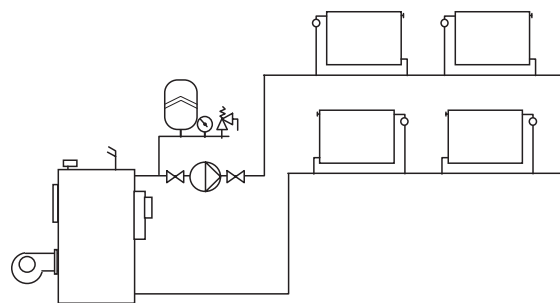
Рис. 35 Однотрубная система отопления
