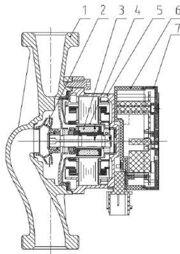
Рис. 42 Насос MASTER S
