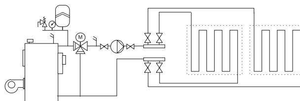
Рис. 37 Система «тёплых полов»
