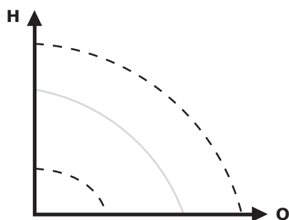
Рис. 73 Режим эксплуатации в соответствии с постоянной характеристикой
