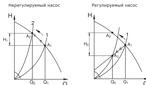
Рис. 38 Изменение положения рабочей точки регулируемого и нерегулируемого насоса
