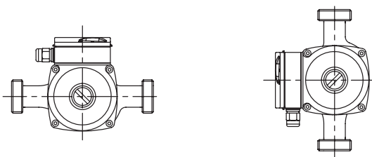
Рис. 16 Возможная ориентация вала
