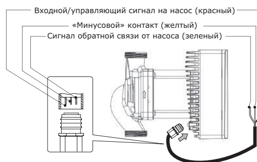
Рис. 61 Схема подключения ШИМ-сигнала MEGA+
