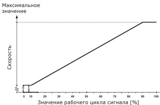
Рис. 40 Профиль управляющего ШИМ-сигнала для режима PWM2
