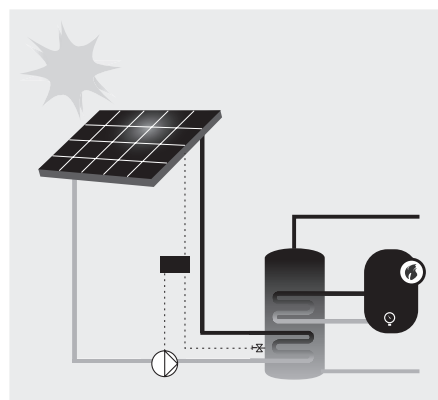
Рис. 68 Функциональная схема системы отопления на основе использования энергии солнца
