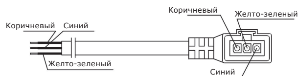
Рис. 52 Электроподключение MEGA+
