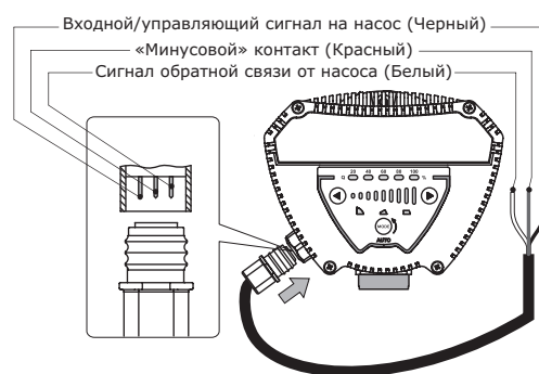
Рис. 60 Схема подключения ШИМ-сигнала MEGA
