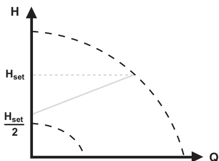
Рис. 70 Регулирование по пропорциональному давлению
