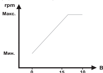
Рис. 76 Зависимость скорости насоса от установленного значения сигнала 4-20 мА
