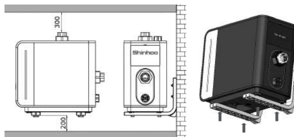
Рис. 8 Соединение комплекта настенного монтажа с установкой AQUAMASTER
