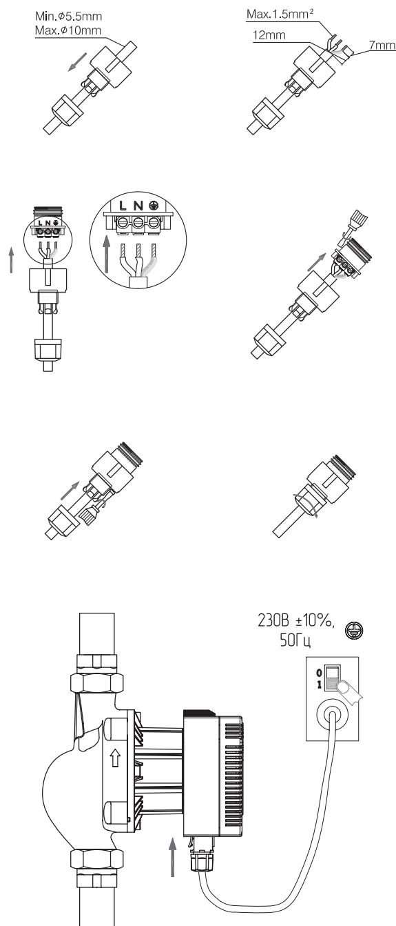
Рис. 51 Электроподключение MEGA
