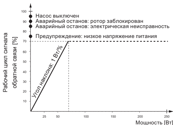
Рис. 41 Профиль ШИМ-сигнала обратной связи
