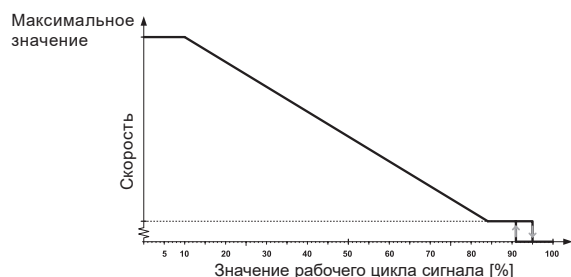
Рис. 39 Профиль управляющего ШИМ-сигнала для режима PWM1
