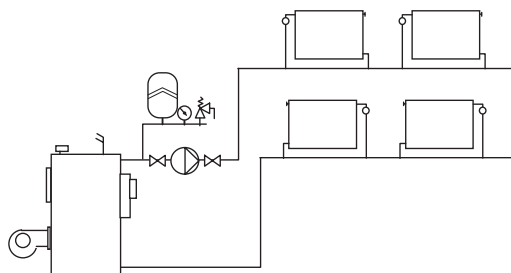
Рис. 12 Однотрубная система отопления
