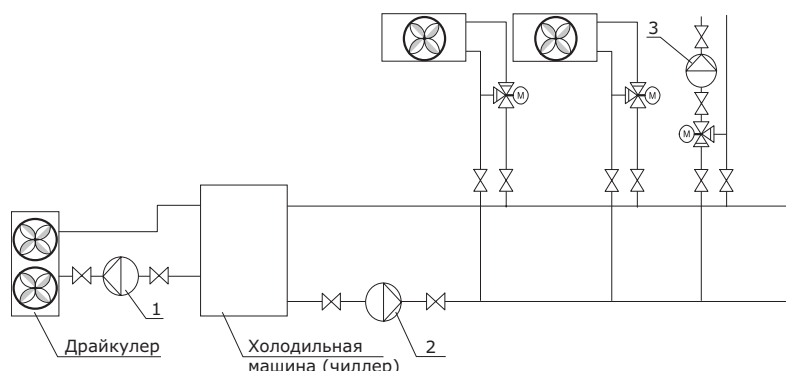
Рис. 26 Схема системы охлаждения и кондиционирования воздуха
