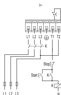
Рис. 30 Схема подключения трехфазного насоса при использовании внешнего электромагнитного пускателя ВКЛ/ВЫКЛ
