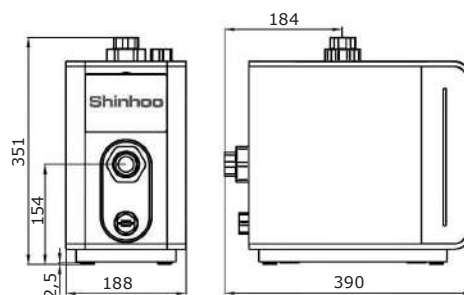
Рис. 10 Габаритный чертеж AQUAMASTER
