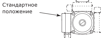
Рис. 17 Возможное положение блока управления для системы отопления
