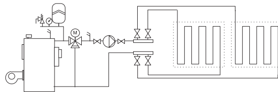
Рис. 14 Система «тёплых полов»
