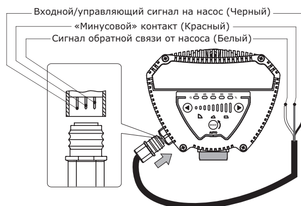
Рис. 59 Схема подключения ШИМ-сигнала
