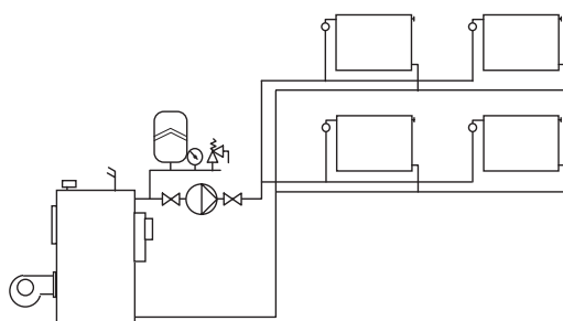
Рис. 13 Двухтрубная система отопления
