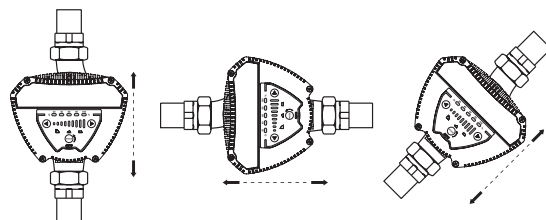
Рис. 48 Допустимое расположение вала насоса (на примере MEGA)
