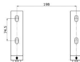
Рис. 9 Монтажные габариты комплекта настенного монтажа
