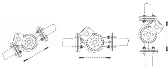
Рис. 28 Возможные положения клеммной коробки
