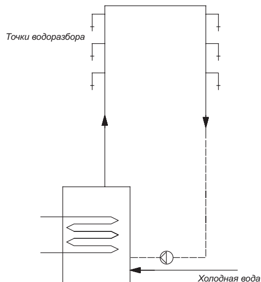
Рис. 20 Одноконтурная схема контура рециркуляции горячей воды
