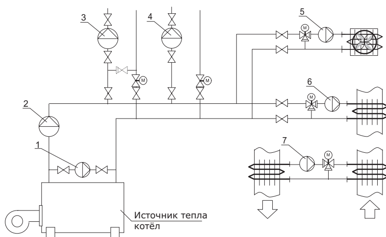
Рис. 25 Схема системы отопления и теплоснабжения
