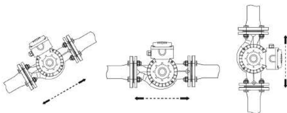
Рис. 77 Варианты монтажа
