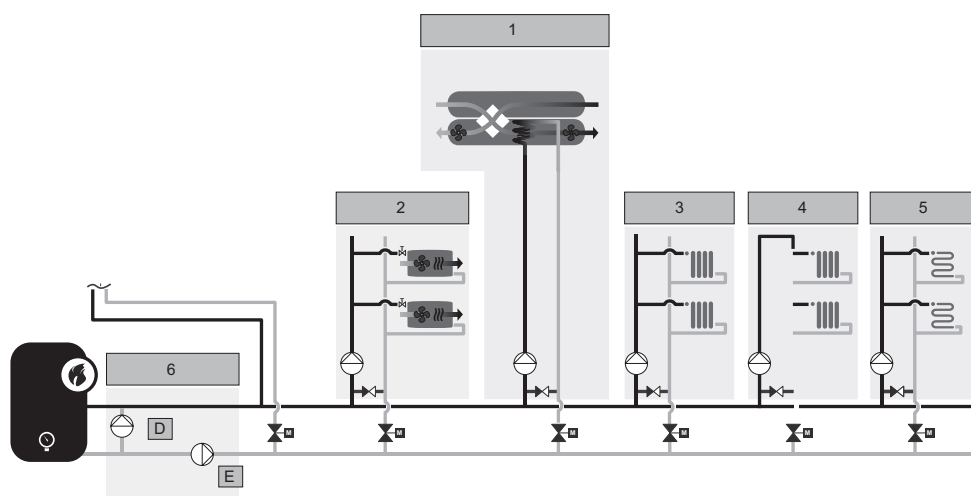
Рис. 65 Функциональная схема системы отопления в коммерческом здании
