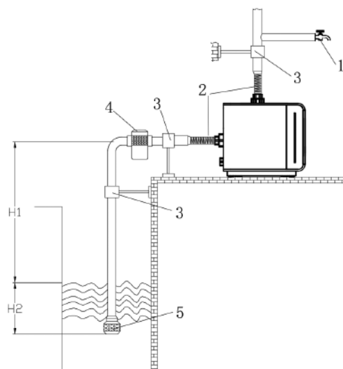
Рис. 5 Схема системы подачи воды из колодца/скважины
