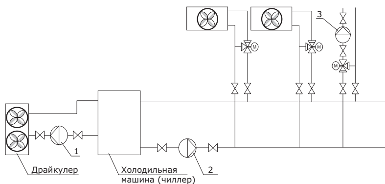
Рис. 47 Схема системы кондиционирования воздуха
