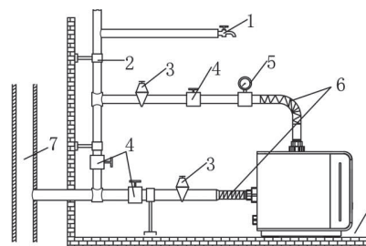
Рис. 4 Повышение давления воды из магистрального трубопровода
