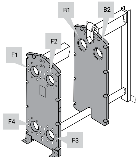
Рис. 2 – Верхнее расположение портов
