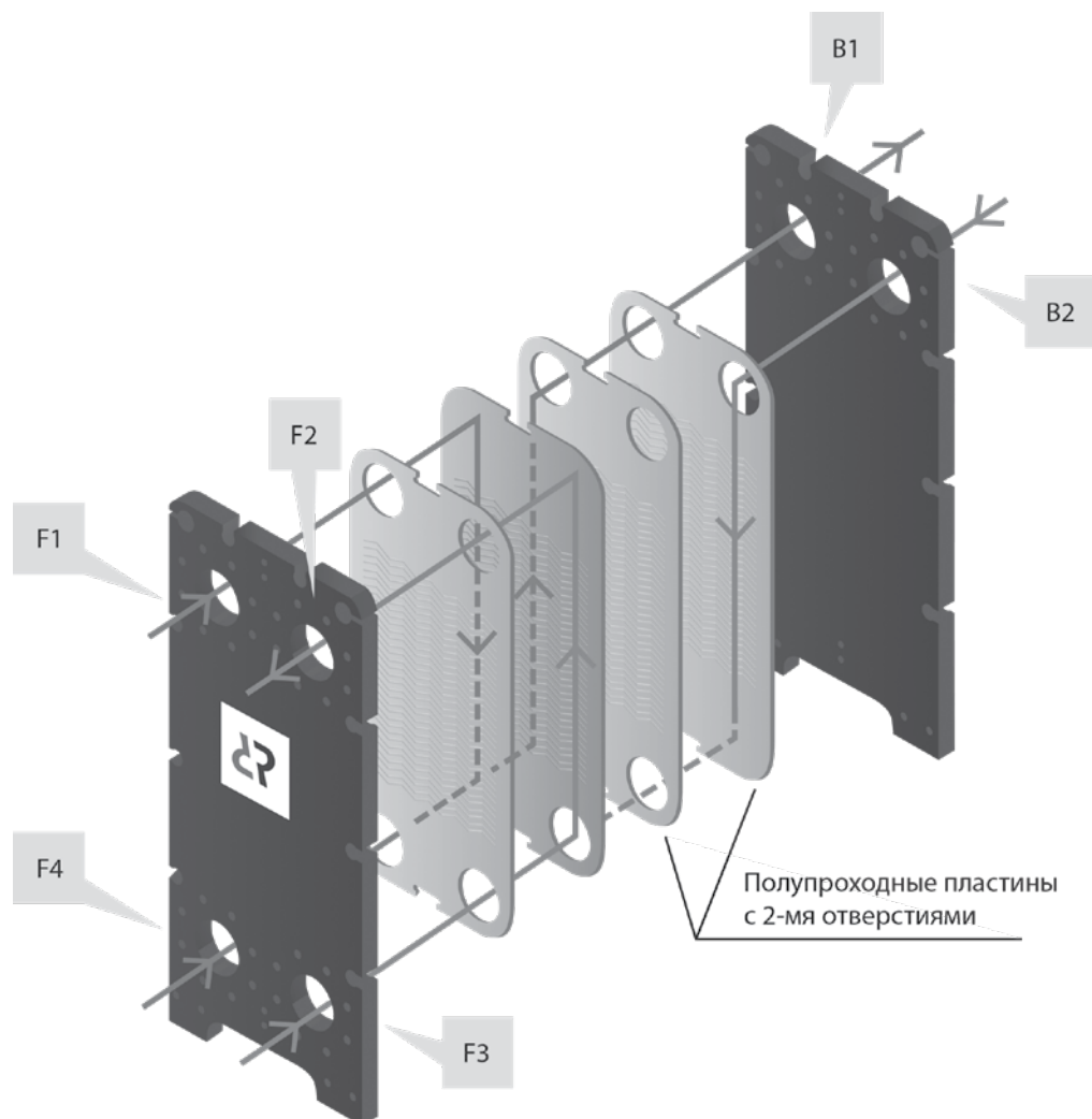
Расположение 6-ти портов на передней (F) и задней (B) плитах*
