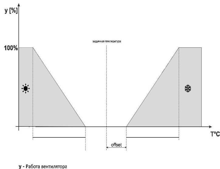
Рисунок 4: Диаграмма работы вентилятора в профиле ЕСО, ЗАЩИТА
