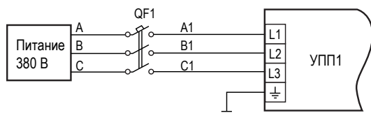
Схема подключения питания УПП1
