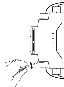
Рисунок 5.3 – Отсоединение съемных частей клемм
