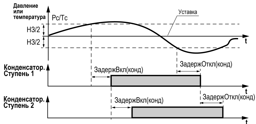
Рисунок 8.10 – Диаграмма регулирования с нейтральной зоной на примере 2-х ступеней конденсатора
