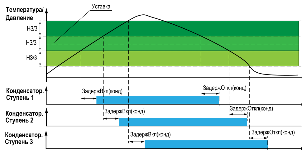
Рисунок 8.11 – Диаграмма регулирования с зонами пропорциональности на примере 3-х ступеней конденсатора
