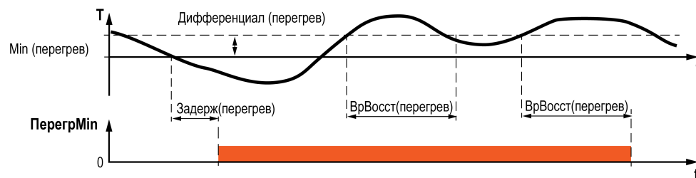
Рисунок 8.18 – Поясняющая диаграмма отработки аварии по низкому перегреву
