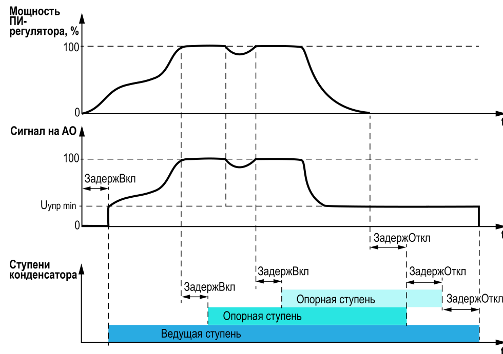
Рисунок 8.12 – Диаграмма управления конденсатором на примере 3-х ступеней, где первая управляется с помощью ПЧ
