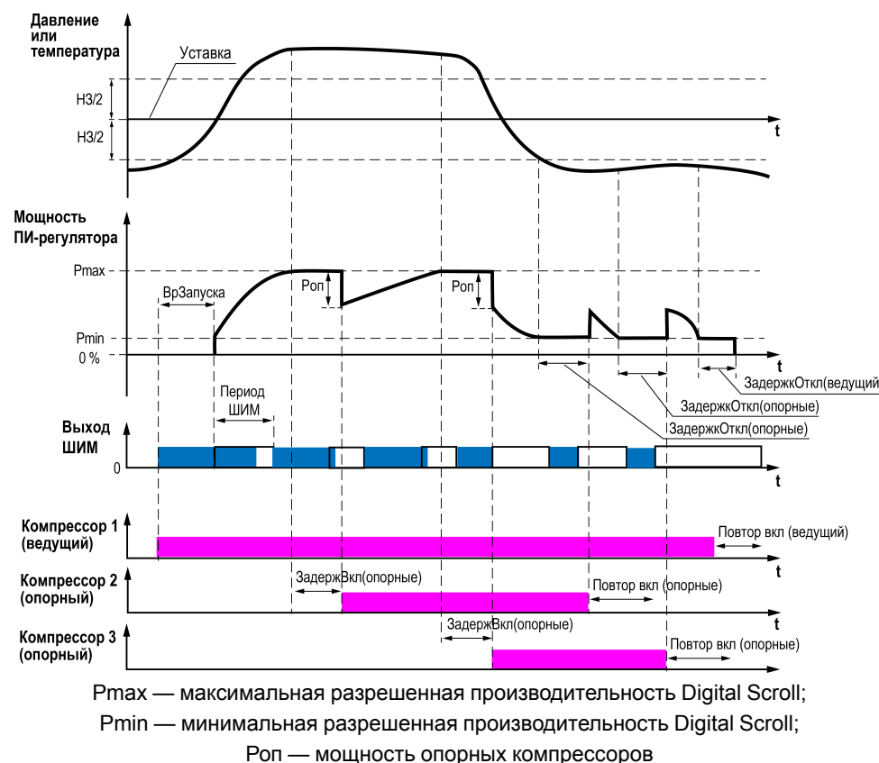
Рисунок 8.6 – Диаграмма регулирования “Digital Scroll + одиночные компрессоры”
