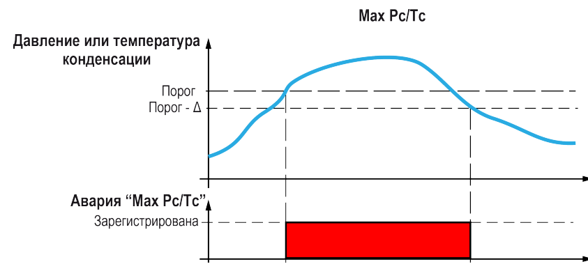
Рисунок 8.16 – Поясняющая диаграмма регистрации прибором аварии по превышению максимального порога давления или температуры конденсации
