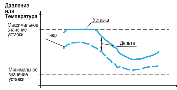
Рисунок 8.8 – Иллюстрация работы «плавающей» конденсации
