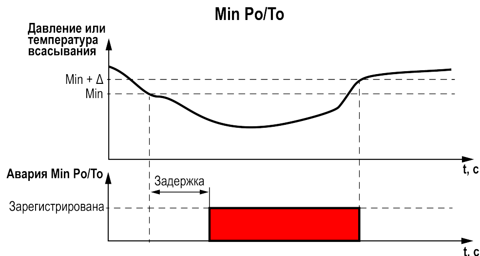
Рисунок 8.15 – Поясняющая диаграмма регистрации аварии по снижению давления (температуры) ниже допустимого порога
