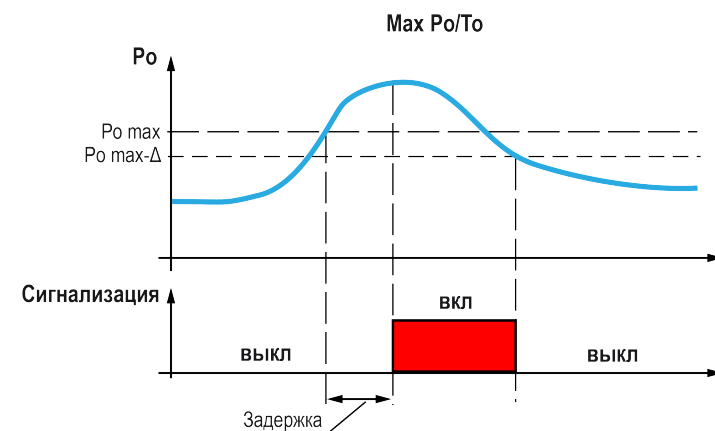
Рисунок 8.14 – Поясняющая диаграмма срабатывания сигнализации на примере превышения давлением порога P_o \max
