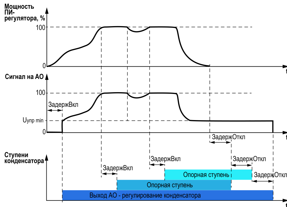
Рисунок 8.13 – Диаграмма управления конденсатором на примере 3-х ступеней, где для первой не используется дискретный выход
