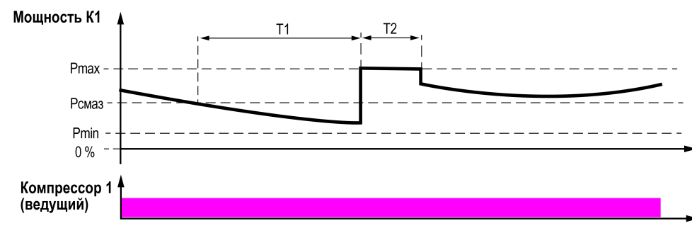
Рисунок 8.7 – Диаграмма работы функции смазывания Digital Scroll
