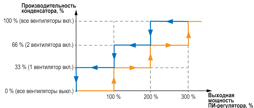
Рисунок 8.9 – Ступенчатое управление конденсатором на примере 3-х ступеней
