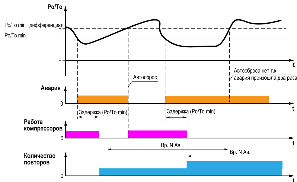
Рисунок 8.17 – Поясняющая диаграмма отработки повторения аварии Min Po/To при допустимом количестве повторений равном двум
