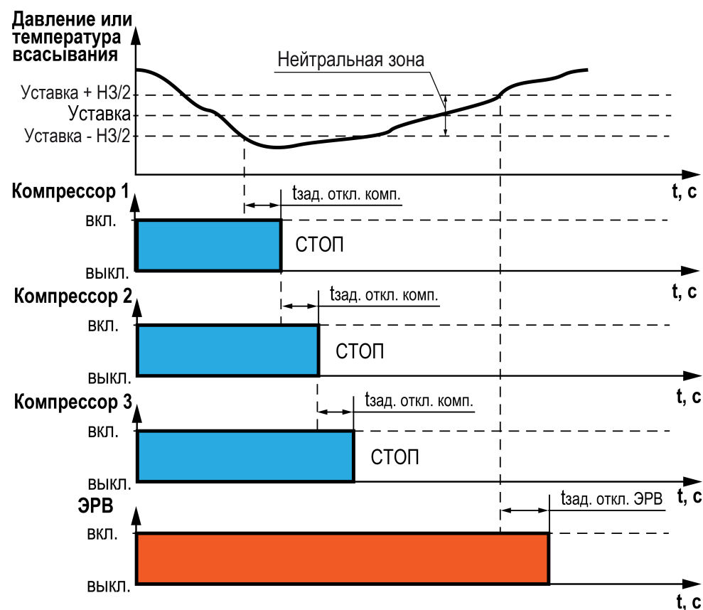
Рисунок 8.20 – Иллюстрация работы функции «Антизалив» компрессоров
