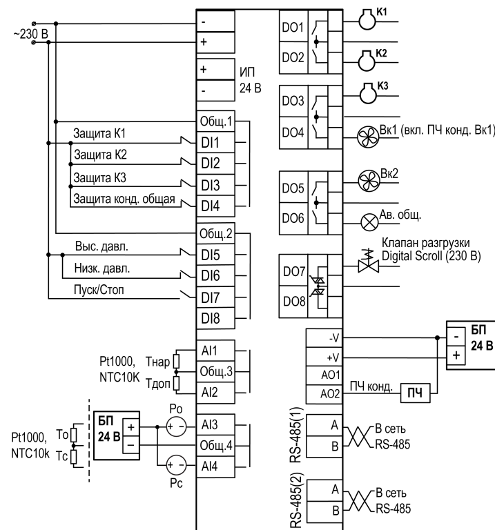
Рисунок 7.15 – Пример схемы подключения сигналов для управления ЦХМ с ведущим компрессором Digital Scroll
