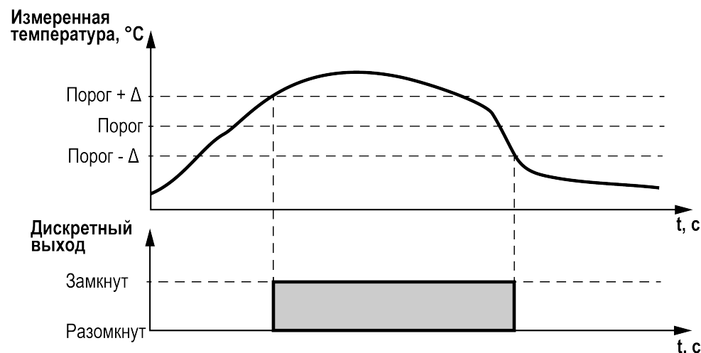
Рисунок 8.19 – Иллюстрация работы функции «Независимый термостат»
