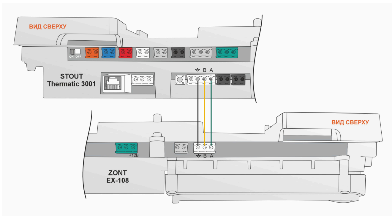
Схема подключения блока расширения EX-108
