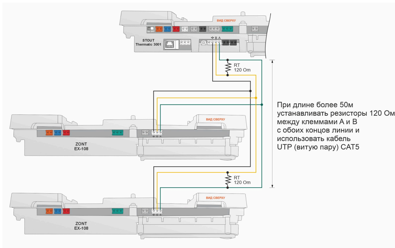
Схема подключения 2х блоков расширения EX-108
