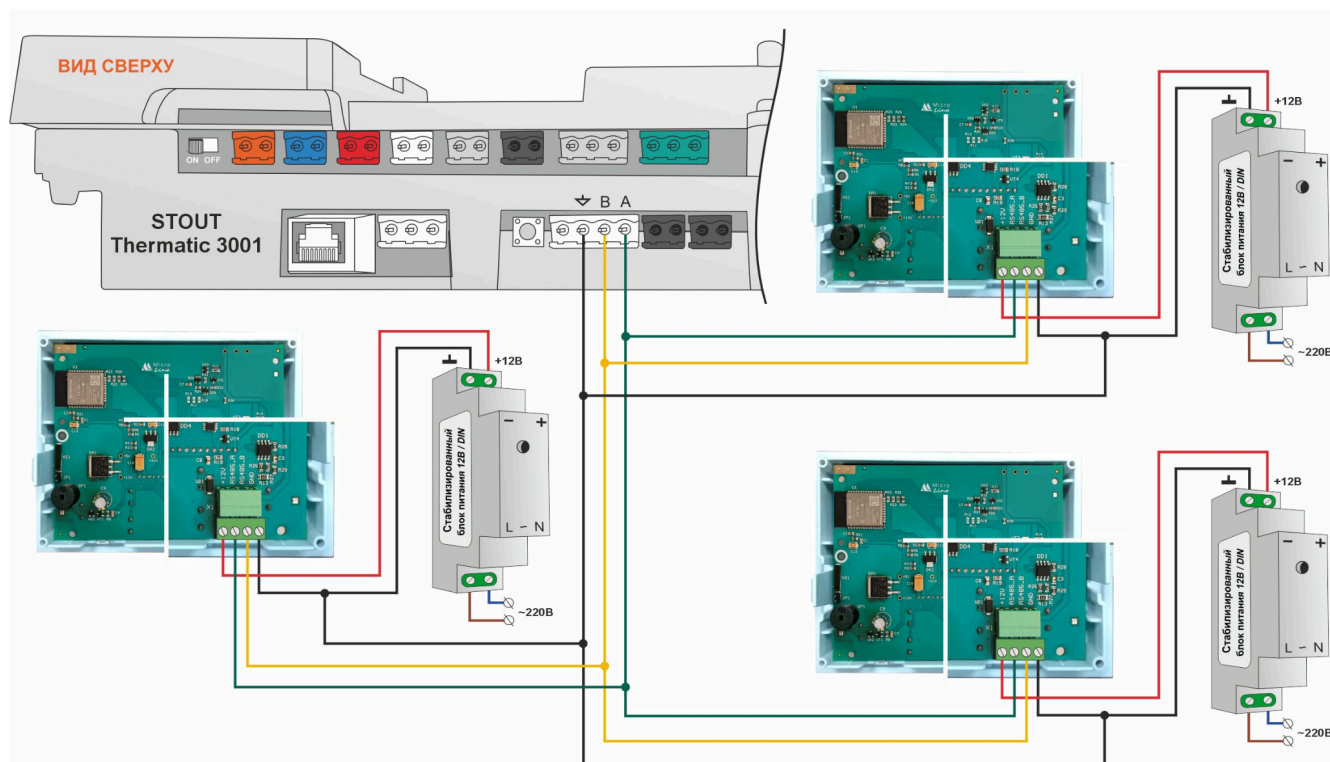
Схема подключения 3-х панелей ручного управления ZONT МЛ-753
