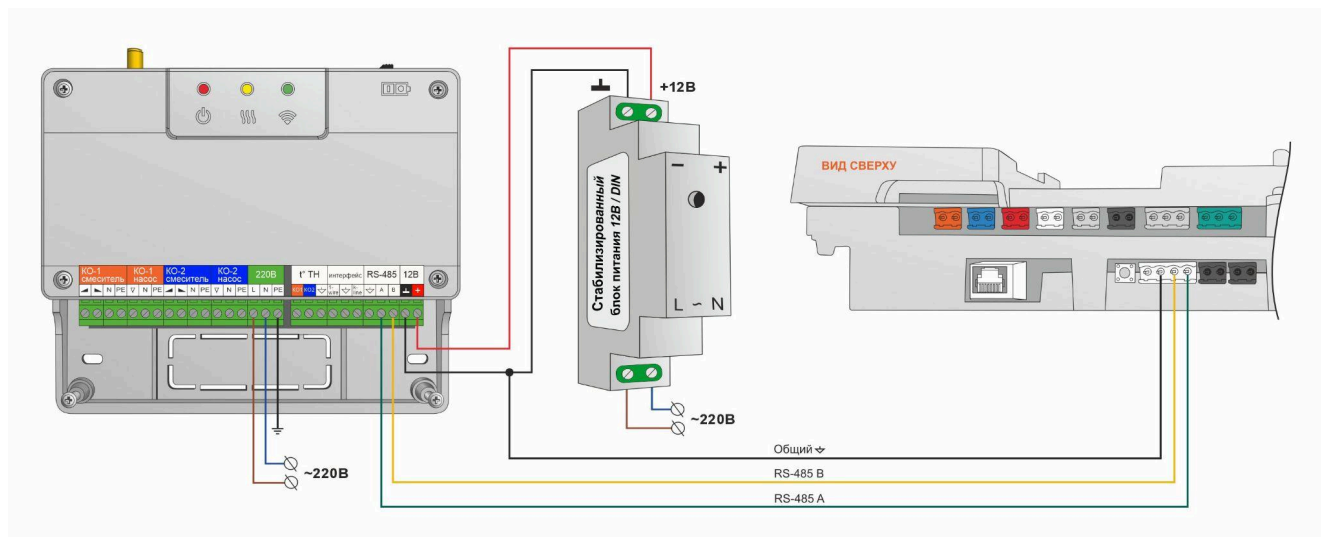
Схема подключения блока расширения EX-77
