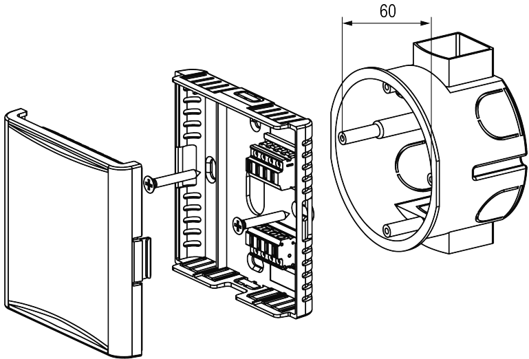
Рисунок 5.3 – Монтаж прибора в подрозетник
