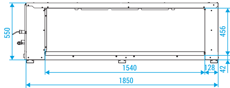
Сторона подачи воздуха в помещение
