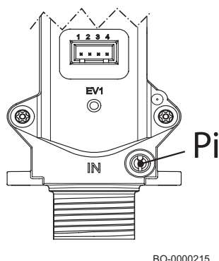
Рис. 232 Газовый клапан
