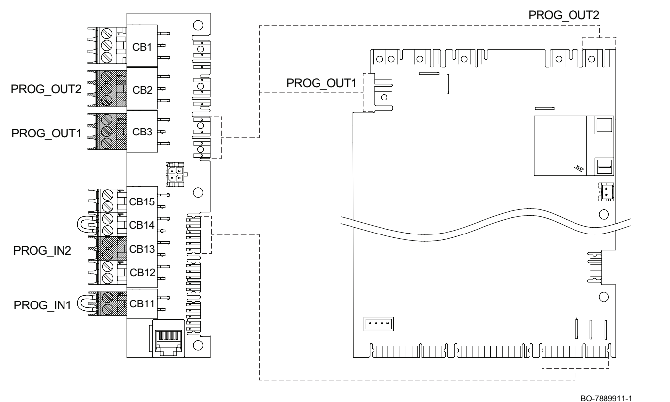
Рис. 223 Схема конфигурации программируемого выхода/входа
