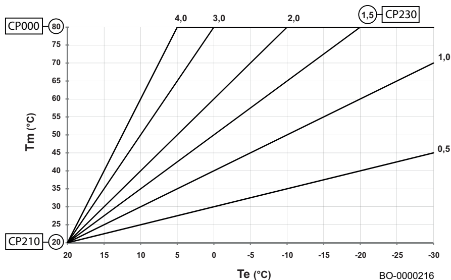
Рис. 242 Отопительный график
