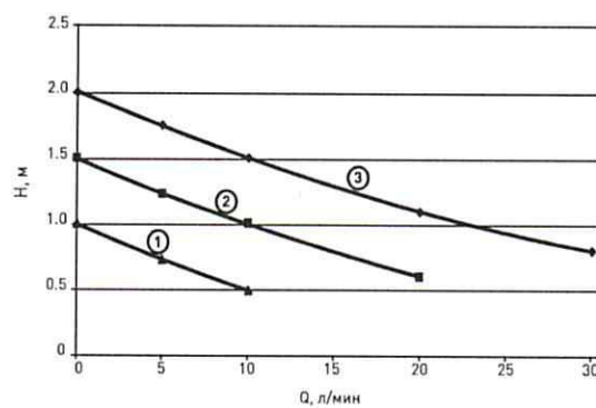
Рабочее поле для насосов WRS-25/40 и WRS-32/40
