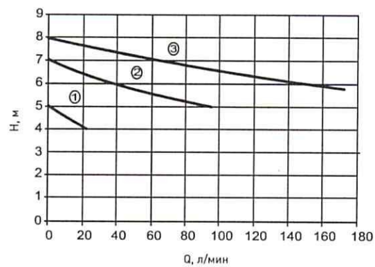
Рабочее поле для насоса WRS-25/80 и WRS-32/80
