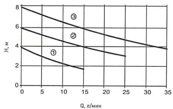
Рабочее поле для насоса WRS-25/80 и WRS-32/80
