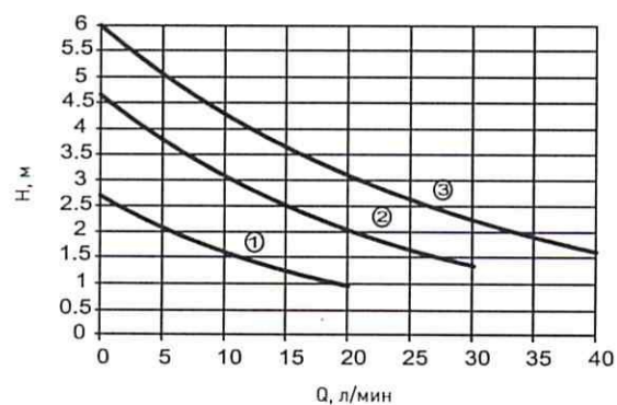
Рабочее поле для насоса WRS-25/70 и WRS-32/70
