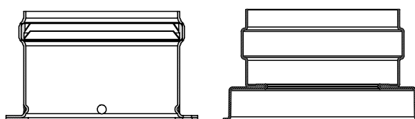
Рис. 14. Переходники раздельной системы дымоудаления \varnothing 80/80 мм.
