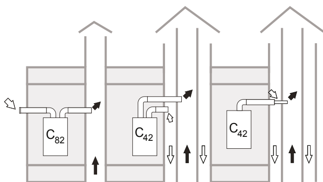
Рис. 15. Примеры систем дымоудаления собранных с помощью раздельных труб. Белой стрелкой обозначен приток воздуха, черной стрелкой поток продуктов сгорания.
