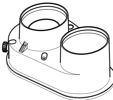
Рис. 13. Переходник с коаксиальной системы дымоудаления \varnothing 60/100 мм на раздельную \varnothing 80/80 мм.
