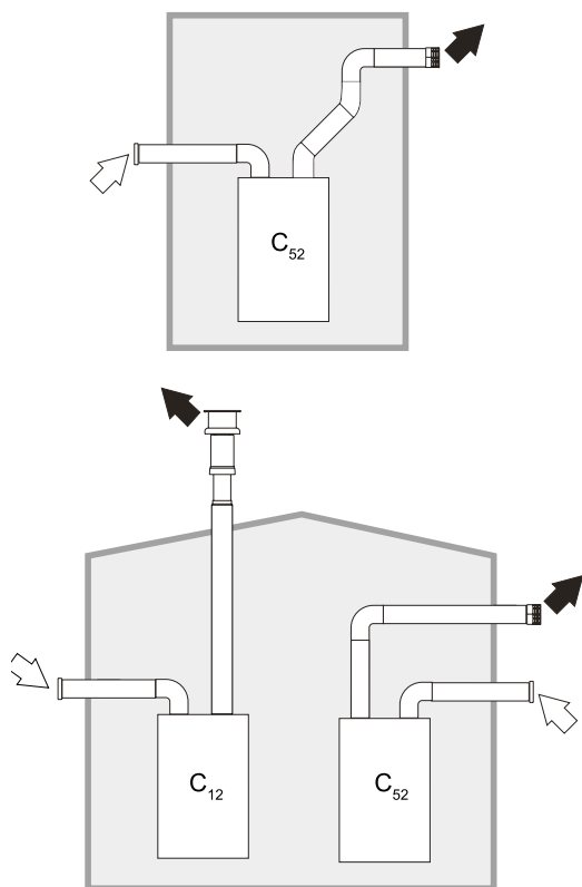
Рис. 12. Пример систем дымоудаления собранных с помощью раздельных труб. Белой стрелкой обозначен приток воздуха, чёрной стрелкой отвод продуктов сгорания
