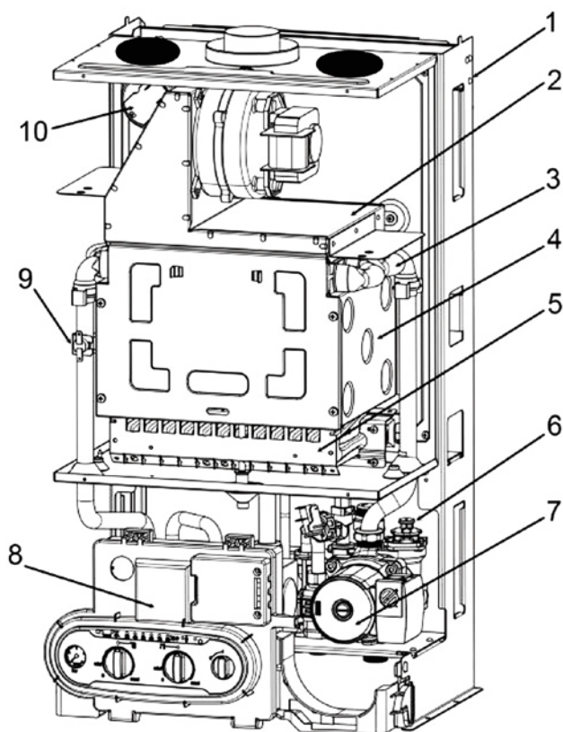
Рис. 21. Общая схема и основные элементы котла
