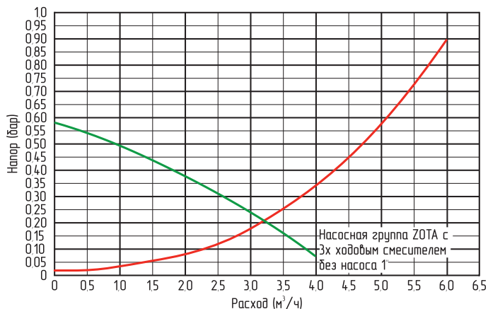
Рис.1 Гидравлические характеристики.
