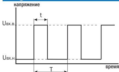
Рис.13 Характеристики ШИМ-сигнала
