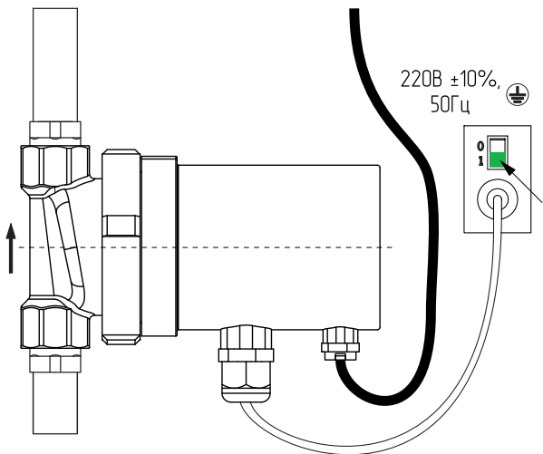
Рис.5 Электроподключение насоса
