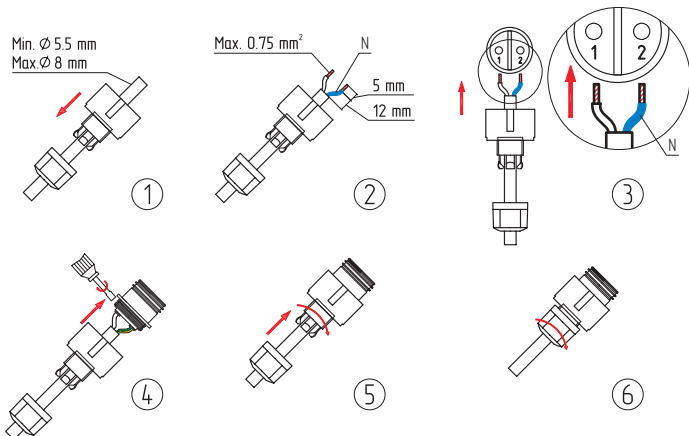
Рис.4 Схема электроподключения
