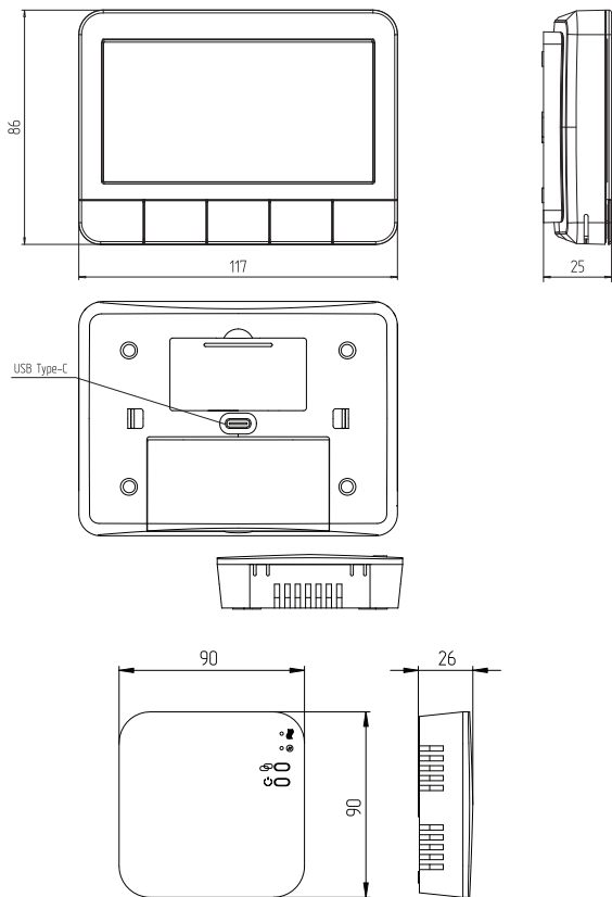
Рис. 4 Габаритные размеры терморегулятора и приемника
