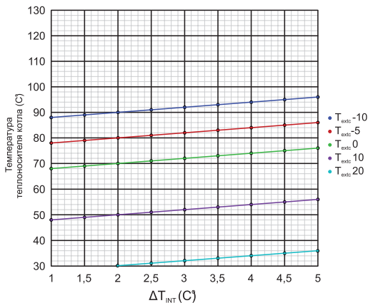
Рис. 12 Тепловая кривая с K_{comp}=4
