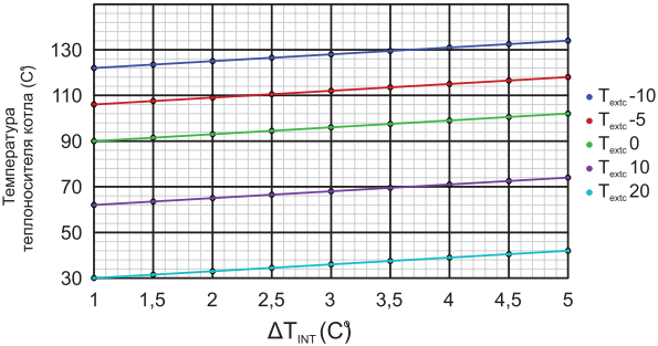
Рис. 10 Тепловая кривая с Kcomp=6 «значение по умолчанию»
