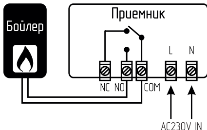
Рис. 8 Схема подключения приемника терморегулятора ZOTA ZT-20W Wi-Fi
