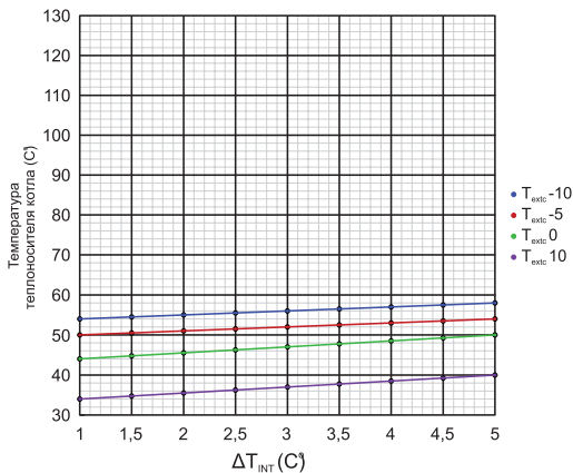
Рис. 13 Тепловая кривая с K_{comp}=2
