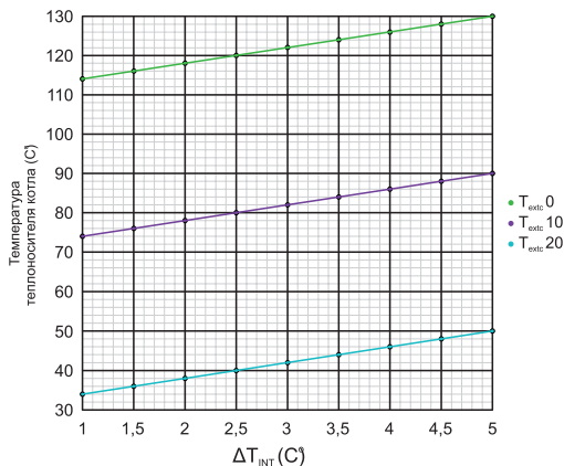
Рис. 11 Тепловая кривая с K_{comp}=8
