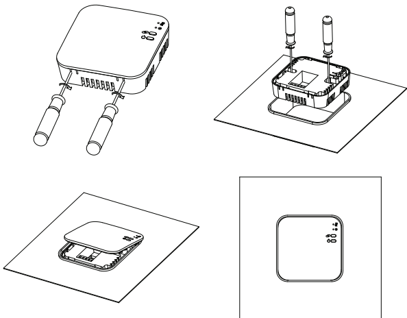
Рис. 7 Установка приемника терморегуляторов ZOTA ZT-20W Wi-Fi и ZOTA ZT-20W Wi-Fi OT+ на стену
