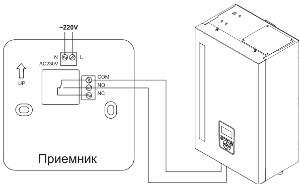
Рис.4 Схема подключения терморегулятора
