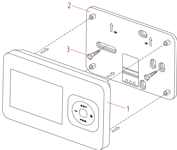
Рис.4 Установка терморегулятора
