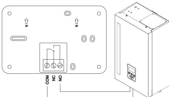
Рис.3 Схема подключения терморегулятора
