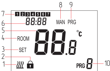
Рис.1 Индикация терморегулятора
