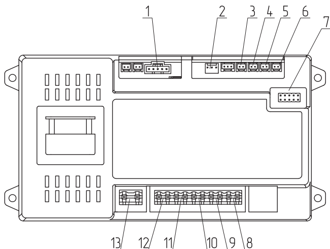
Рис.7 Подключение панели управления
