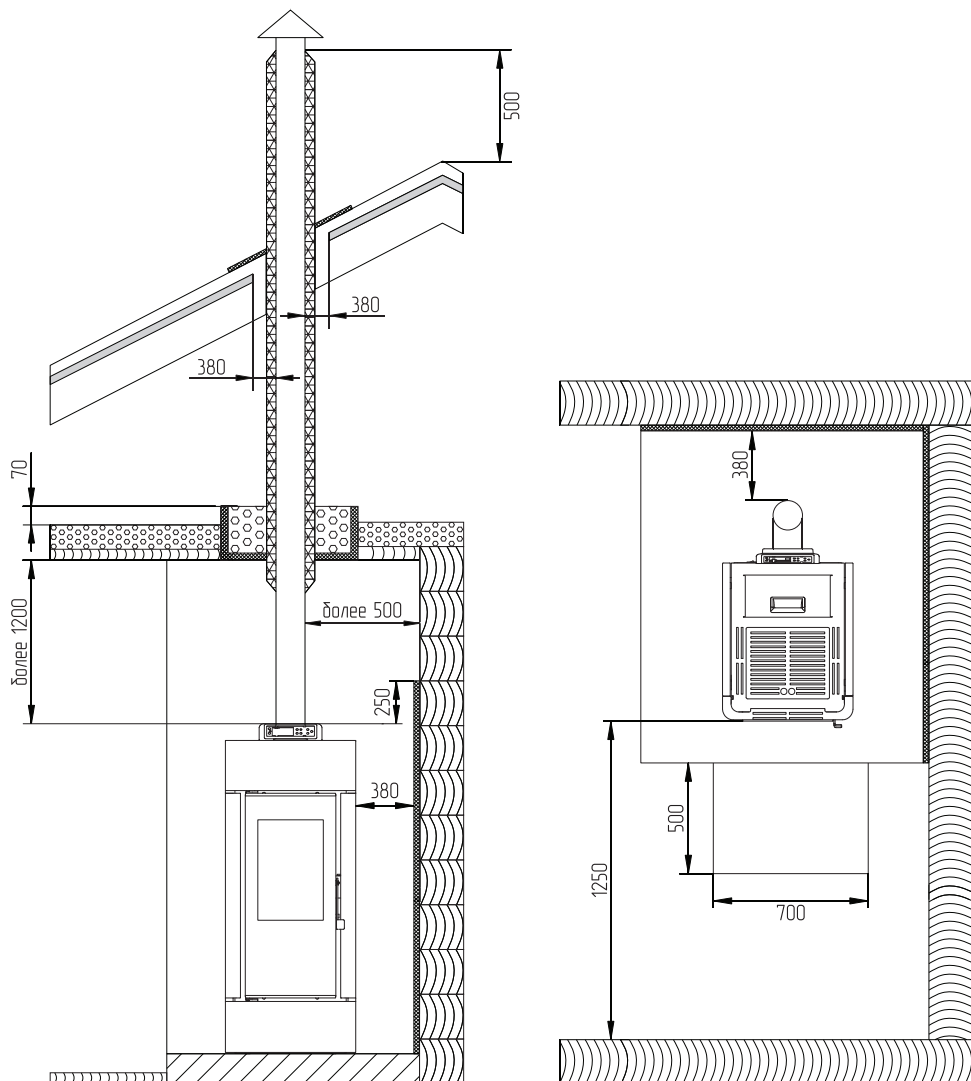
Рис.2 Схема установки камина
