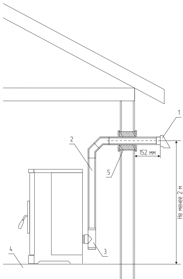
Рис.5 Подключение дымохода через стену
