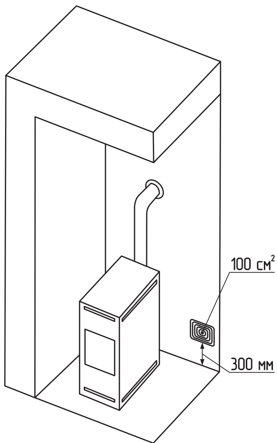
Рис.3 Расположение приточной вентиляции
