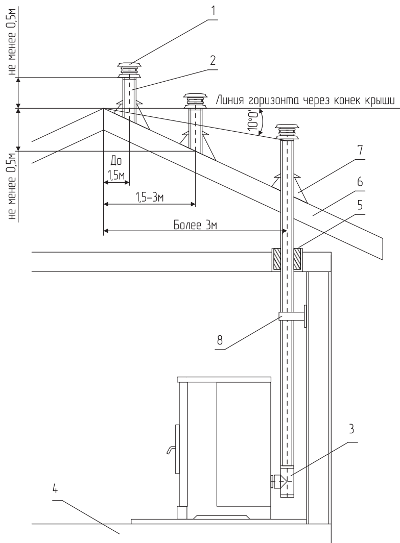
Рис.6 Подключение дымохода через крышу
