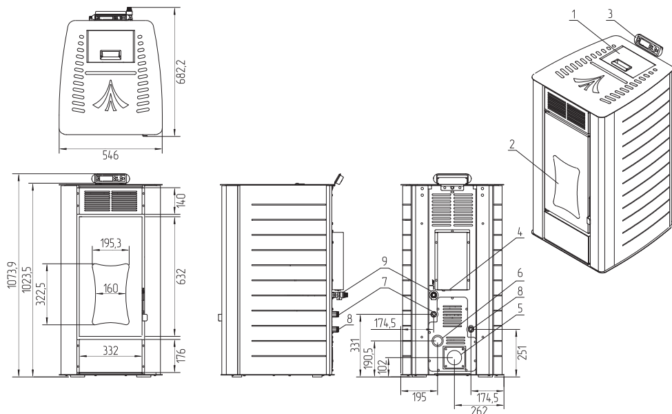
Рис.1 Устройство камина WD18H30
