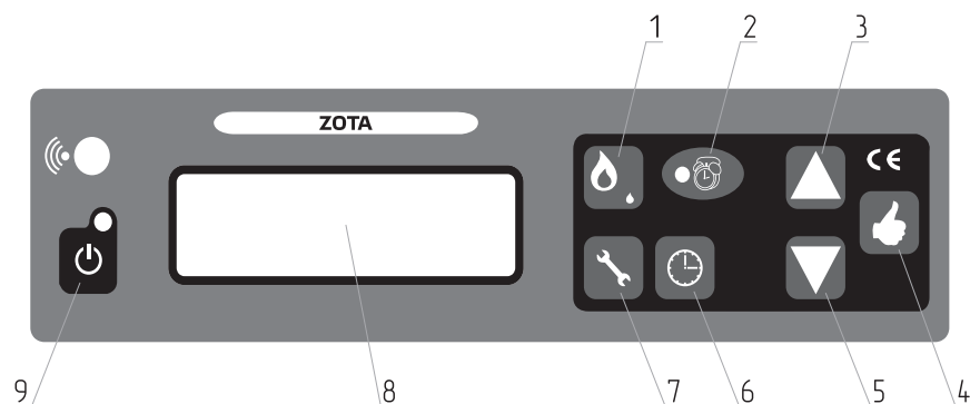
Рис.11 Устройство панели управления
