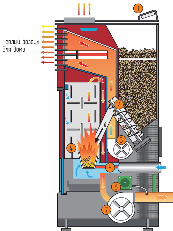
Рис.5 Функциональная схема камина
