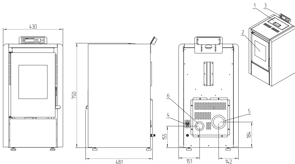
Рис.3 Устройство камина А6Н13
