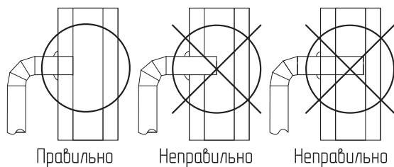
Рис.8 Подключение дымоотводящей трубы к кирпичному дымоходу
