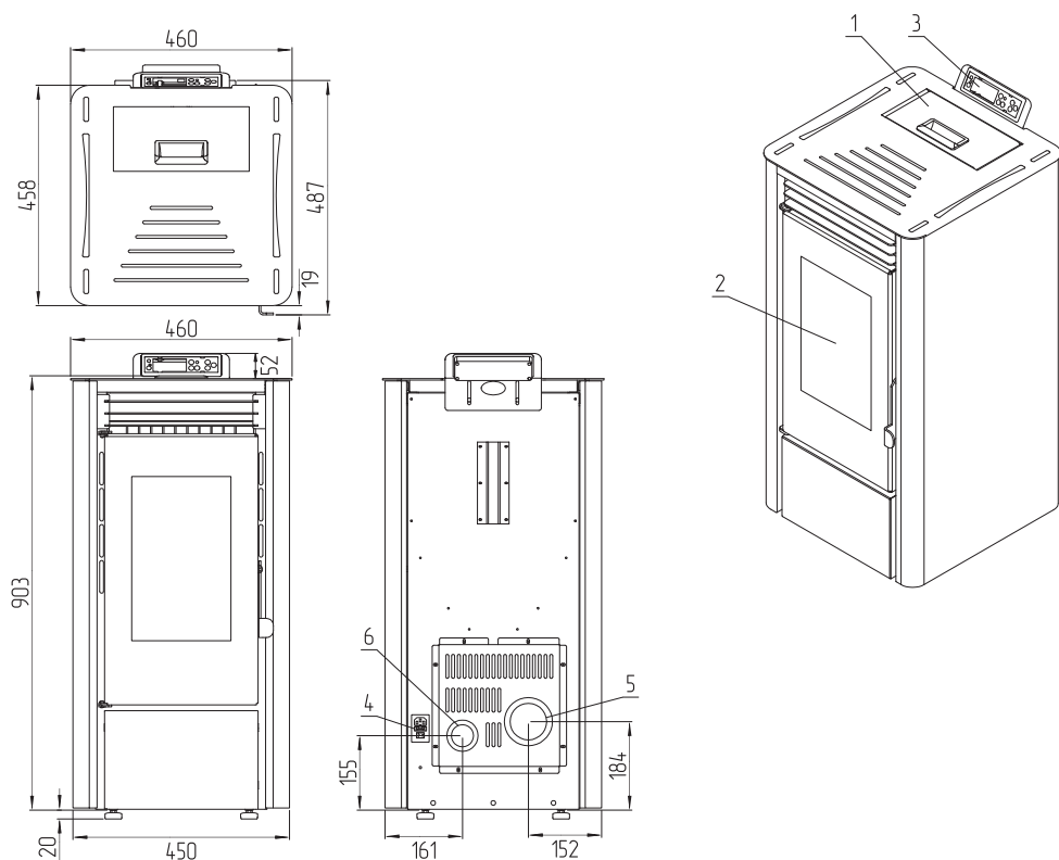
Рис.2 Устройство камина А9Н20
