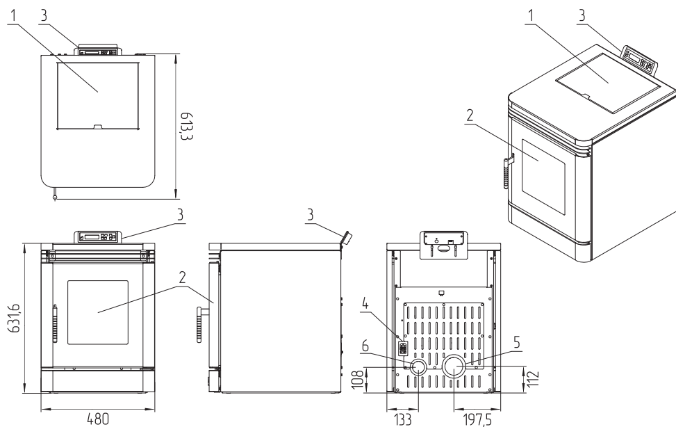
Рис.4 Устройство камина В6Н22
