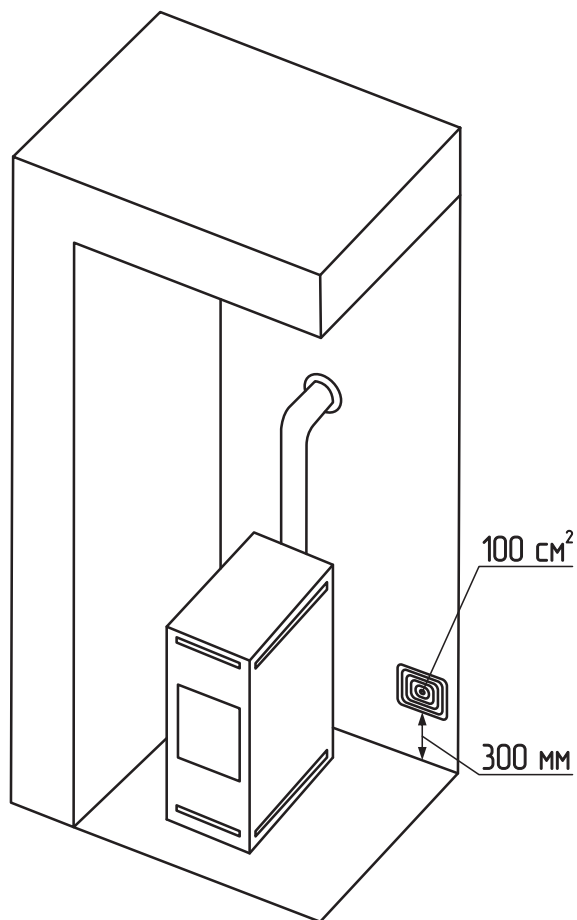
Рис.7 Расположение приточной вентиляции
