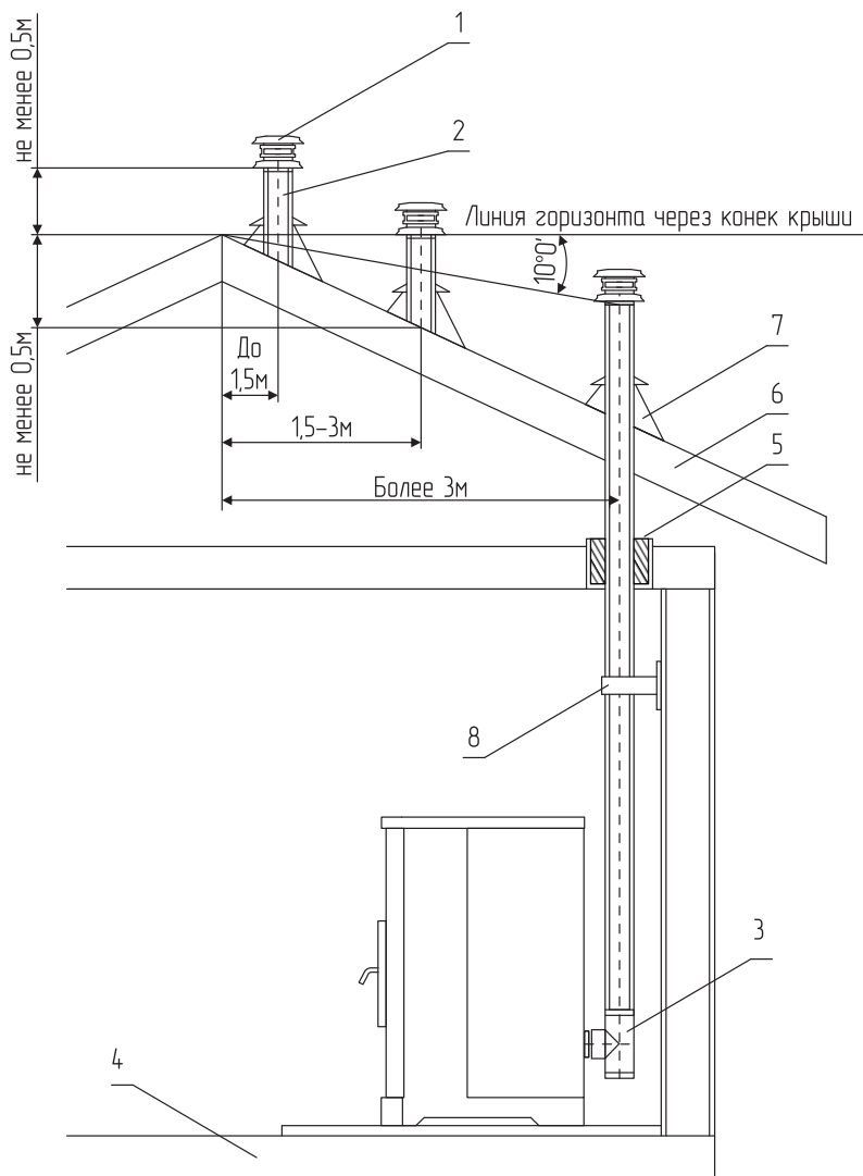
Рис.10 Подключение дымохода через крышу
