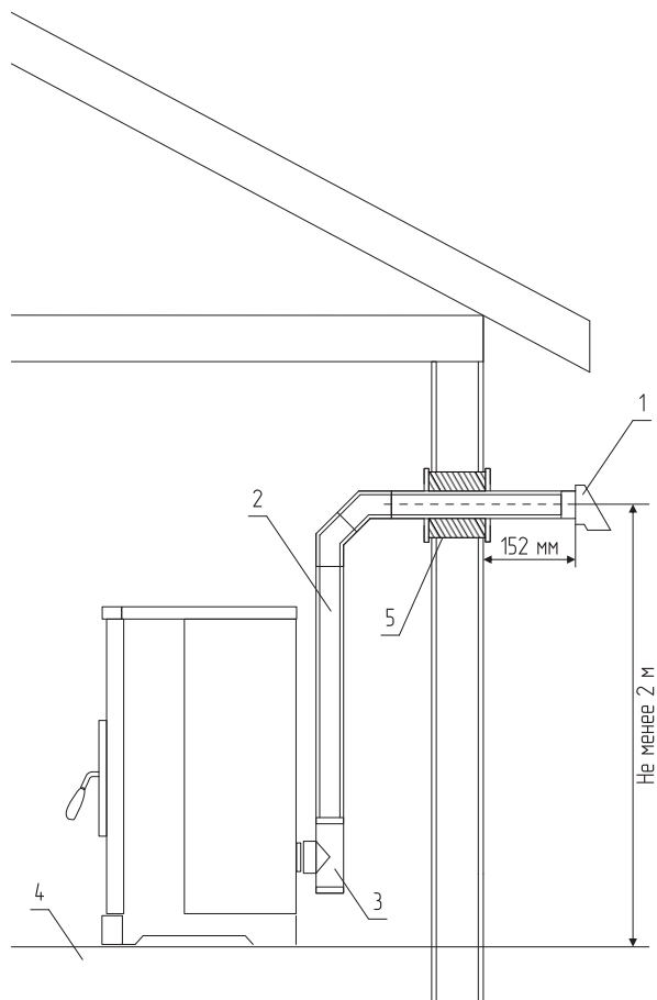
Рис.9 Подключение дымохода через стену
