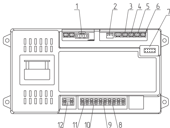
Рис.11 Подключение панели управления
