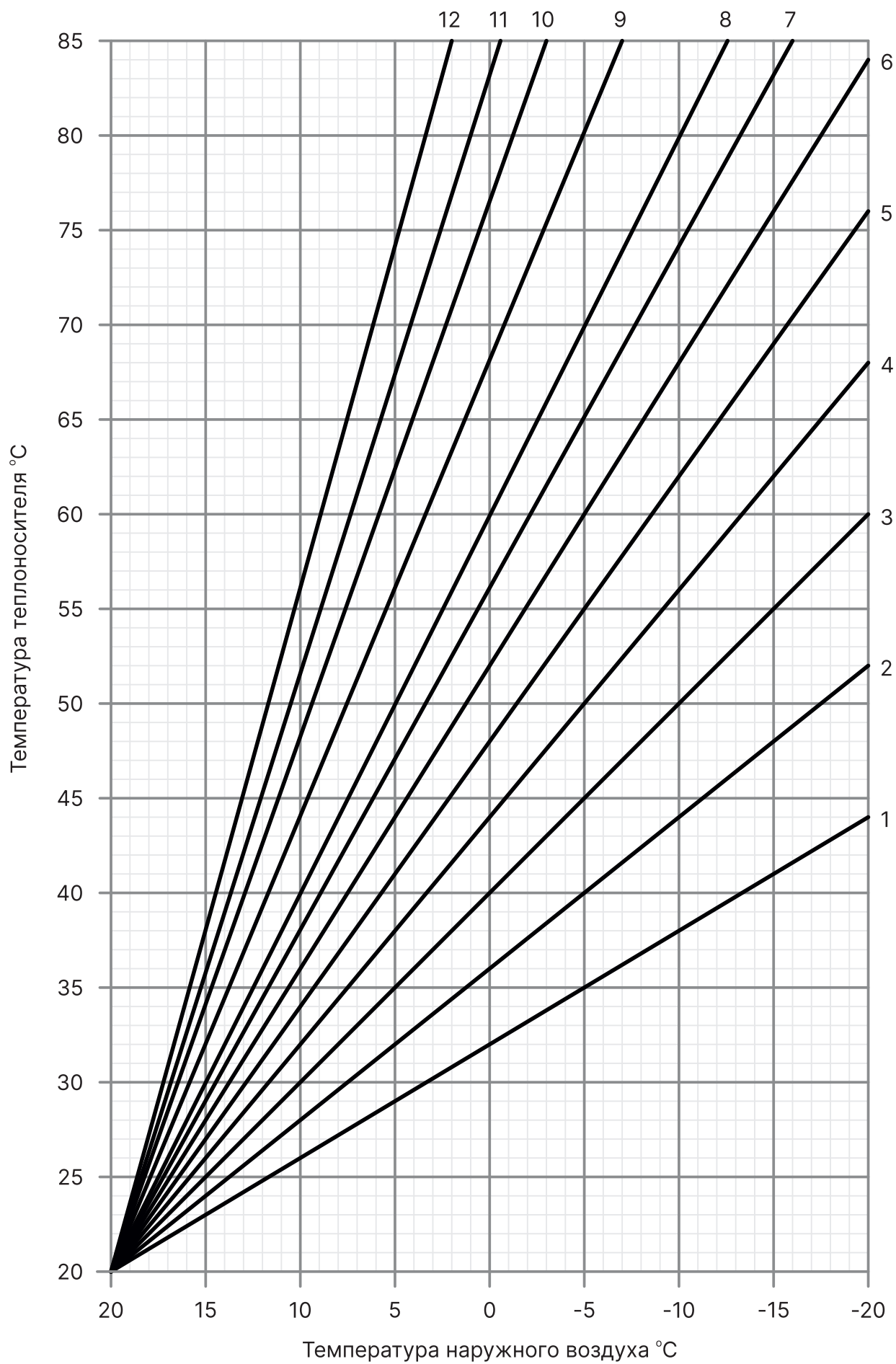
Рис. 28 Графики погодозависимого регулирования
