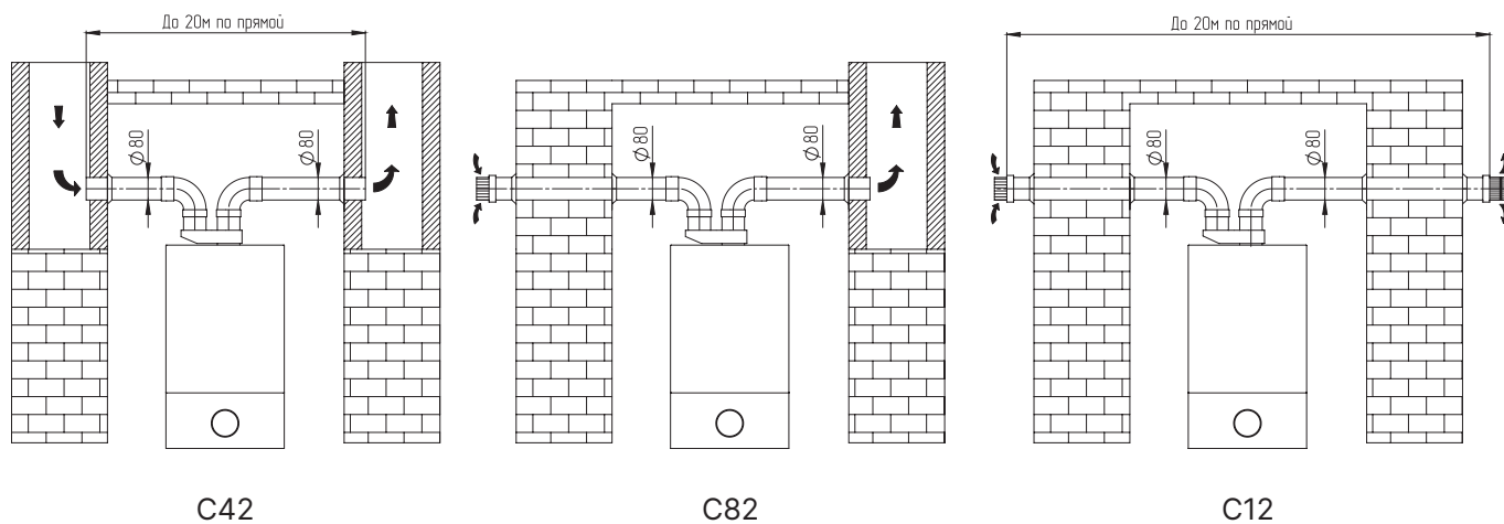
Рис. 20 Варианты монтажа раздельной системы дымохода горизонтально
