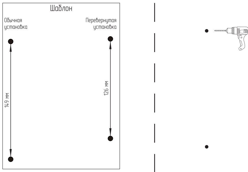
Рис.3 Монтажный шаблон
