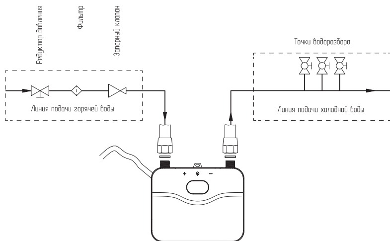
Рис.7 Подключение системы водоснабжения (перевернутая установка)
