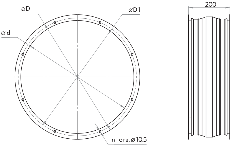
Гибкая вставка «В» типа «фланец-фланец»
