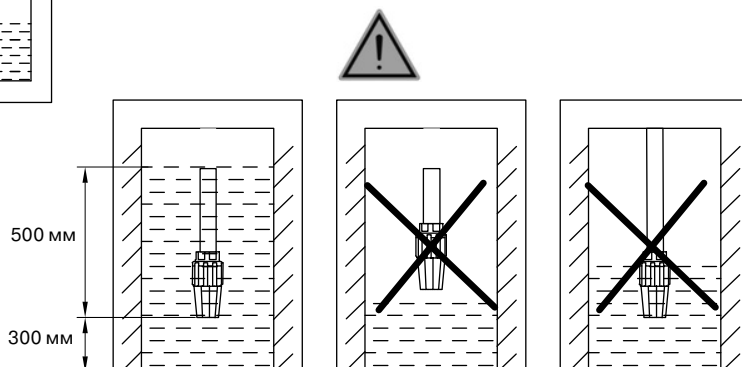
Монтаж обратного клапана и фильтра
