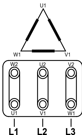
Соединение обмоток «в треугольник» (Δ) (для сети с напряжением 3*230 VAC)
