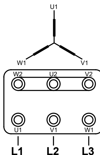
Соединение обмоток «в звезду» (Y) (для сети с напряжением 3*400 VAC)
