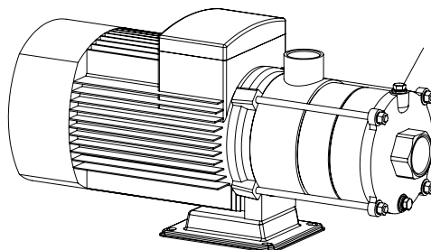
Положение заливного отверстия. 1 – отверстие для заливки
